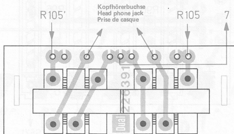
Fig. 24 Übertragerplatte 226 439 (Leiterseite)
