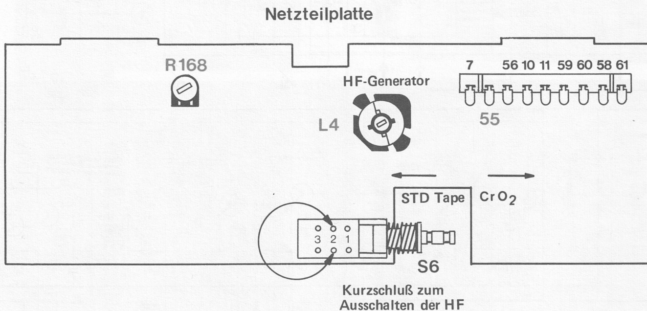
Fig. 17 Abgleichpositionen
