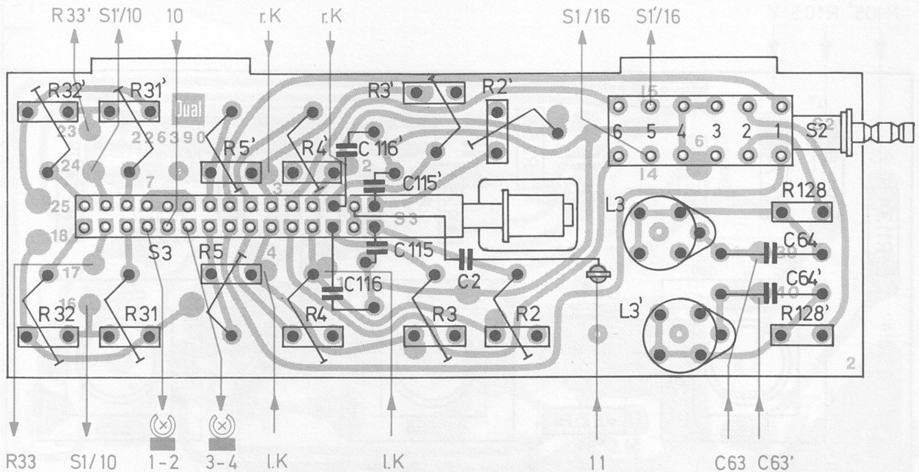
Fig. 23 Netzplatte 226 773 (Leiterseite)
