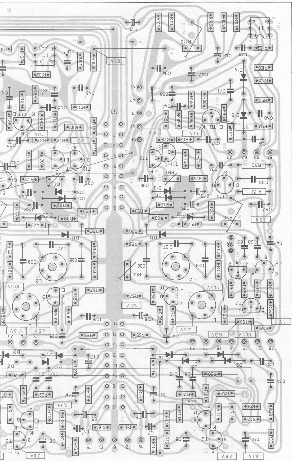
Fig. 20 Verstärkerplatte 226 784 (Bestückungsseite)
