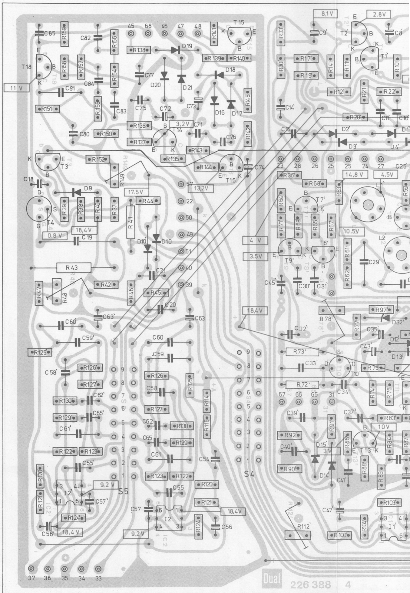
Fig. 21 Verstärkerplatte 226 784 (Leiterseite)
