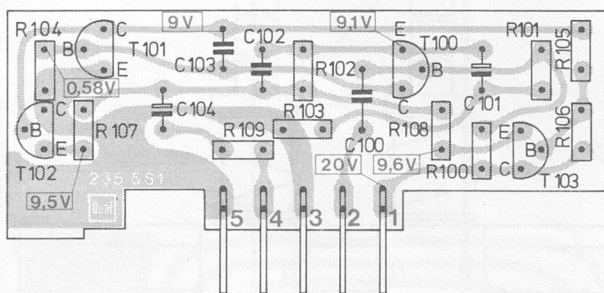
Fig. 29 Ausgangsverstärker 235 494 (Leiterseite)
