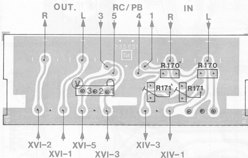
Fig. 30 Buchsenplatte 235 491 (Leiterseite)
