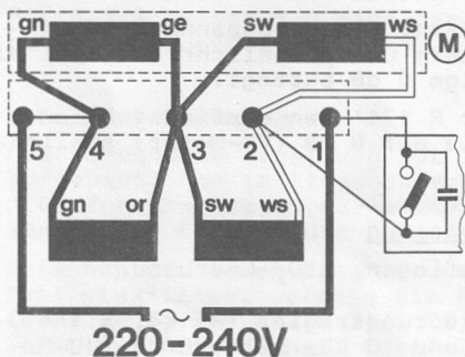
Fig. 18 Spannungsumschaltung
