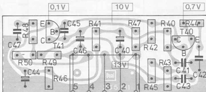
Fig. 24 Wiedergabeverstärker 235 483 (Leiterseite)
