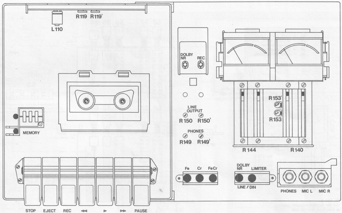
Fig. 19 Abgleichpositionen, Geräteoberseite
