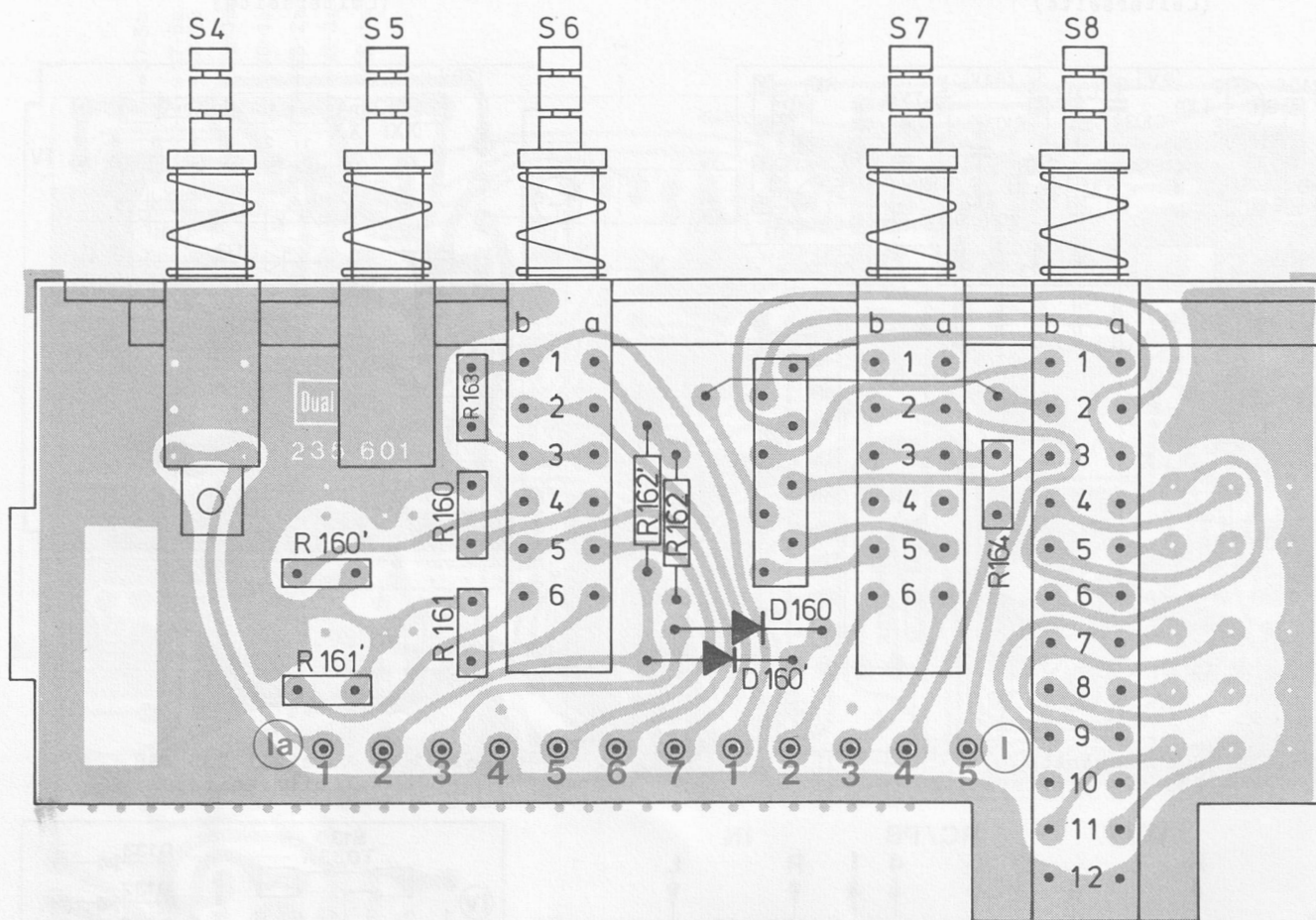
Fig. 33 Tastenplatte 235 489 (Leiterseite)
