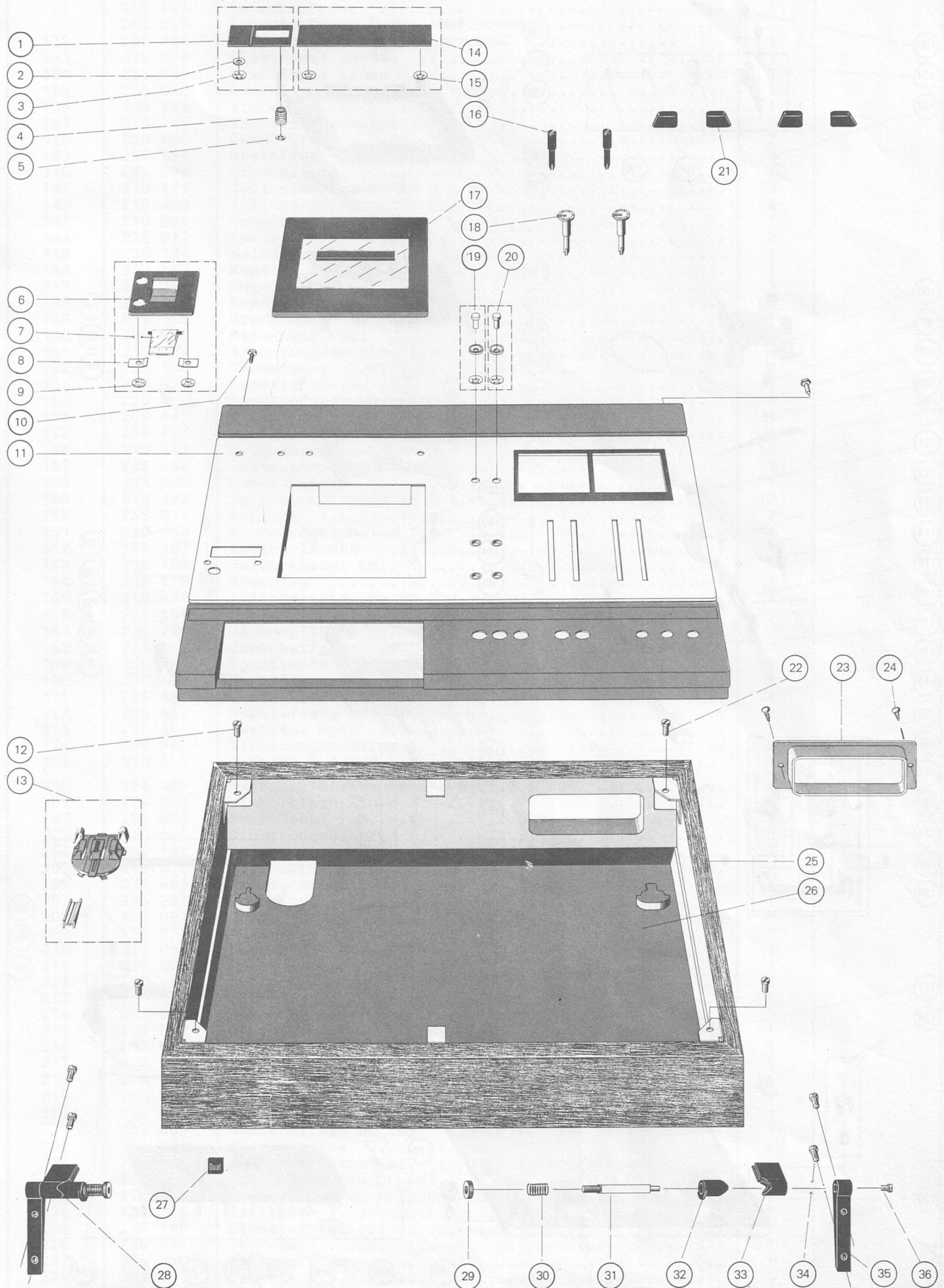
Fig. 36 Explosionsdarstellung I
