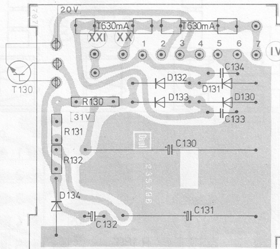
Fig. 31 a Netzteil 241 732 (Leiterseite)
