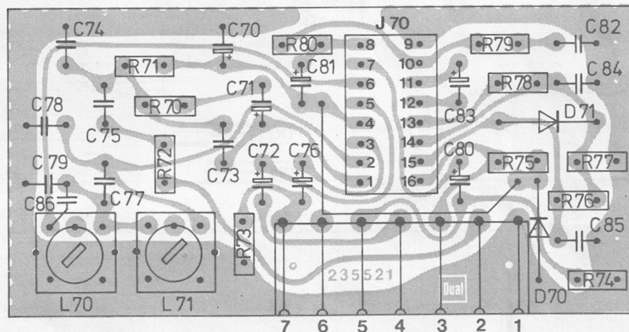
Fig. 23 Dolbyverstärker 235 484 (Leiterseite)
