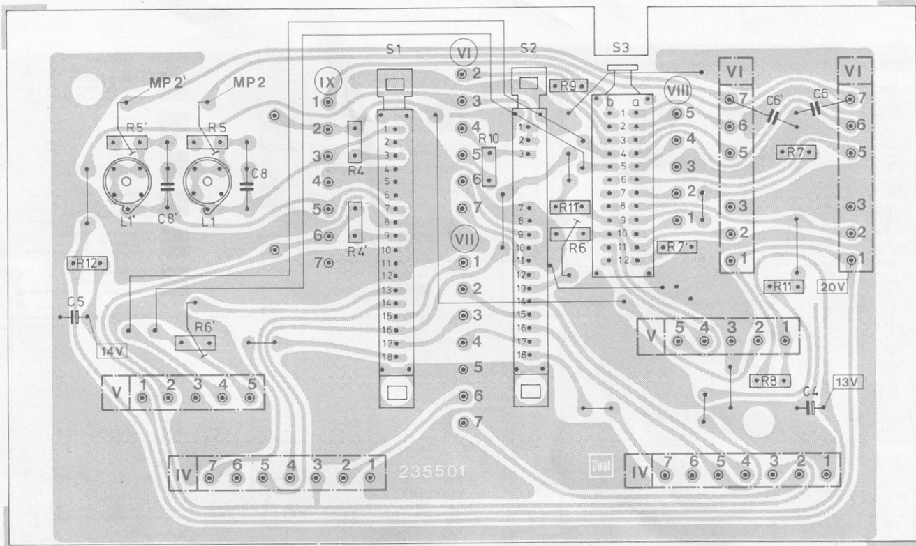
Fig. 22 Grundplatte 235 485 (Leiterseite)
