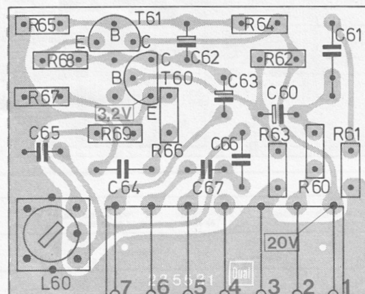
Fig. 25 Aufnahmeverstärker 235 482 (Leiterseite)
