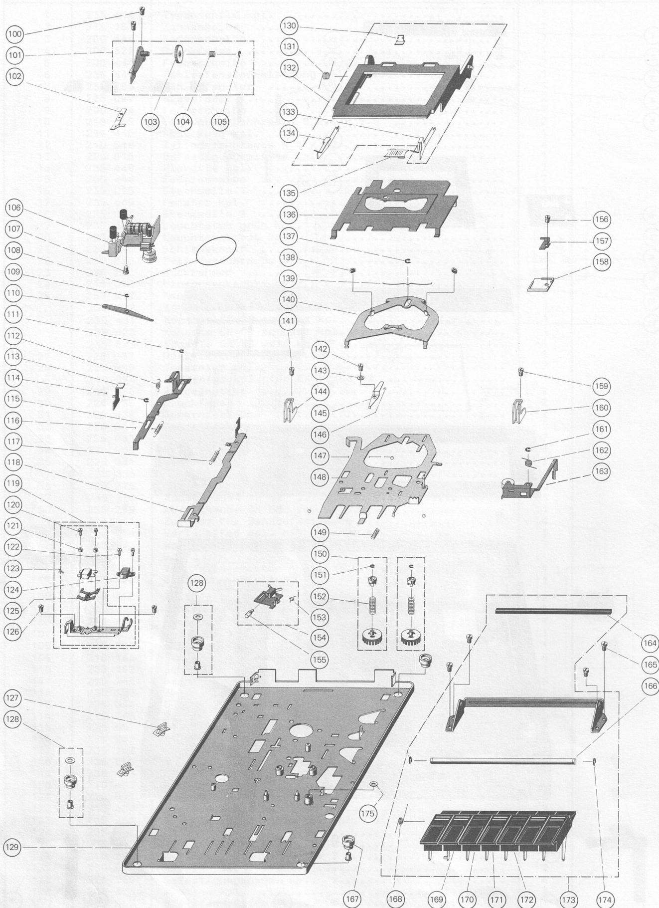
Fig. 37 Explosionsdarstellung II
