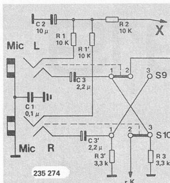
Schaltbuche Mic. links in Arbeitsstellung Switching jack Mic. left in working position Prise de commutation Mic gauche en fonction
