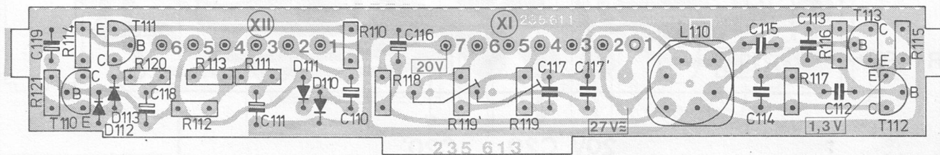
Fig. 32 Generatorplatte 235 481 (Leiterseite)
