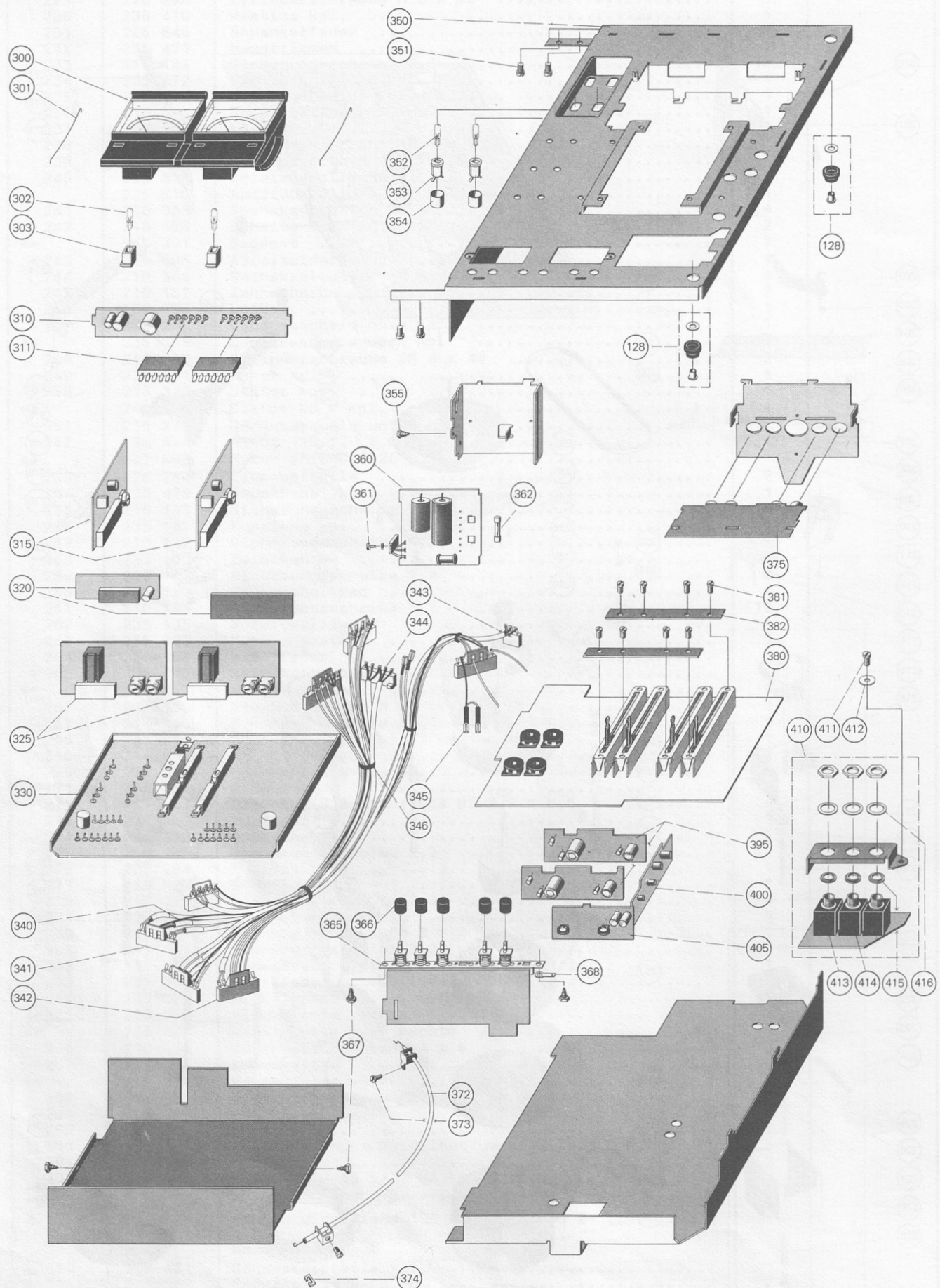
Fig. 39 Explosionsdarstellung IV
