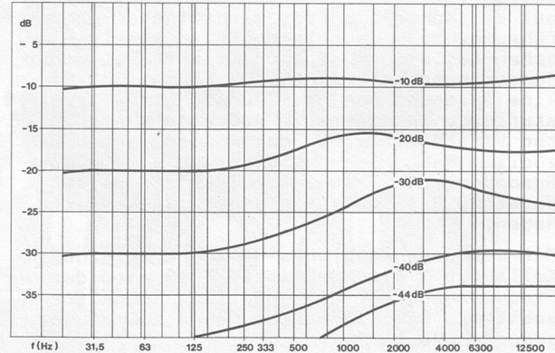
Fig. 16 Dolby-Frequenzverlauf
