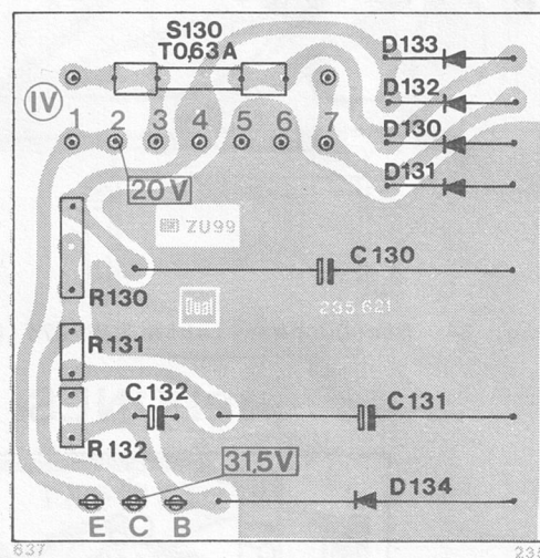
Fig. 31 b Netzteil 235 488 (Leiterseite)
