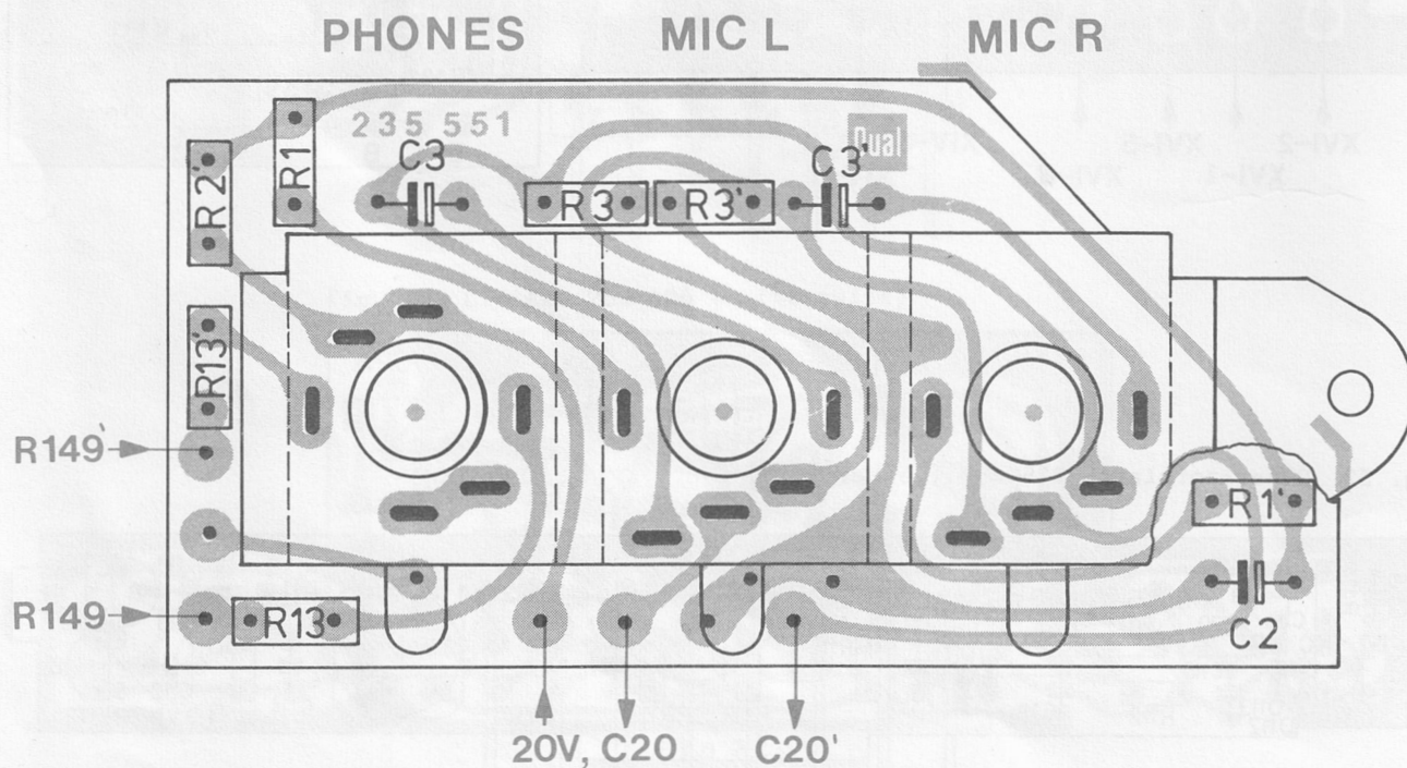
Fig. 34 Mic-Buchsenplatte 235 274 (Leiterseite)
