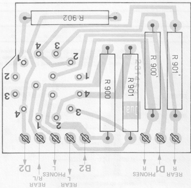
Fig. 4 Betriebserschalter 233 975 (Leitersseite)
