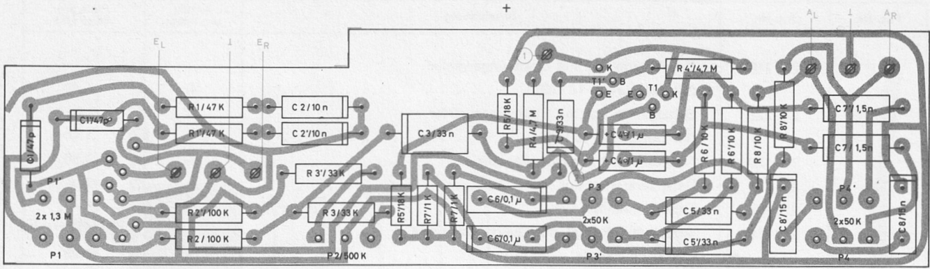
Fig. 4 Ätzschnitplatte Regelverstärker (Bestückungsseite)
