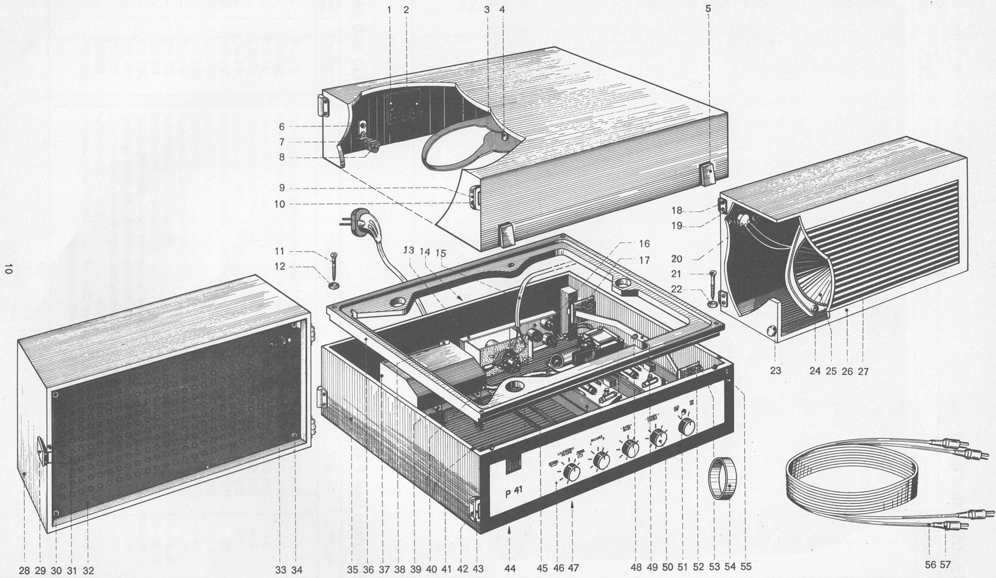
Fig. 7 Koffer, Bedienungselemente und Beschlagteile Stereo-Verstärkerkoffer Dual P 41
