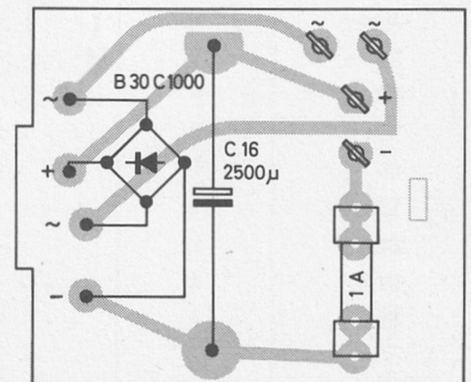
Fig. 2 Ätzschtaltplatte für Netzteil, 213 869
