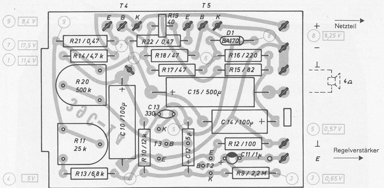
Fig. 5 Ätzzschaltplatte Endstufeneinheit (Bestückungsseite)
