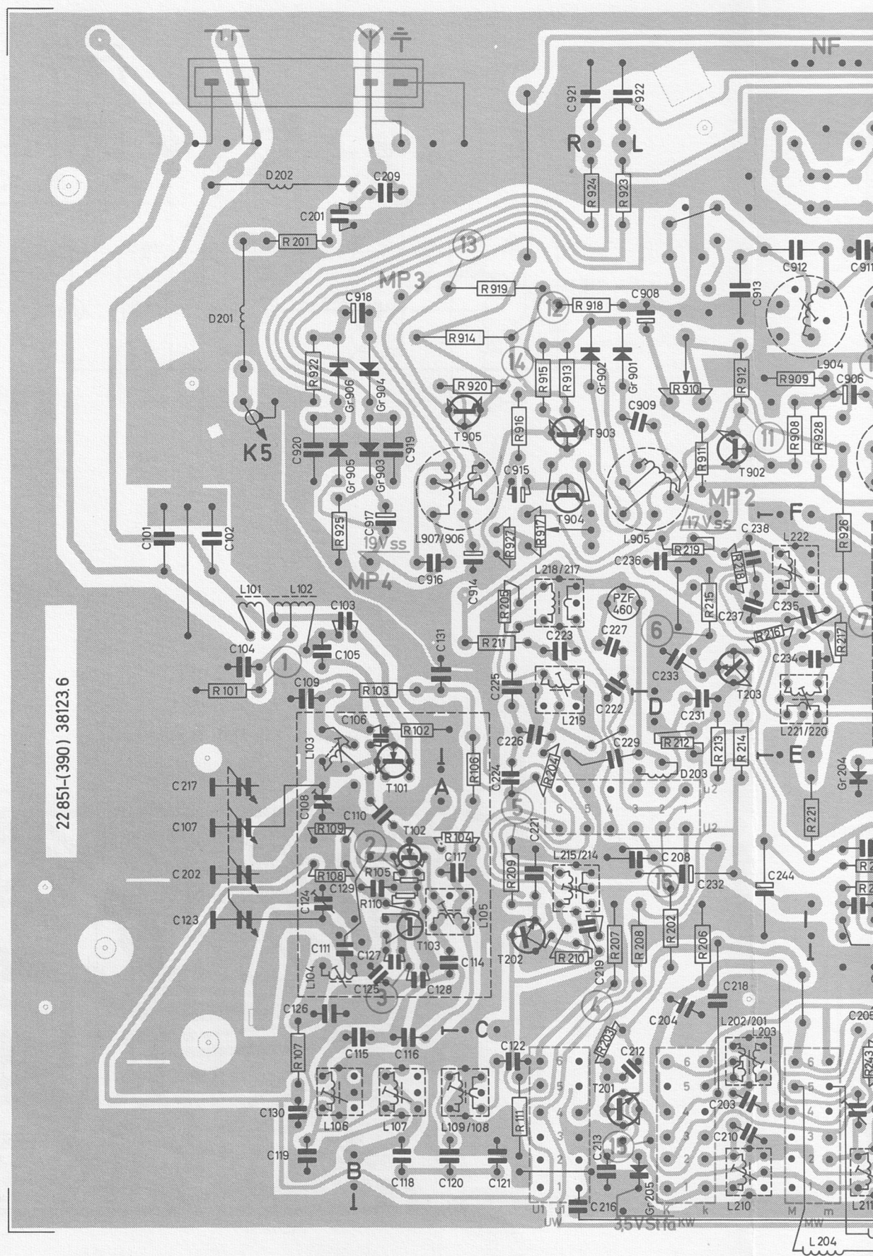
FM ① + 1 V ② + 1,4 V ③ + 1,4 V ④ + 1,8 V ⑤ + 1,1 V ⑥ + 1,9 V ⑦ + 1,1 V ⑧ + 10 V ⑨ + 2,3 V ⑩ + 8 V ⑪ + 9 V ⑫ + 0,7 V ⑬ + 4,9 V m.Pilot ⑭ + 23 V + 5 V AM ⑮ + 3,5 V ⑯ + 15 V ⑰ + 1,5 V
