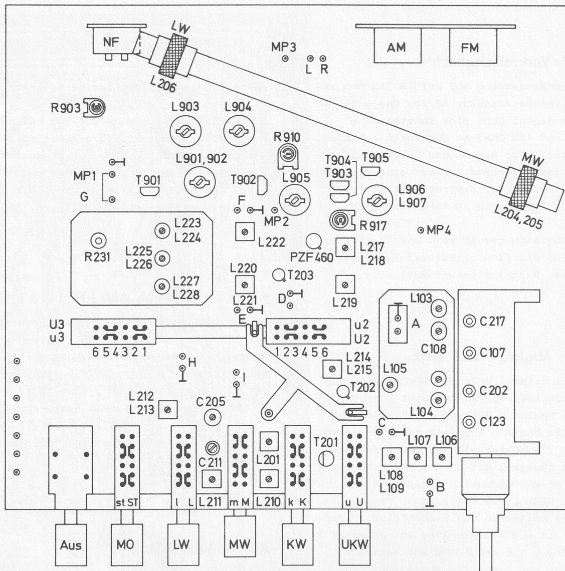
Fig. 11 Abgleichpunkte
