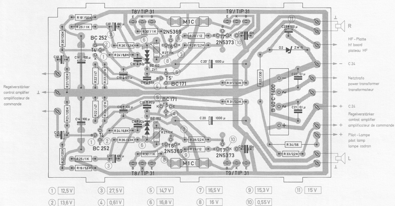
Fig. 9 Ätzsaltplatte des Endverstärkers 220 521 (Leiterseite)
