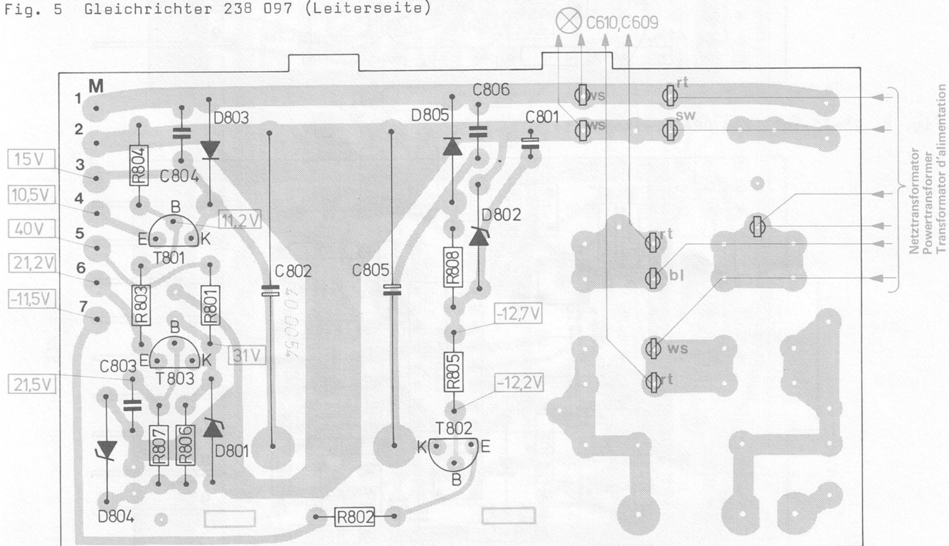
Fig. 5 Gleichrichter 238 097 (Leiterseite)
