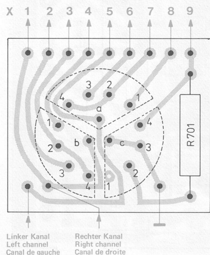
Fig. 14 Betriebsartenschalterplatte 234 473 (Leiterseite)
