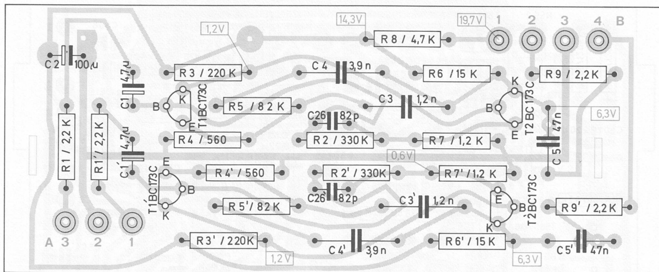
Fig. 13 Lautsprecheranschlußplatte 234 475 (Leiterseite)
