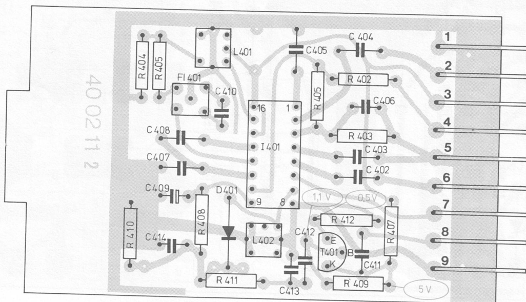
Fig. 8 AM-ZF-Teil 238 098 (Leiterseite)
