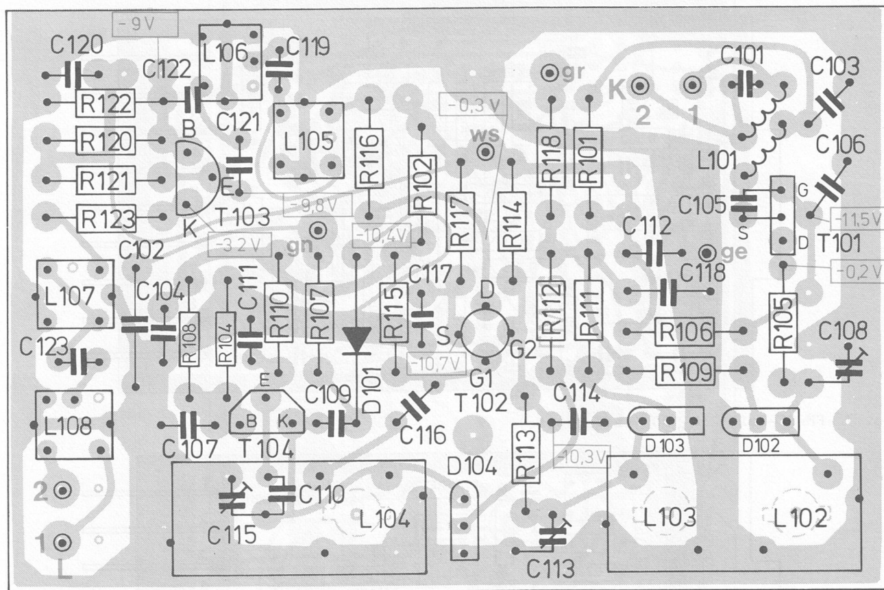
Fig. 4 UKW-Teil 238 096 (Leiterseite)
