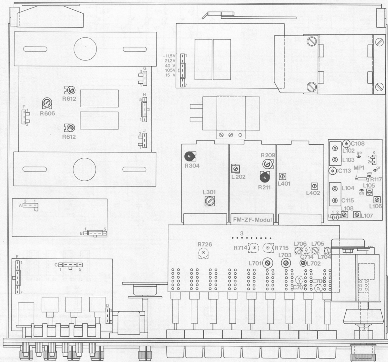
Fig. 1 Abgleichpositionen
