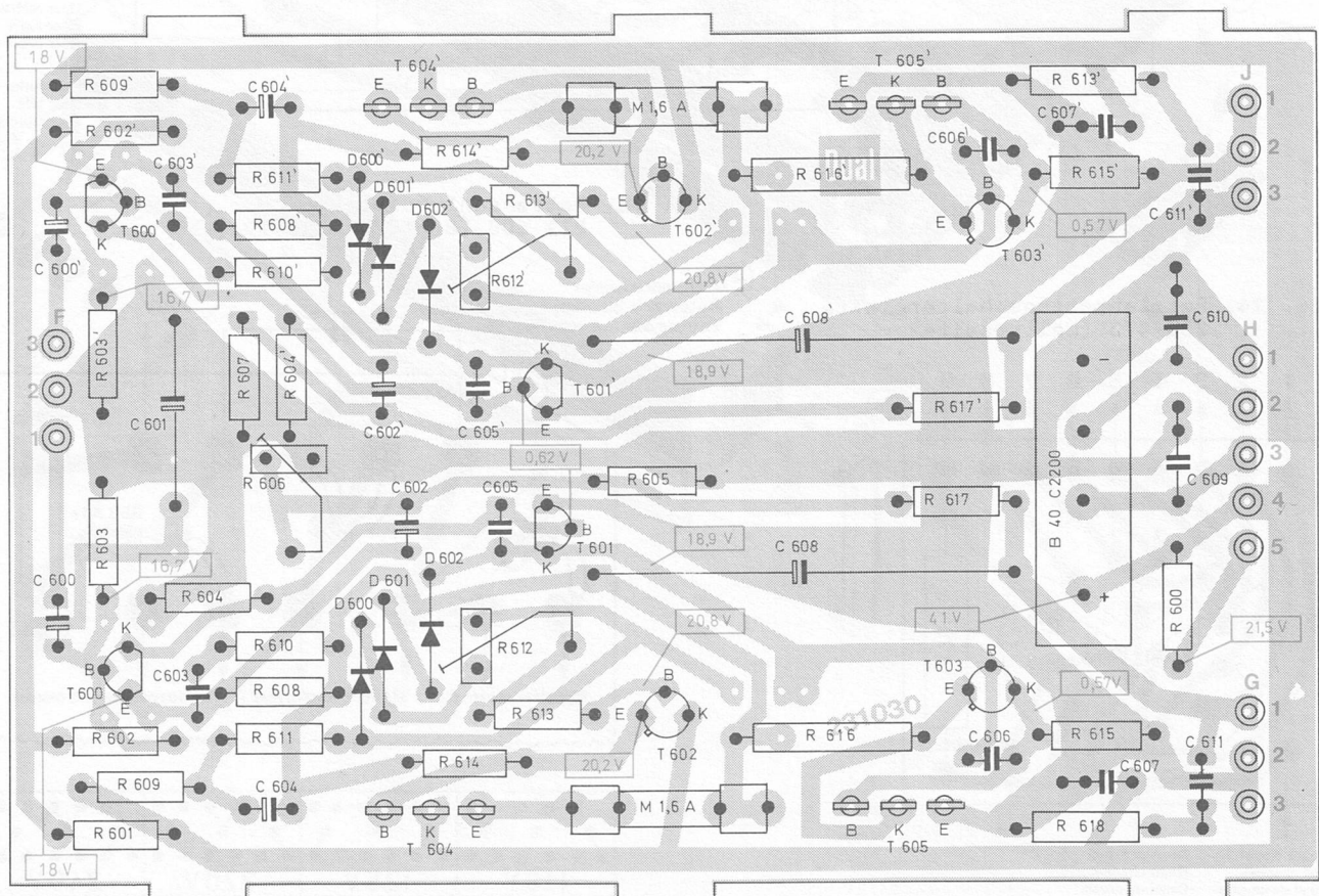
Fig. 11 Endverstärker 234 147 (Leiterseite)
