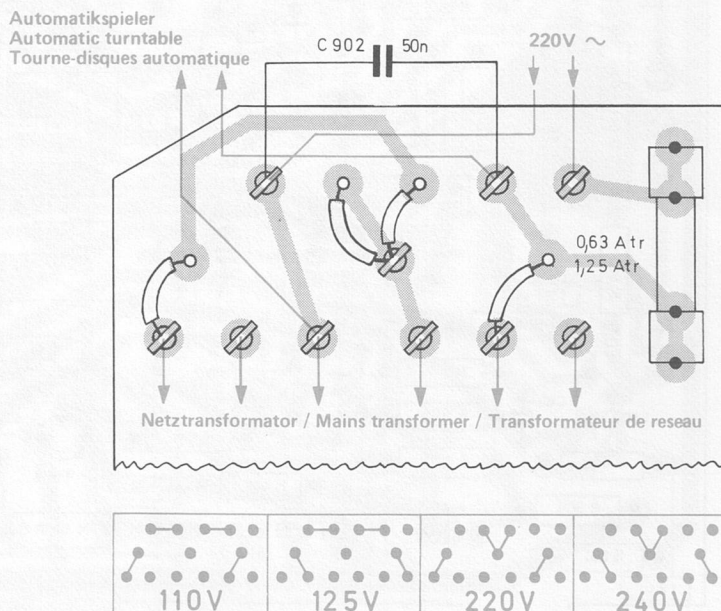
Fig. 15 Netzanschlußplatte 212 600 (Bestückungsseite)
