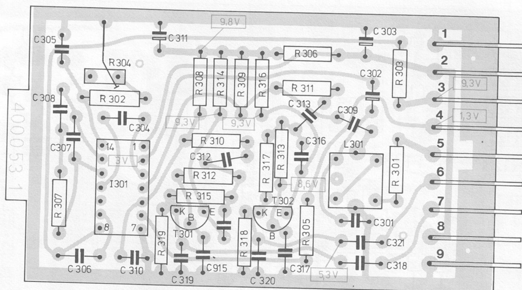
Fig. 7 FM-ZF-Teil 238 100 (Leiterseite)
