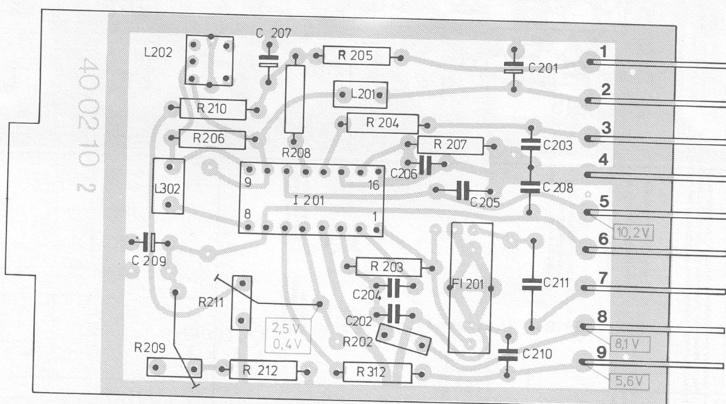
Fig. 8 AM-ZF-Teil 238 098 (Leiterseite)
