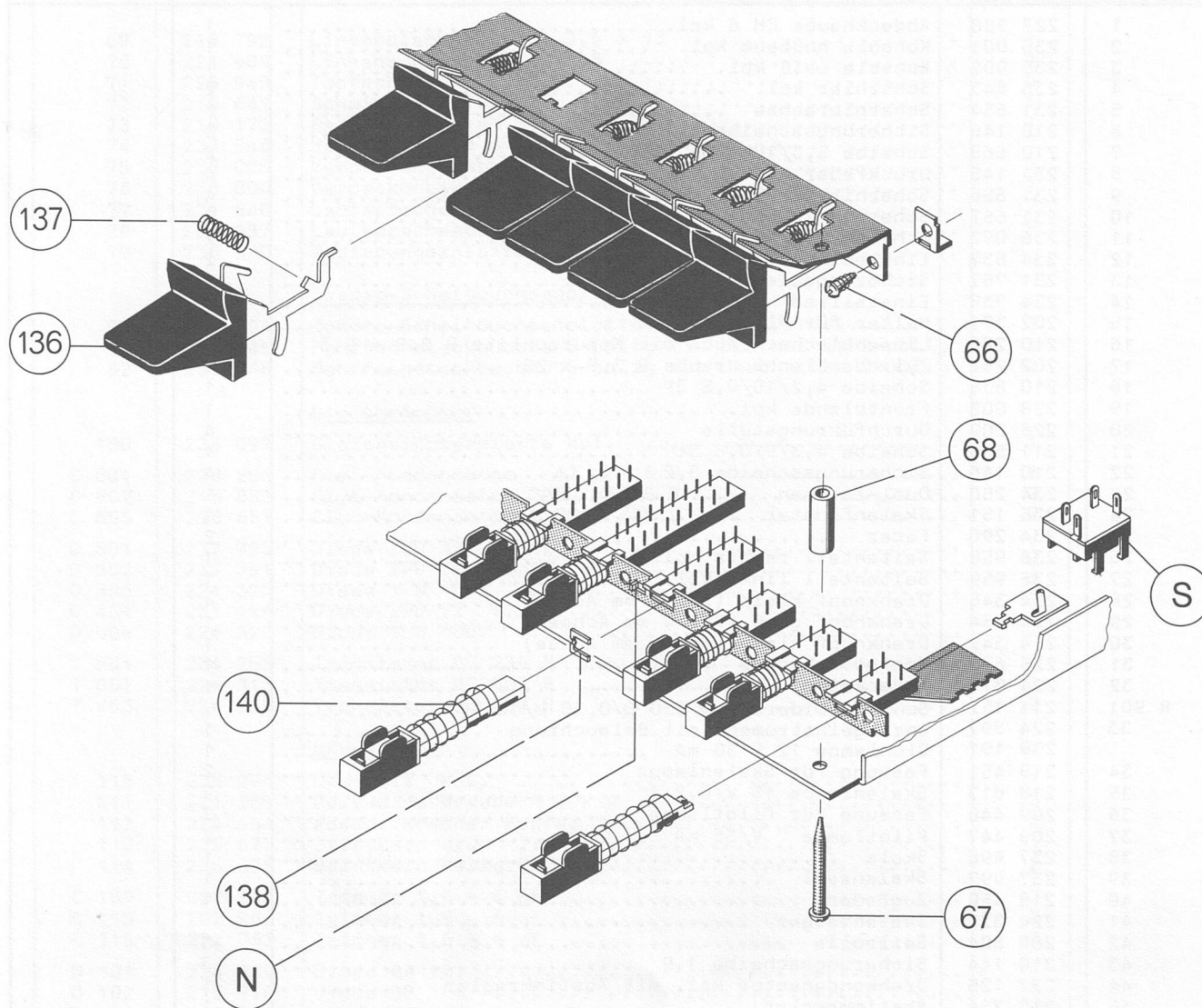
Fig. 17 Auswechseln der Tastenschieber
