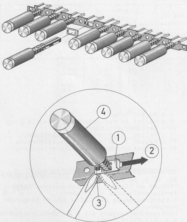
Fig. 9 Auswechseln der Schieber
