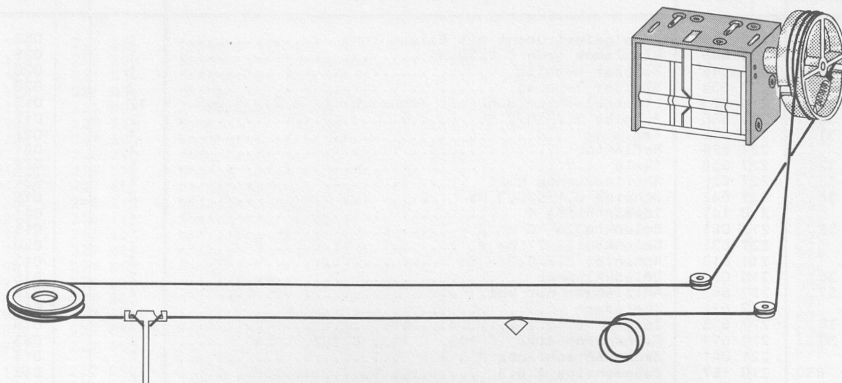
Fig. 8 Seilschema
