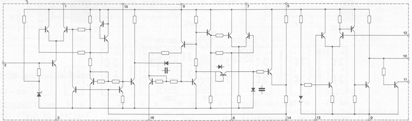
Fig. 3 Prinzipschaltbild TBA 570
