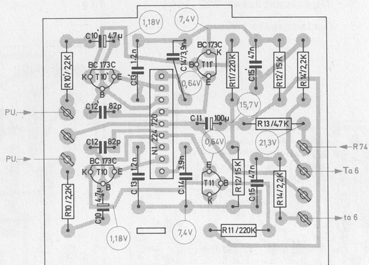
Fig. 4 Vorverstärker 227 585 (Leiterseite)
