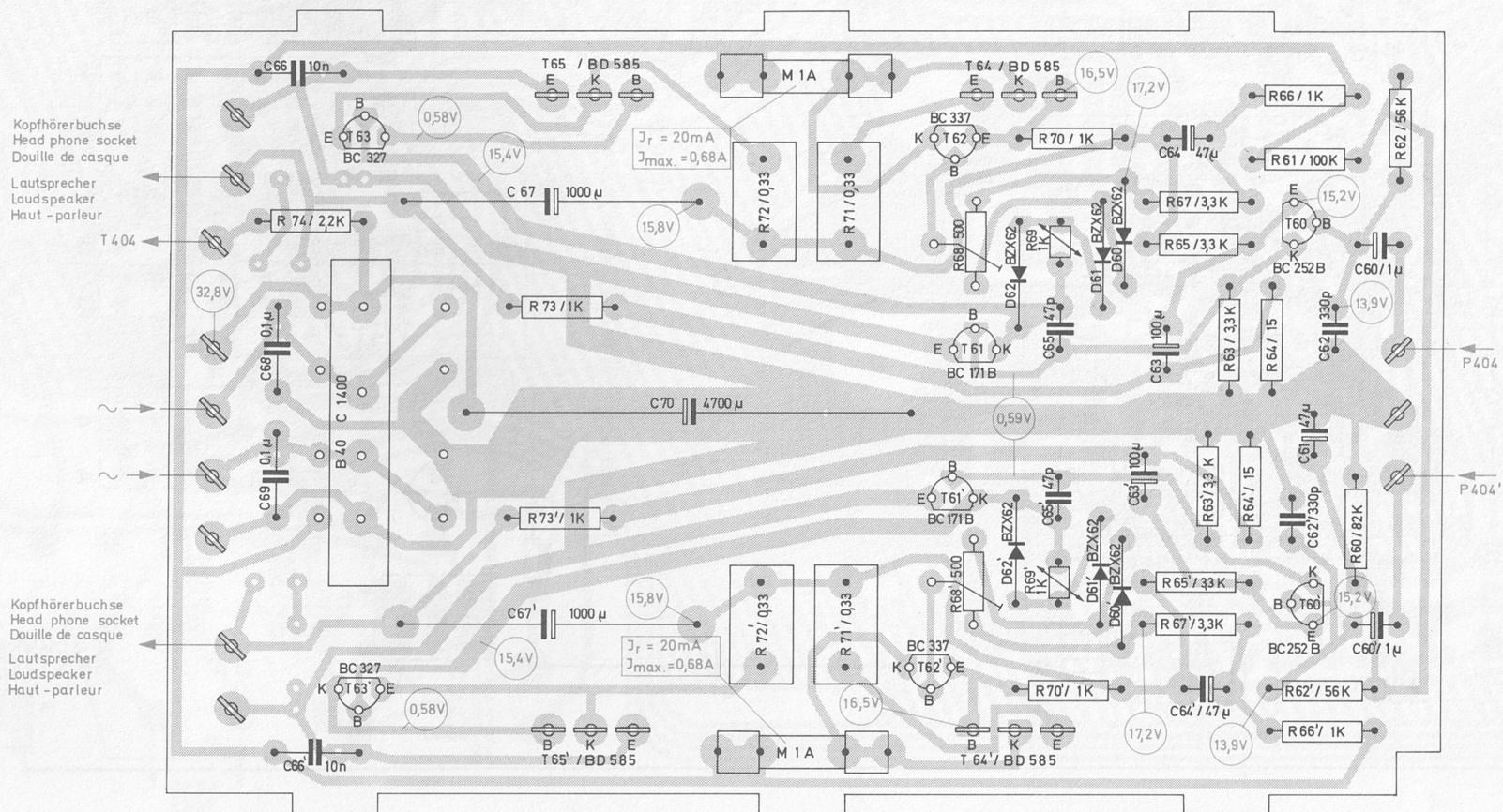
Endverstärker 227 587 (Leiterseite)
