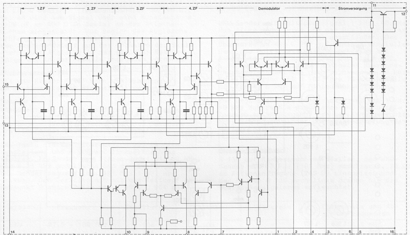
Fig. 3 Prinzipschaltbild TBA 570
