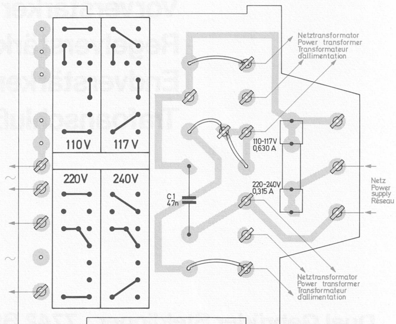
Anschlußplatte 225 535 (Bestückungsseite)
