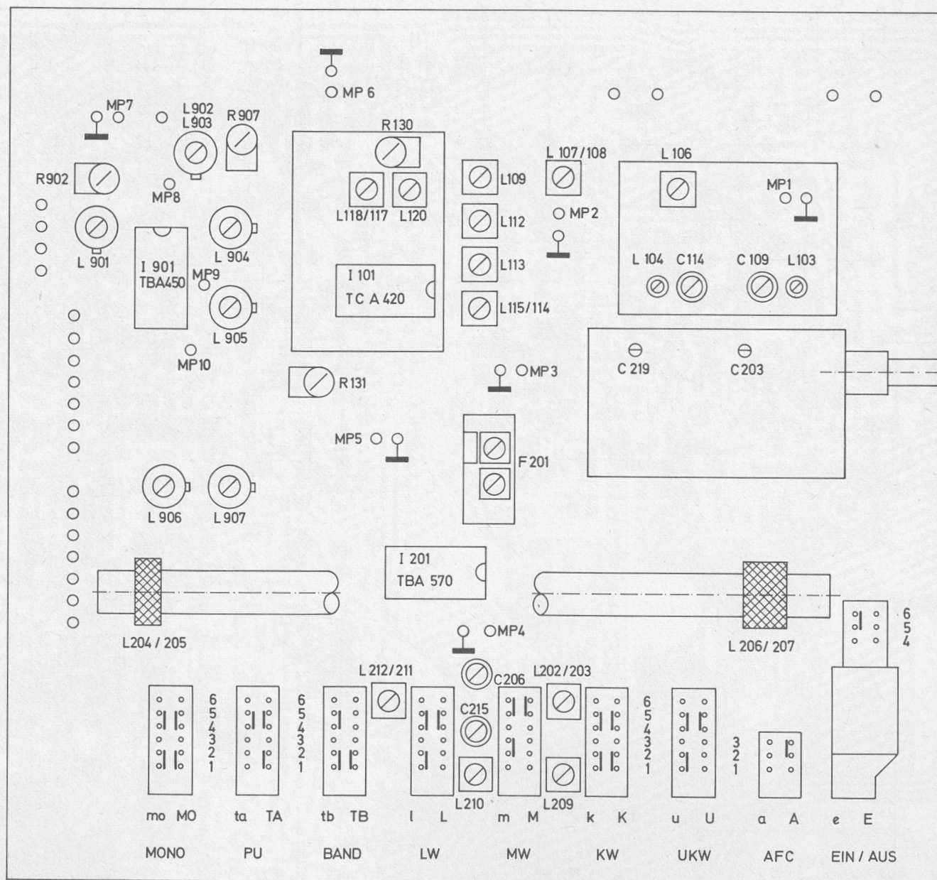
Fig. 8 Abgleichpositionen
