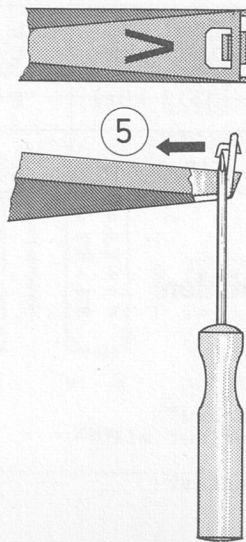
Fig. 7 Demontage Reflektor
