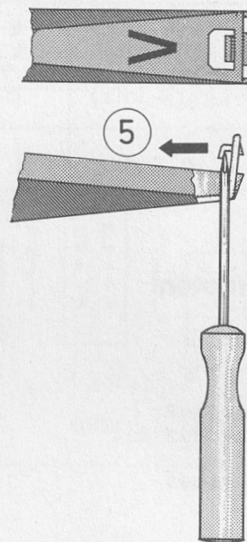
Fig. 10 Demontage des Reflektors
