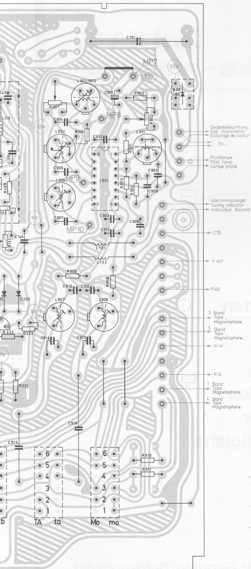
Vorverstärker 227 585 (Leiterseite)
