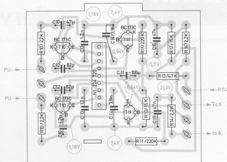
Vorverstärker 227 585 (Leiterseite)
