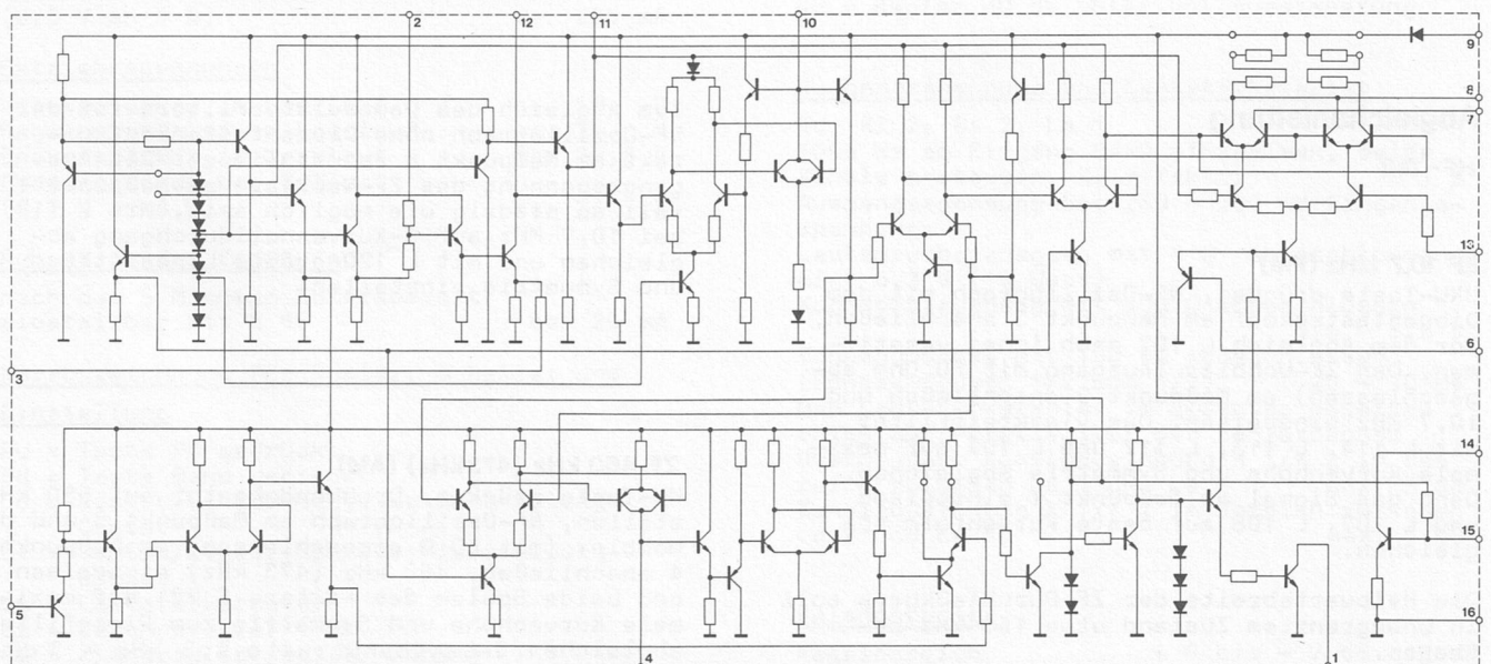
Fig. 4 Prinzipschaltbild TBA 450
