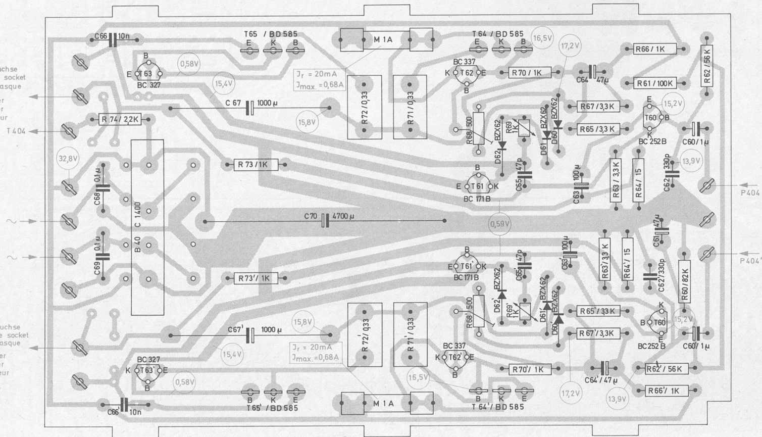
Fig. 7 Endverstärker 227 587 (Leitersseite)
