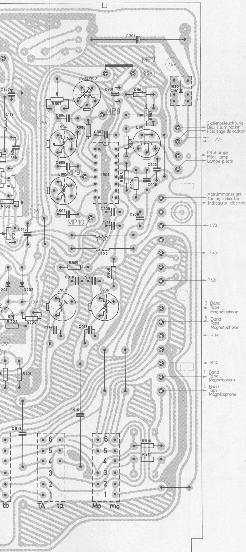
Fig. 4 Vorverstärker 227 585 (Leiterseite)
