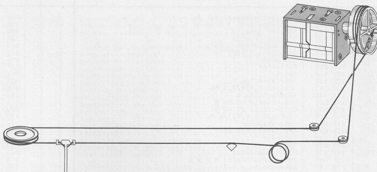
Fig. 11 Seilschema
