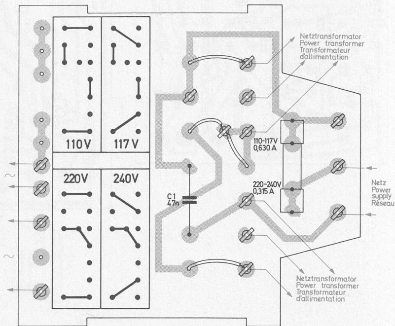
Fig. 5 Anschlußplatte 225 535 (Bestückungsseite)
