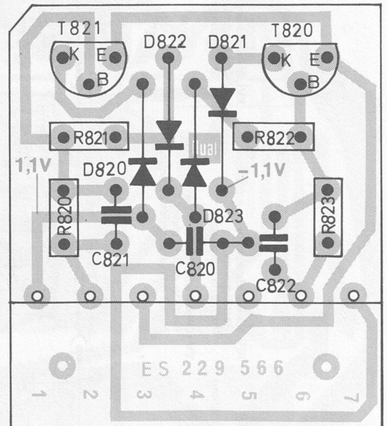
Fig. 41 Elektronische Sicherung IX 232 451 Leiterseite
