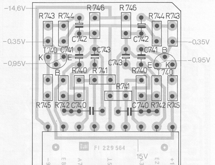
Fig. 43 Filter XI 233 053 Leiterseite
