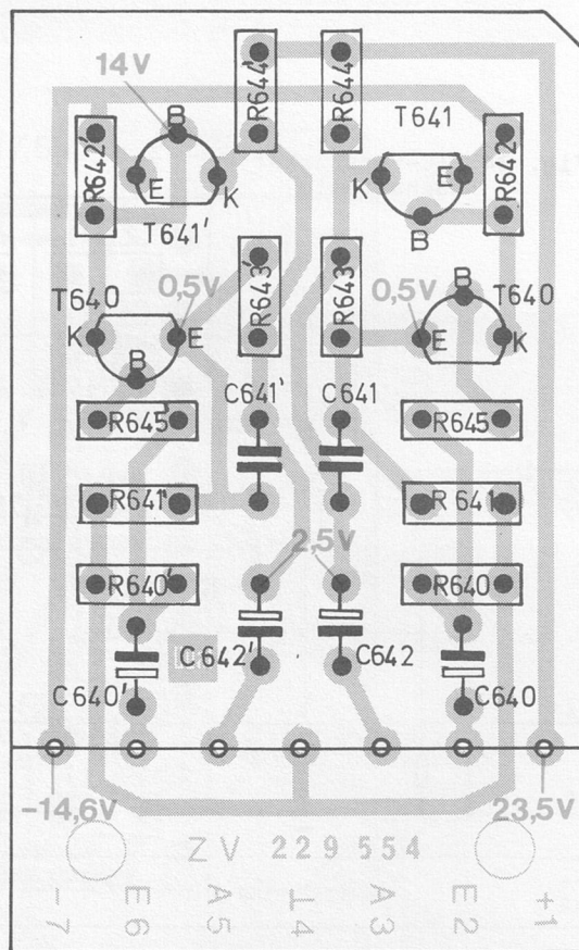
Fig. 39 Zwischenverstärker VII 232 460 Leiterseite
