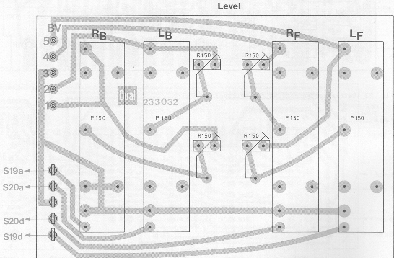
Fig. 24 Pegelregler 236 864 Leiterseite
