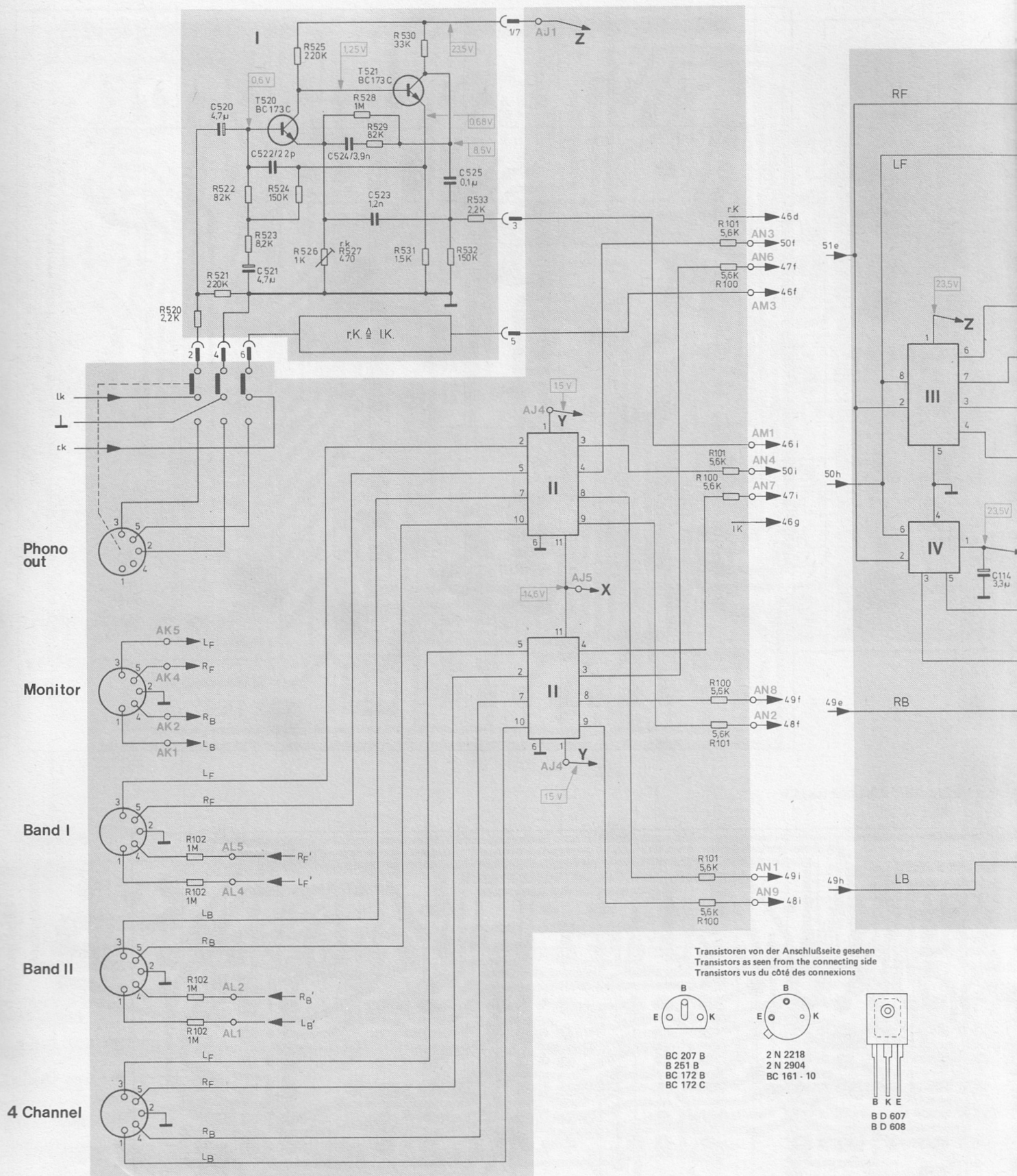
Fig. 11 NF-Teil, Schaltbild
