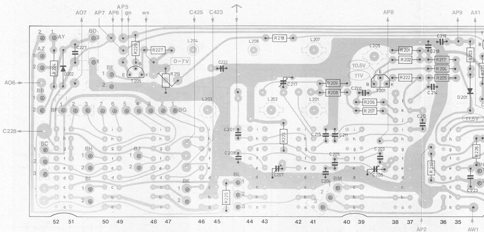
Fig. 12 AM-HF-Teil 236 874 Leiterseite
