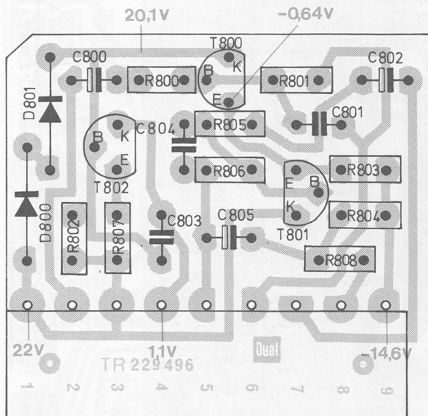
Fig. 40 Universalaltreiber VIII 232 452 Leiterseite
