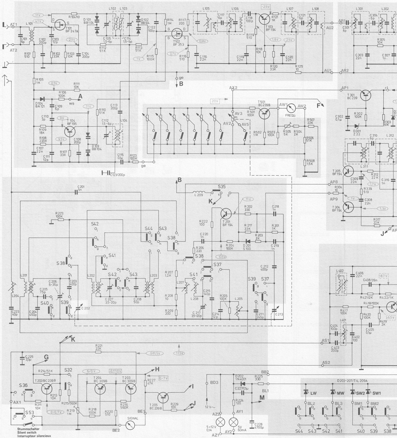
Fig. 10 HF-Teil, Schaltbild
