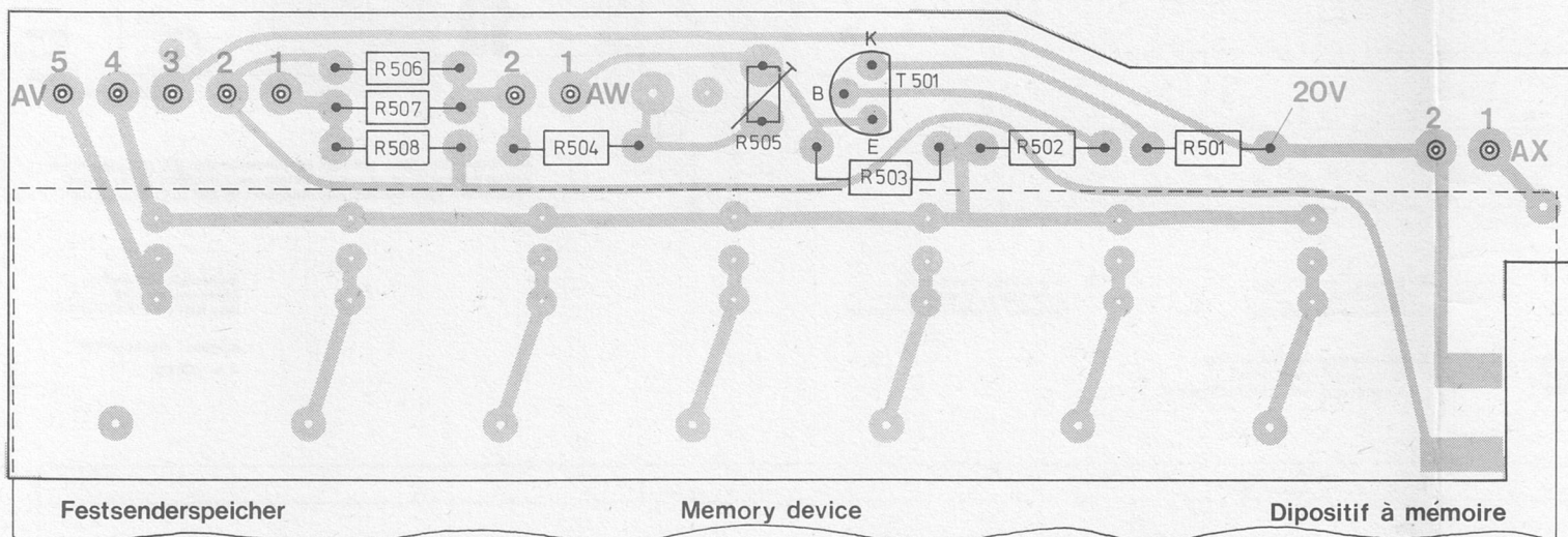
Fig. 14 Festsenderspeicher 236 873 Leiterseite
