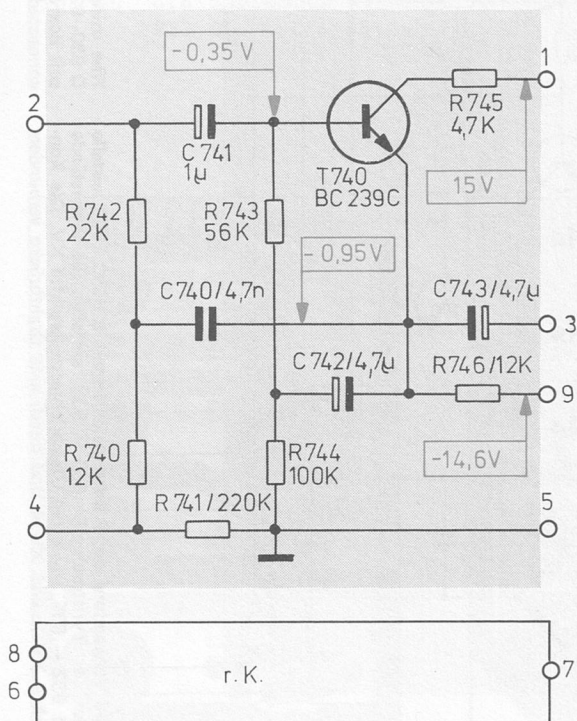
Fig. 42 Filter XI Schaltbild
