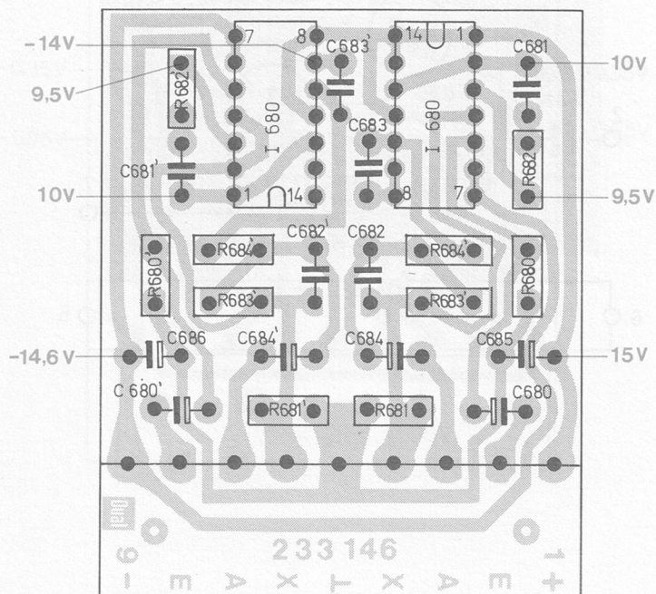
Fig. 35 IC-Verstärker V 232 459 (Leiterseite)
