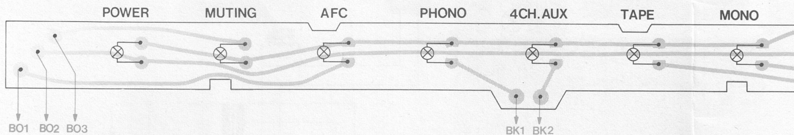
Fig. 13 Tastenanzeigeplatte 236 880 Leiterseite
