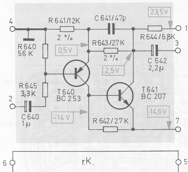
Fig. 38 Zwischenverstärker VII Schaltbild
