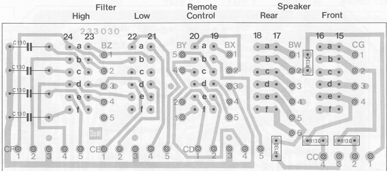
Fig. 23 Schalterplatte 236 866 Leiterseite
