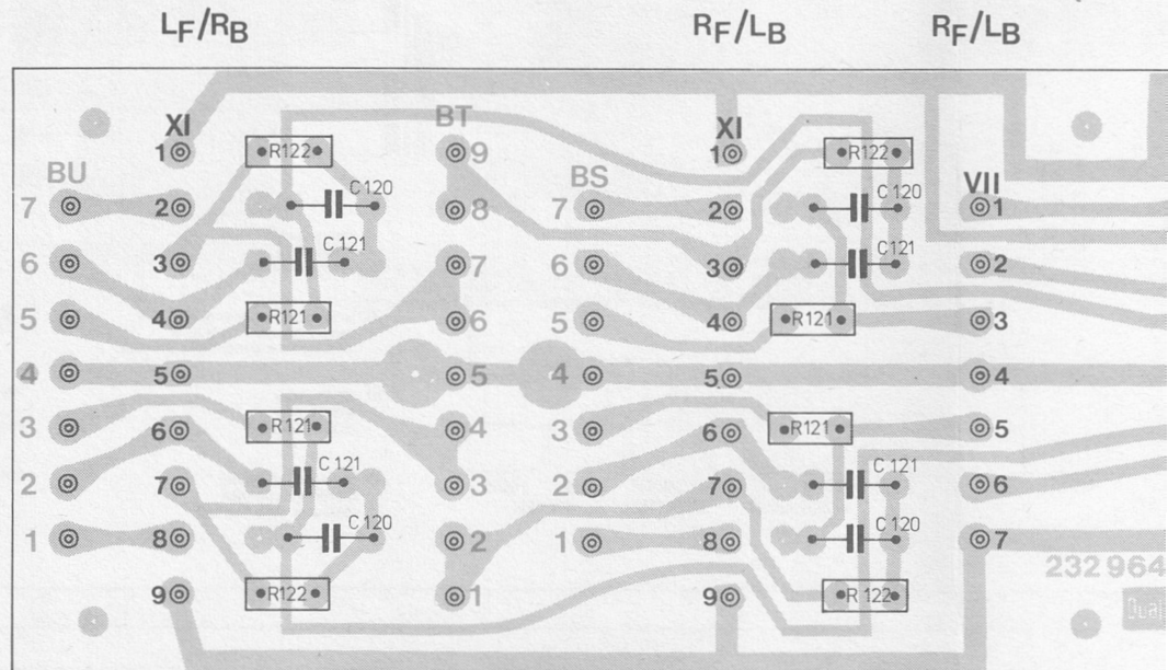
Fig. 17 Steuerverstärker 236 861 Leiterseite
