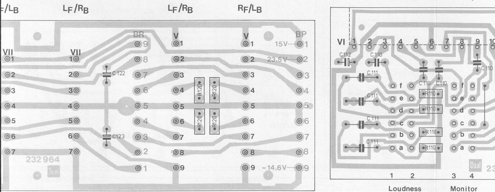
Fig. 19 Betriebsartenschalter 236 858
