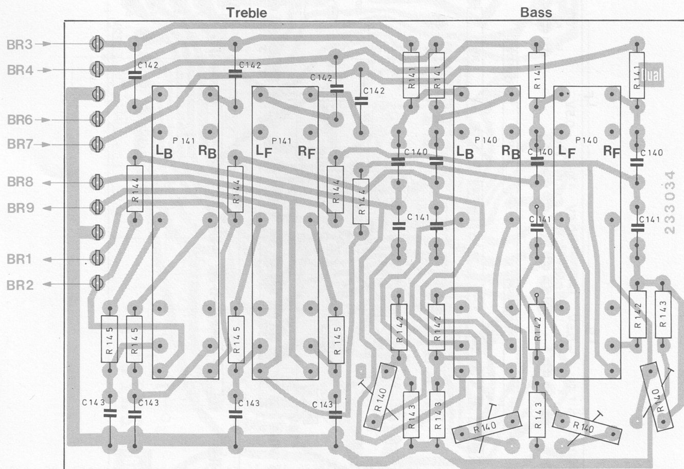
Fig. 25 Klangregler 236 865 Leiterseite
