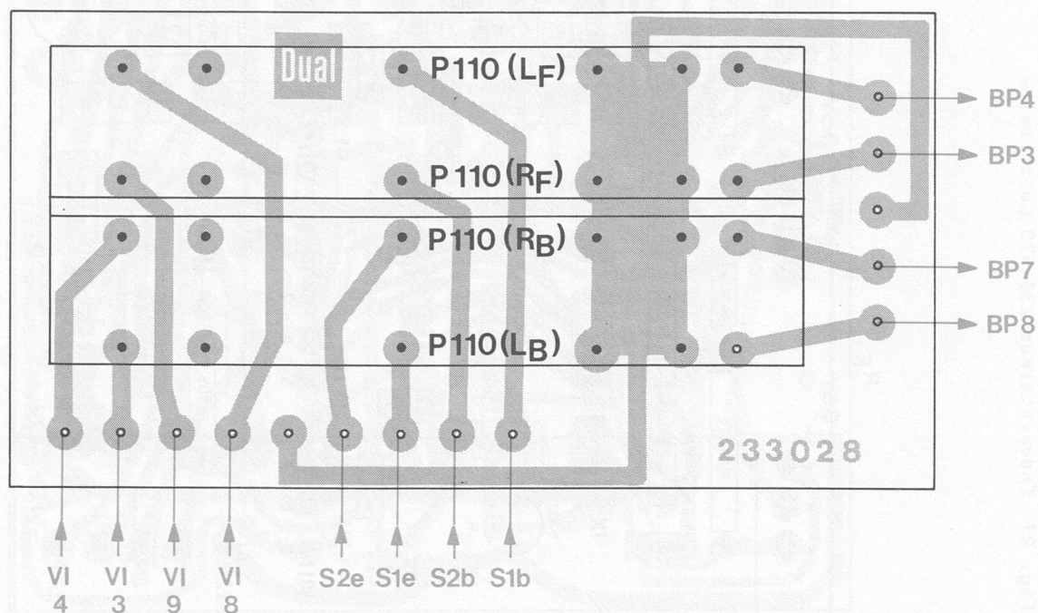
Fig. 26 Lautstärkeregler 236 859 Leiterseite
