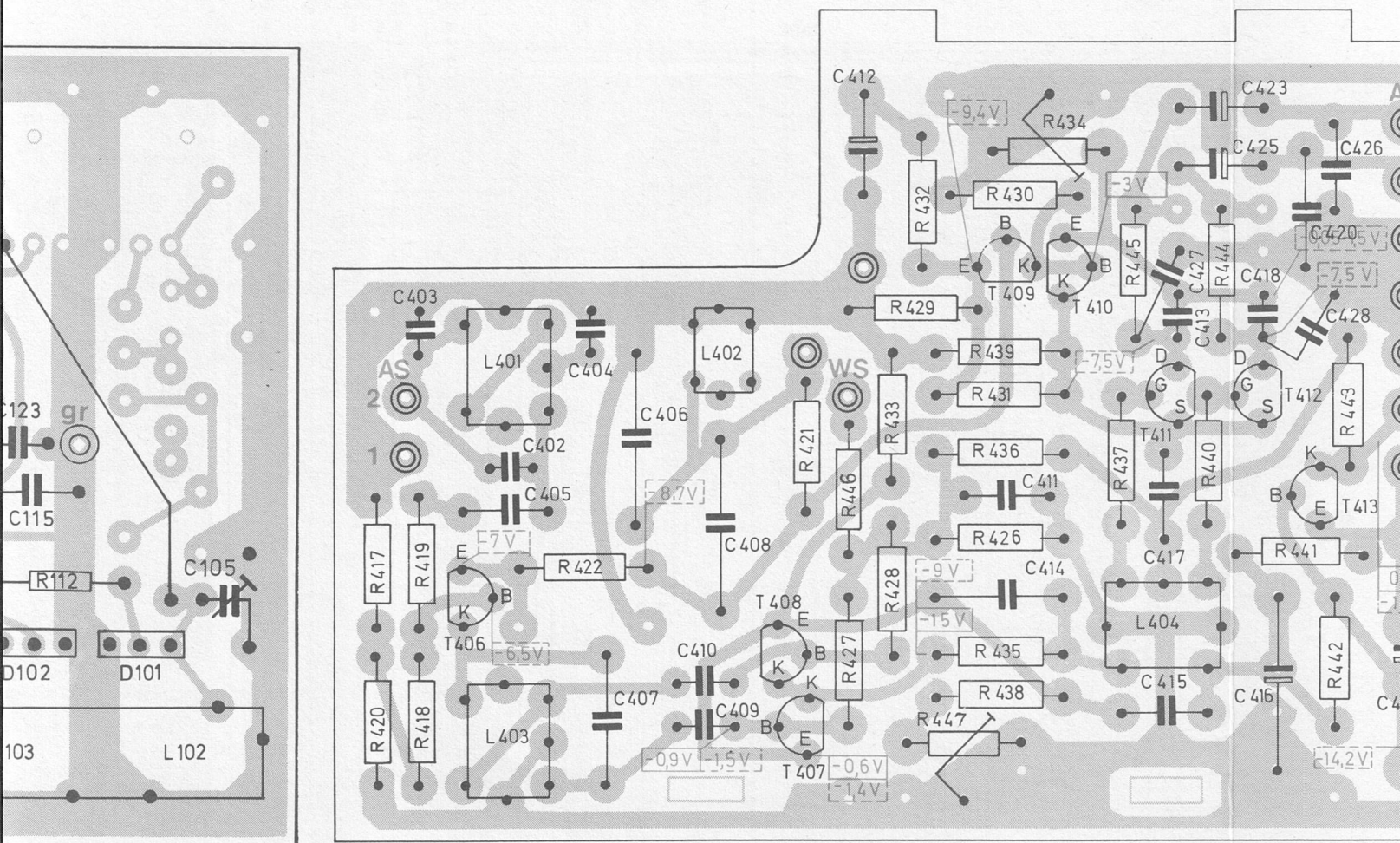
Fig. 18 Stereo-Decoder 236 882 Leiterseite
