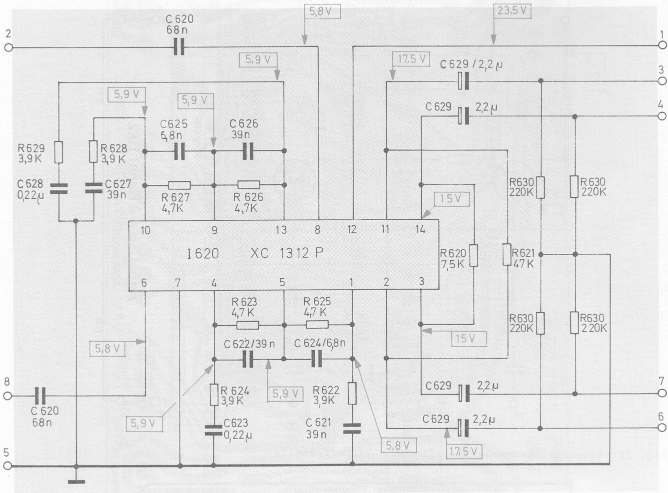
Fig. 31 SQ-Decoder III 232 461 (Leiterseite)
