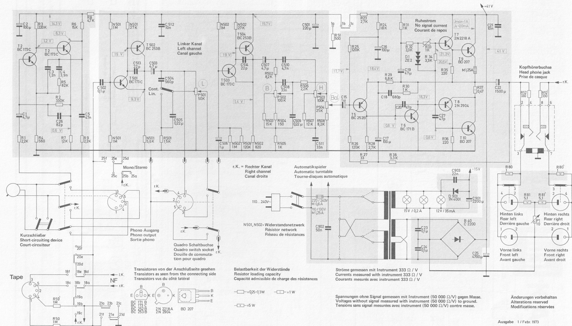
Fig. 2 Schaltbild NF
