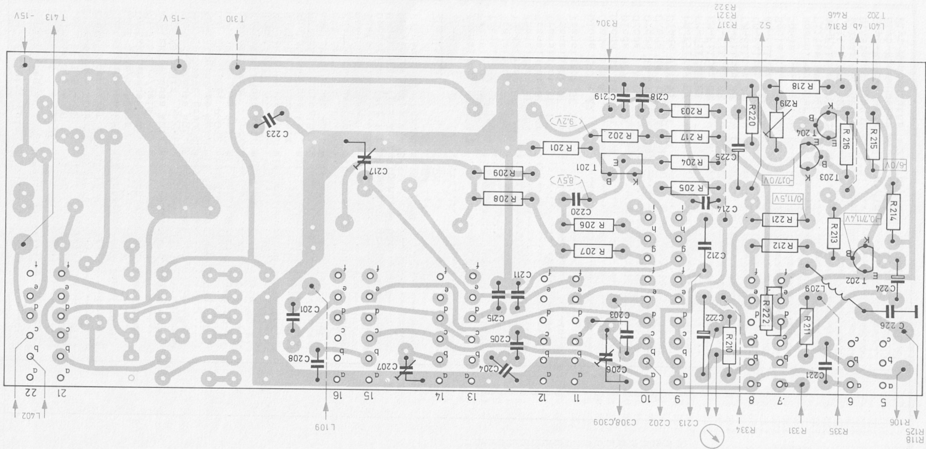
Fig. 12 AM-HF-Platte 231 206 (Leiterseite)
