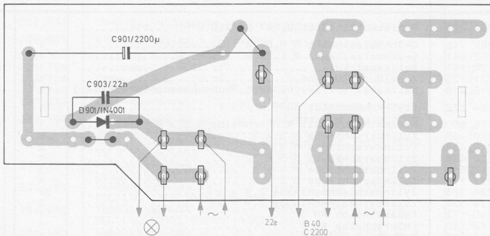
Fig. 13 Gleichrichter-Platte 231 217 (Bestückungsseite)
