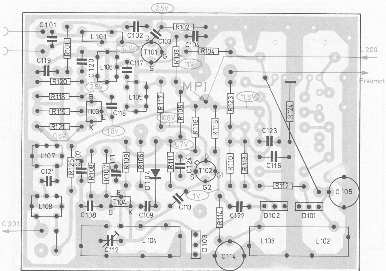
Fig. 10 UKW-Teil 231 211 (Leiterseite)
