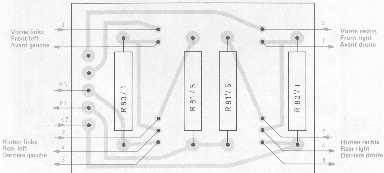
Fig. 7 Widerstands-Platte 231 212 (Bestückungsseite)
