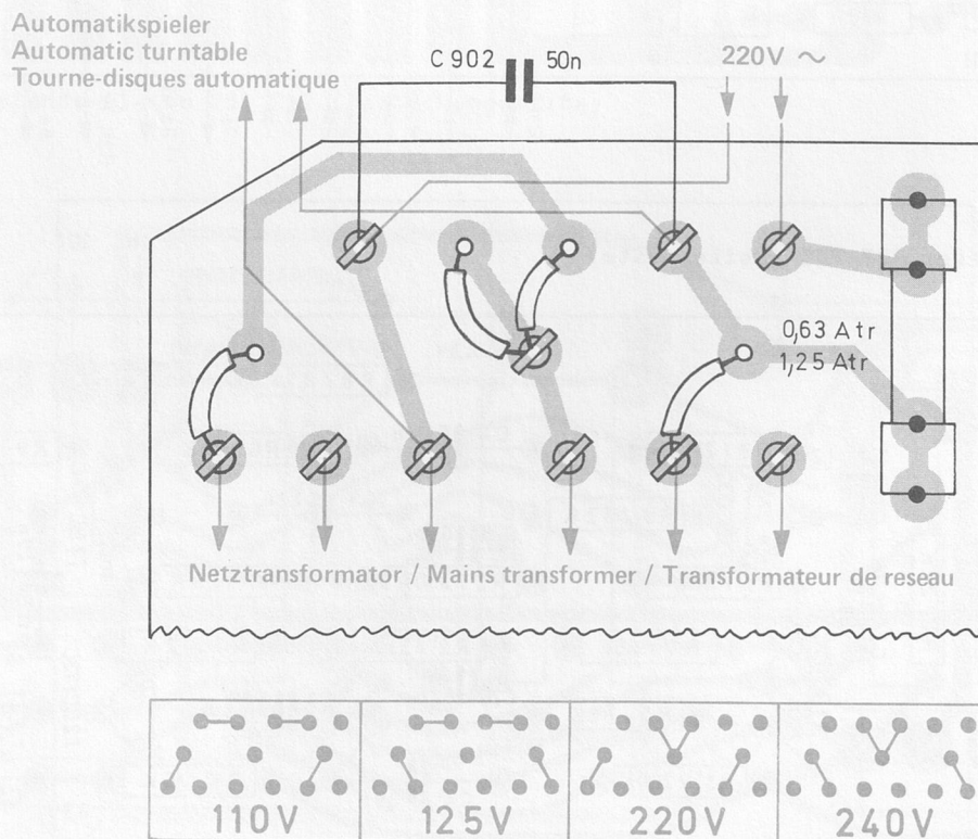
Fig. 11 Netzanschluß-Platte 212 600 (Bestückungsseite)
