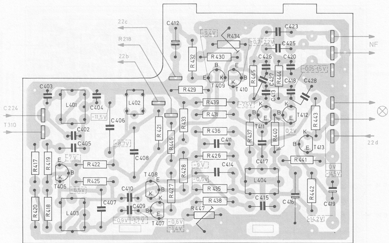
Fig. 6 Decoder 231 209 (Leiterseite)
