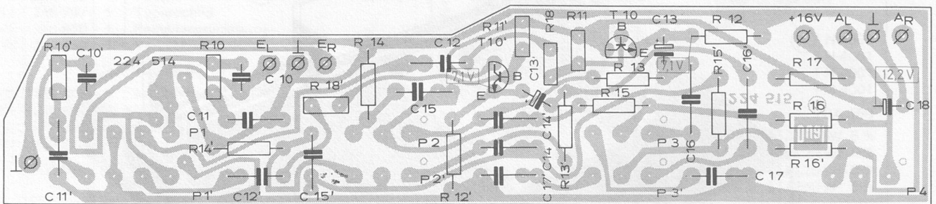
Fig. 5 Regelverstärker 225 474 Bestückungsseite
