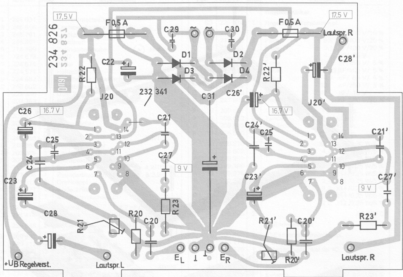
Fig. 4 Endverstärker 236 957 Bestückungsseite
