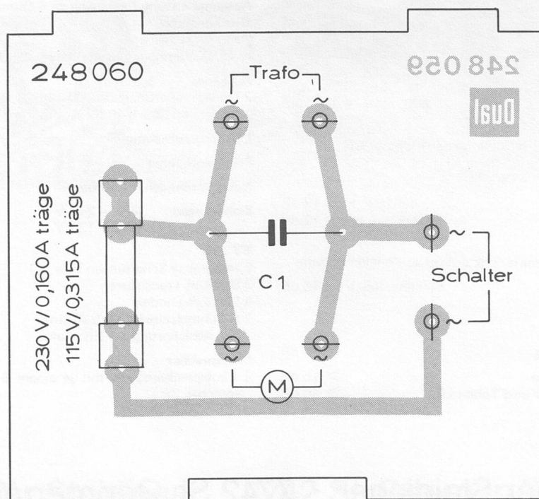
Fig. 1 Netzplatte 248 060 Bestückungsseite
