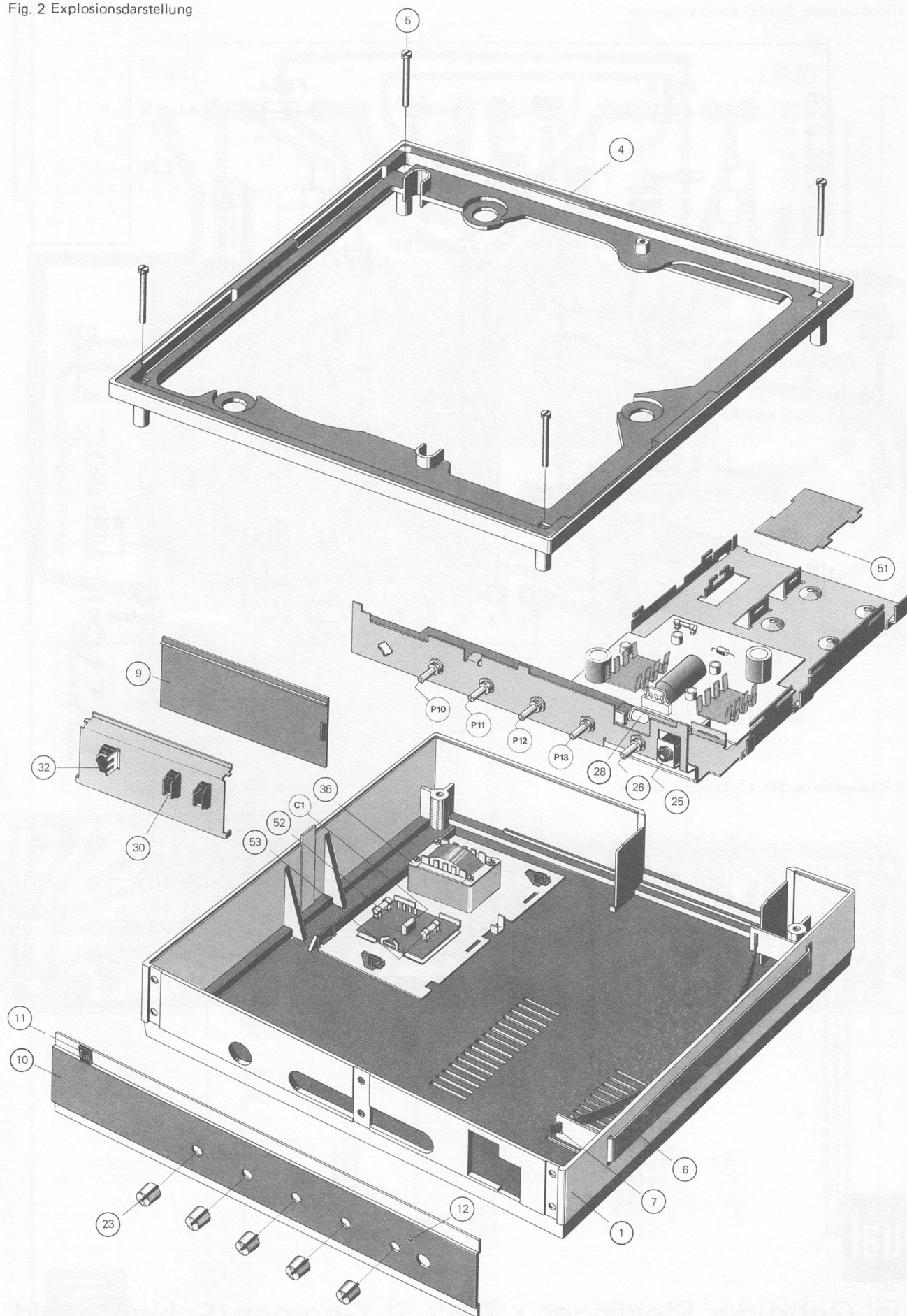
Fig. 2 Explosionsdarstellung
