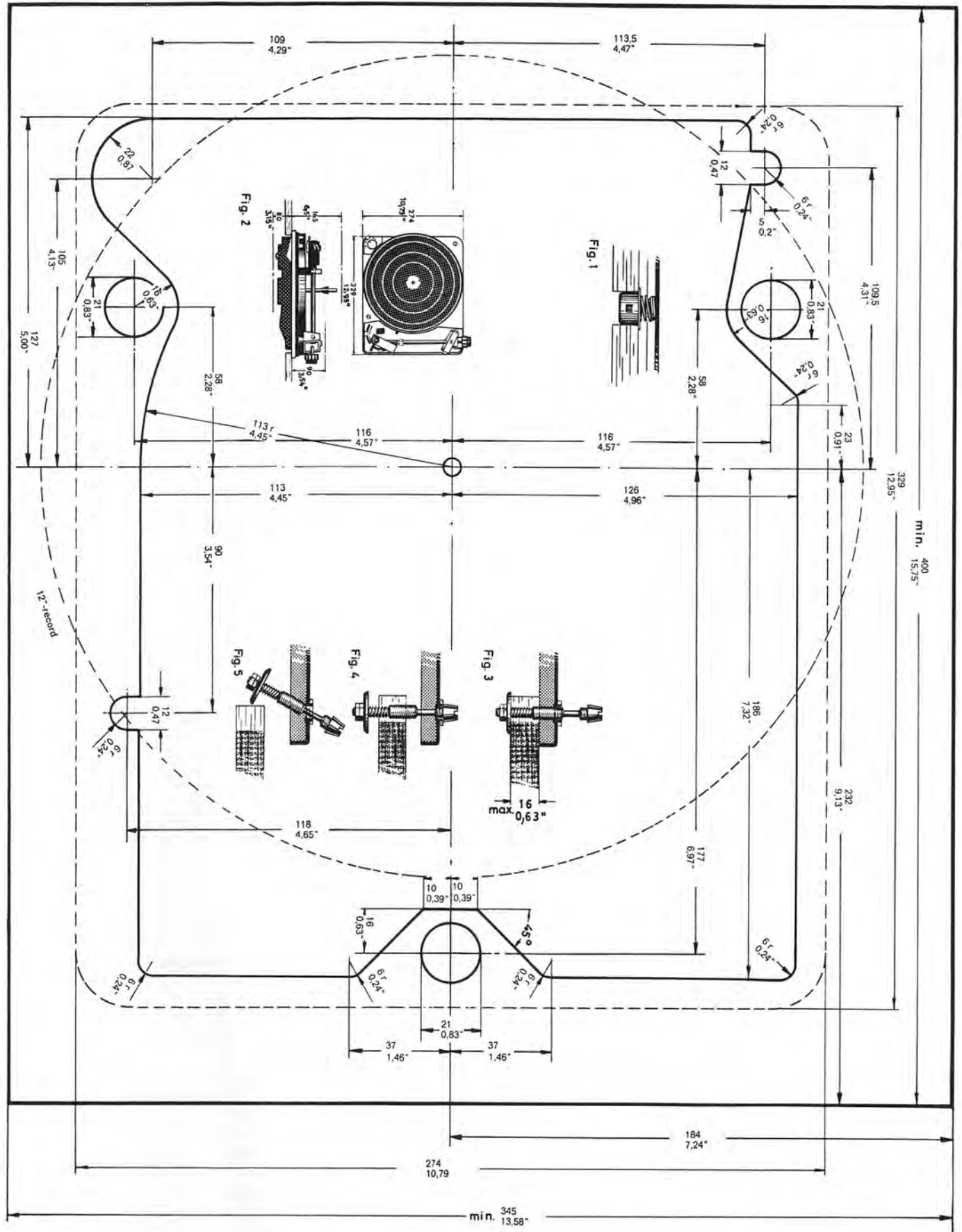
Abb. 14, Einbauschablone
