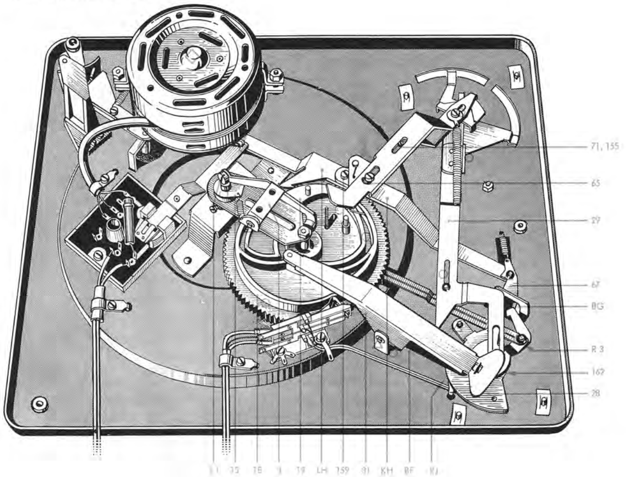
Abb. 13, Chassis von unten
