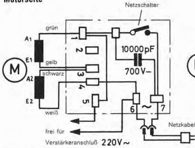
Abb. 11, Schaltbild
