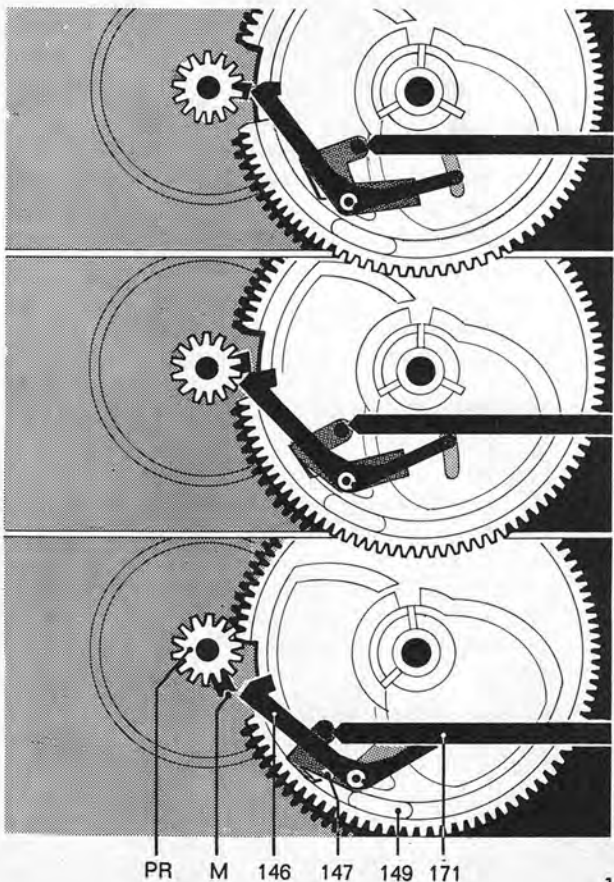
Fig. 14 Einleitung der Wechsel- bzw. Abstellfunktion
