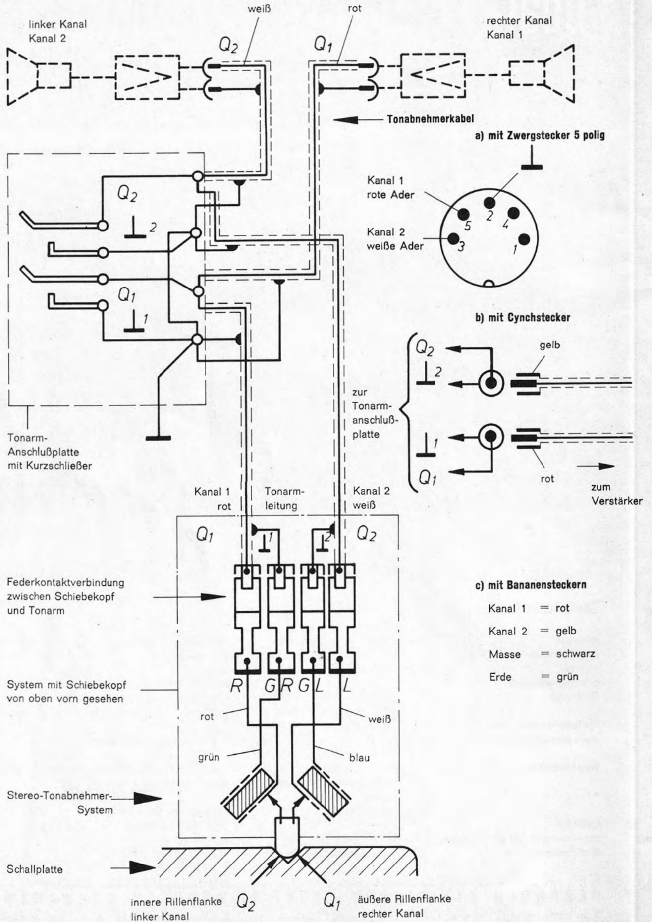
Fig. 1 TA-Anschlußschema
