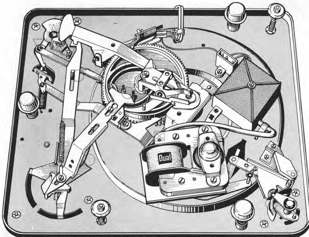
Fig. 18 Chassis von unten
