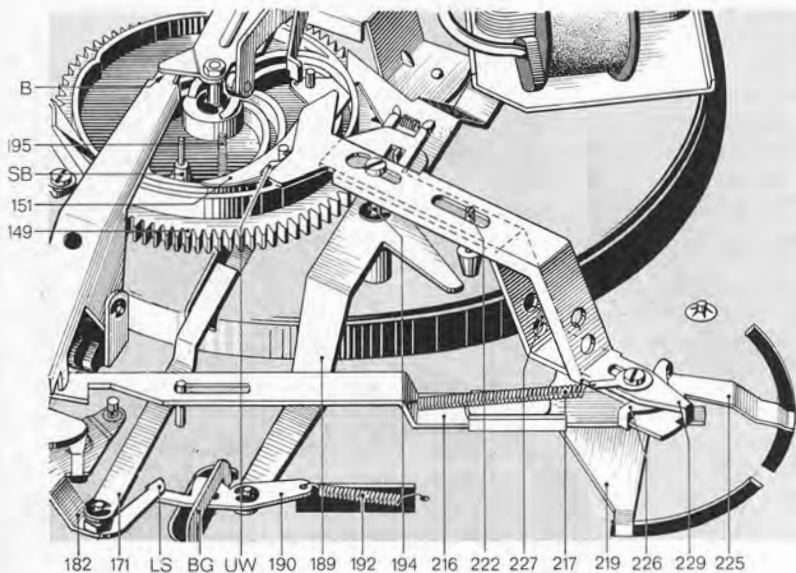
Fig. 9 Funktion „Stop“
