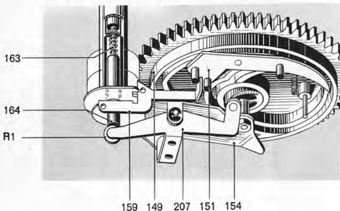
Fig. 13 Endabstellung
