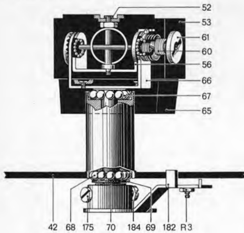
Fig. 5 Tonarmlagerung
