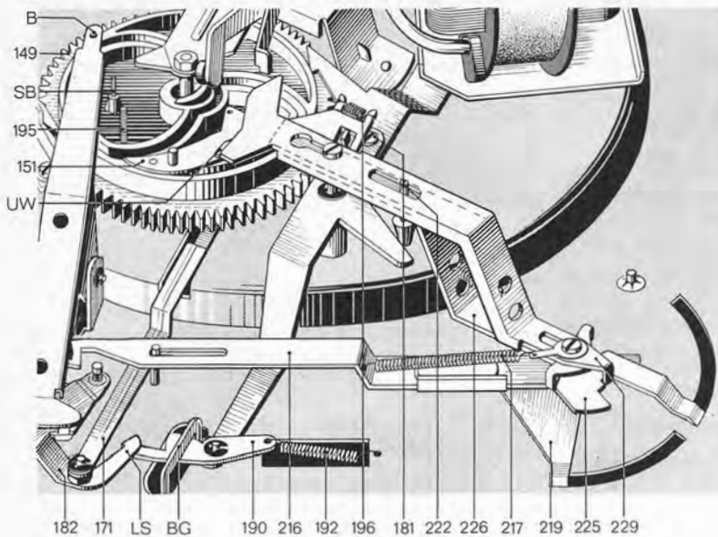
Fig. 9 Funktion „Stop“
