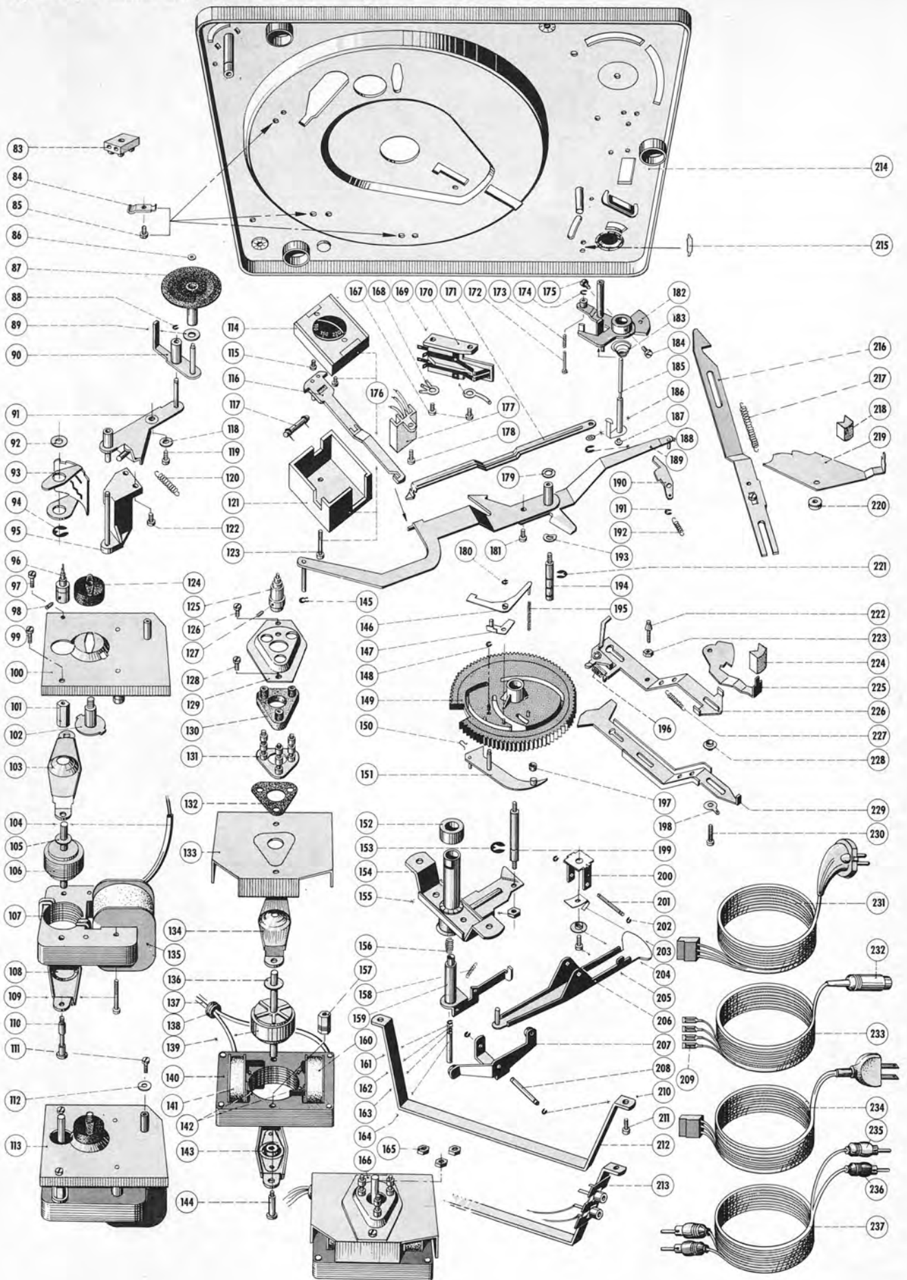
Fig. 16 Explosionsdarstellung, Teile unter der Platine
