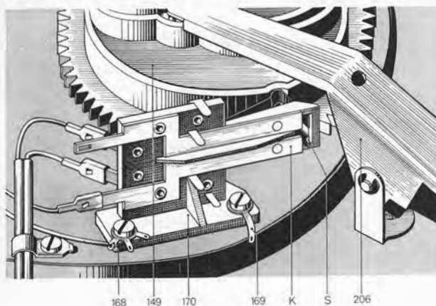
Fig. 10 Kurzschließer
