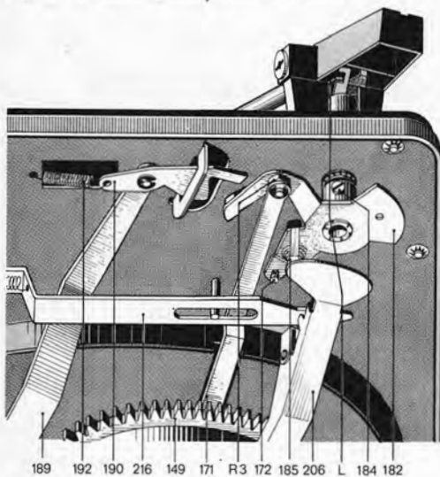
Fig. 6 Tonarmlagerung (Unteransicht)
