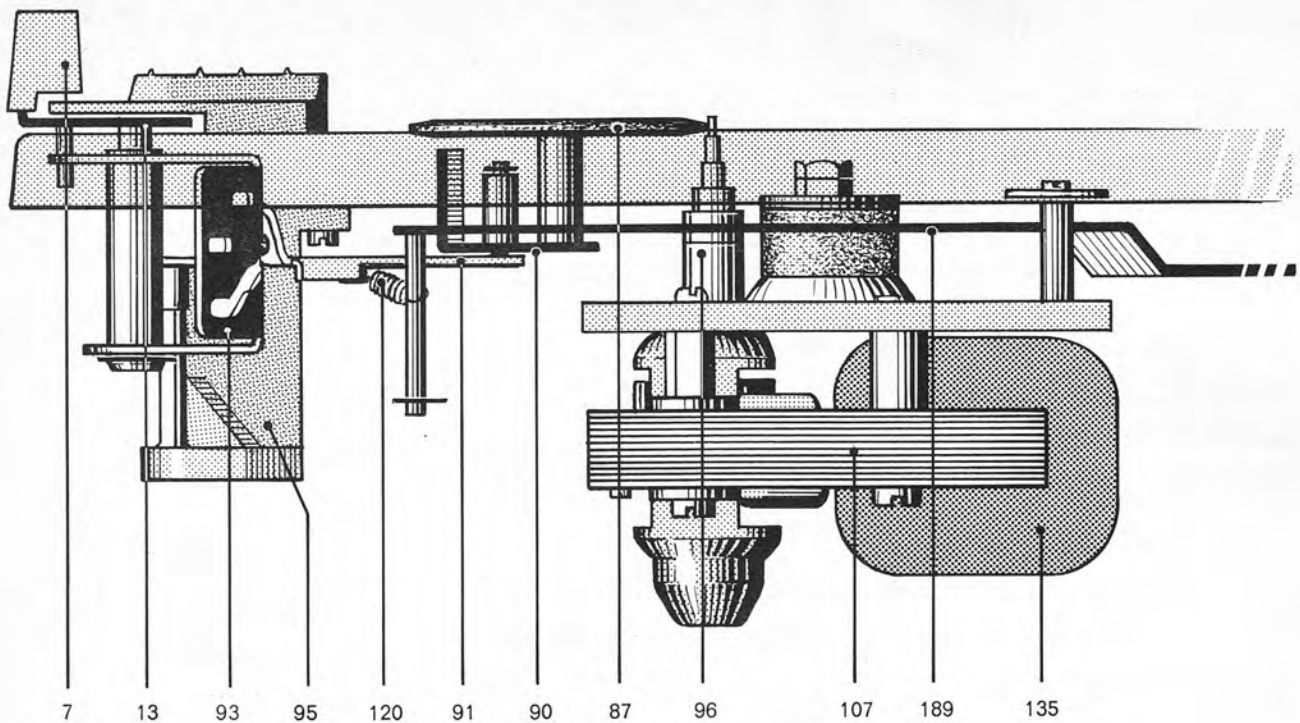
Fig. 2 Motoraufhängung und Antrieb des Plattentellers
