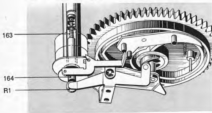
Fig. 12 Wechseltvorgang
