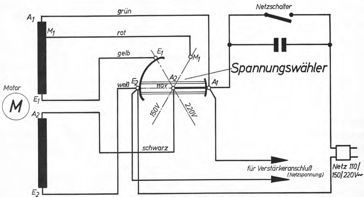
Fig. 3 Anschluß der Feldspule Spannungswähler in Stellung 110 Volt
