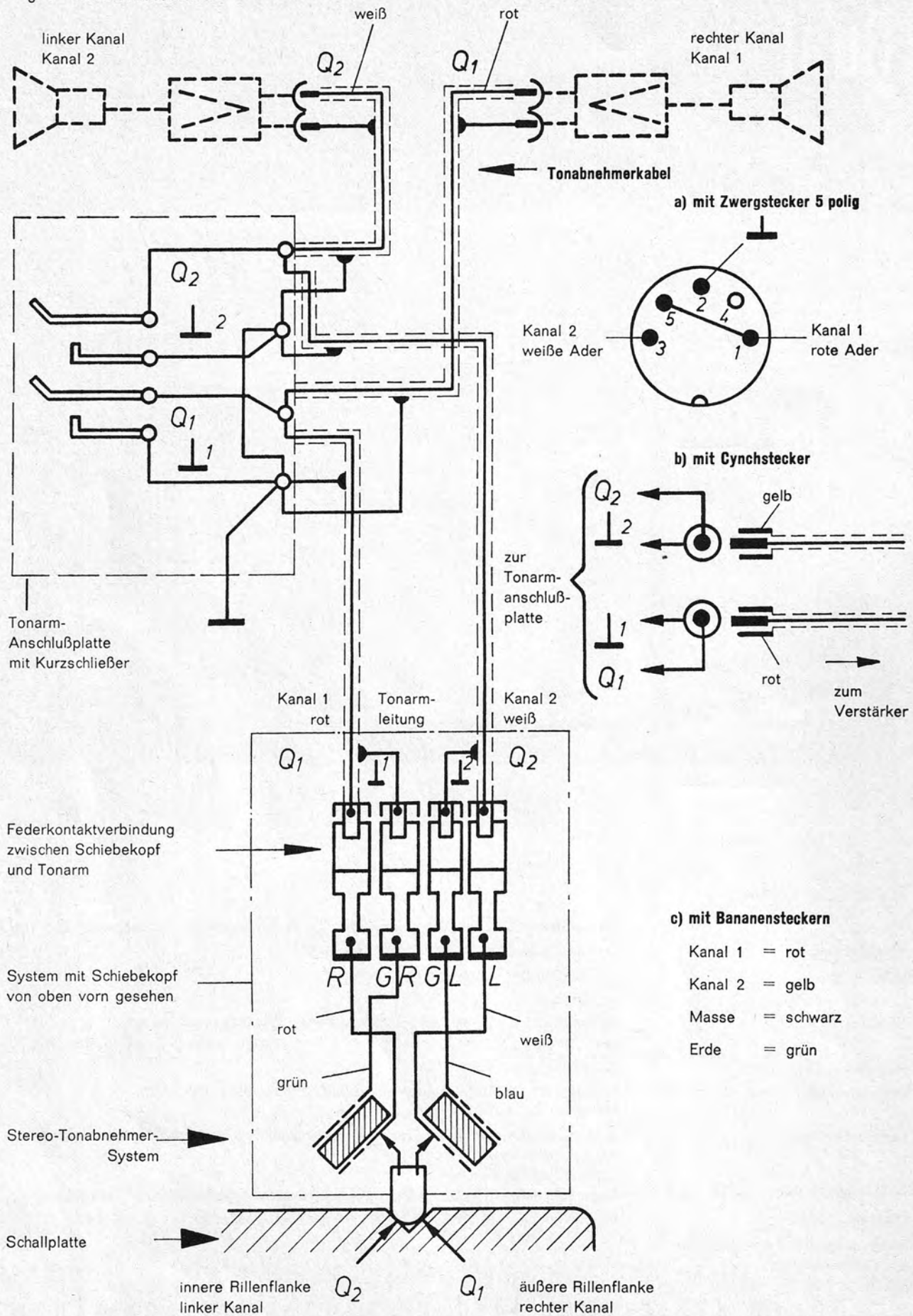
Fig. 1 TA-Anschlußschema
