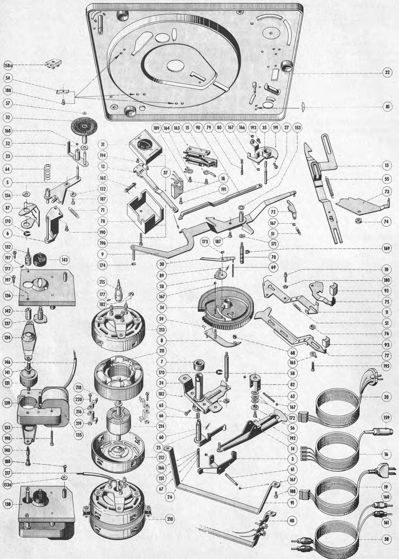
Fig. 17 Teile unter der Platine
