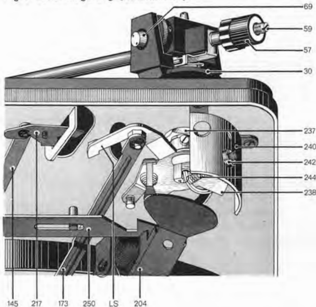
Fig. 7 Tonarmlagerung (Unteransicht)
