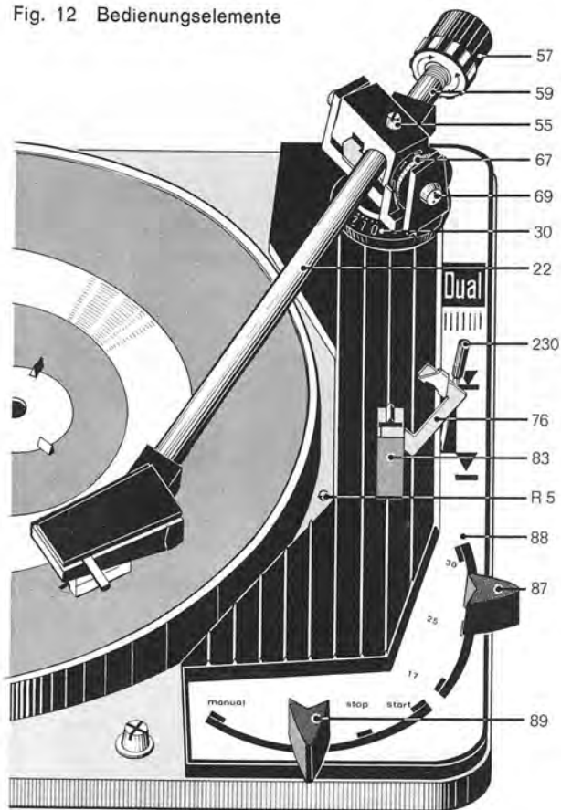
Fig. 12 Bedienungselemente
