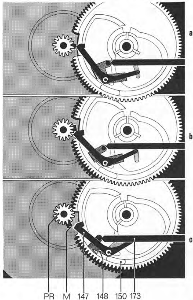
Fig. 18 Einleitung der Wechsel- bzw. Abstellfunktion
