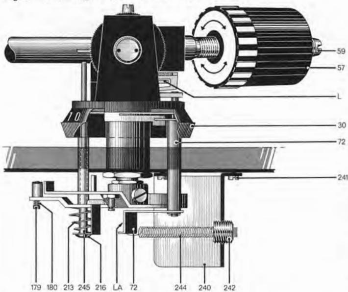
Fig. 7 Tonarmlagerung (Unteransicht)
