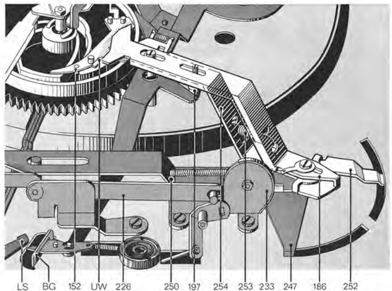
Fig. 14 Funktion „Stop“
