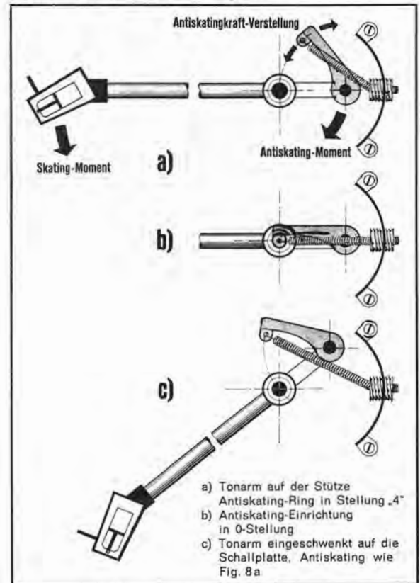
Fig. 8 Skating- und Antiskatingkraft
