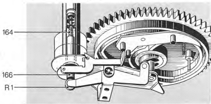
Fig. 16 Wechselvorgang
