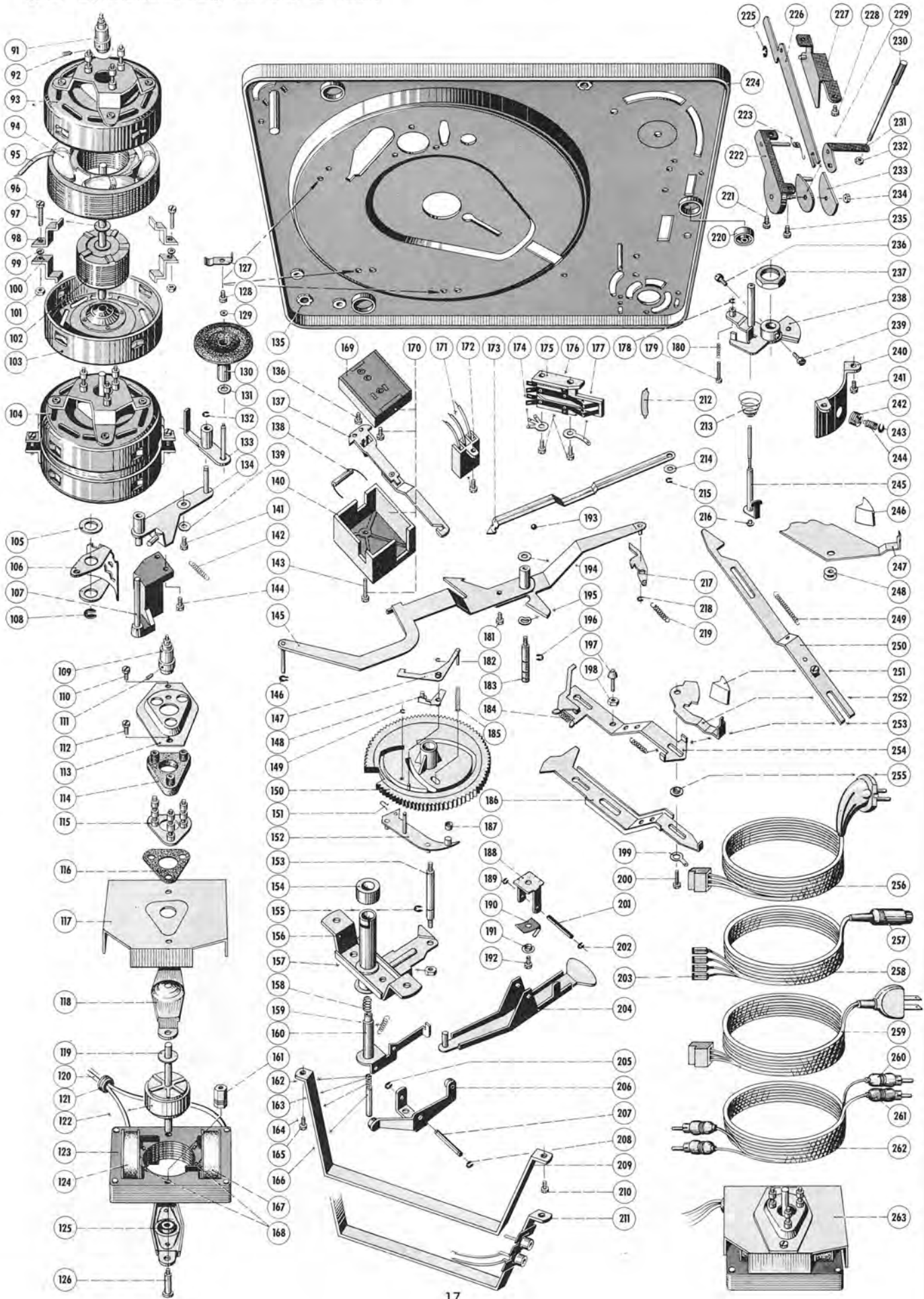
Fig. 20 Explosionsdarstellung, Teile unter der Platine
