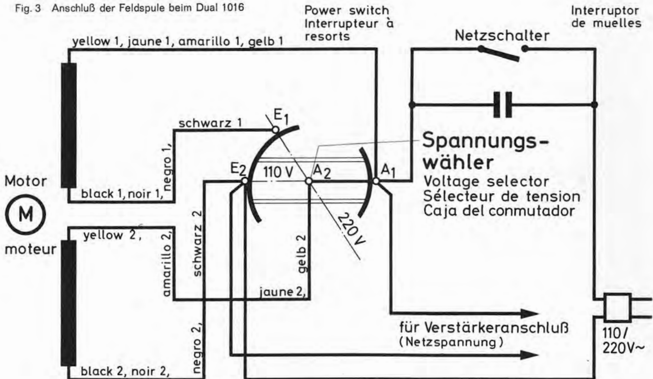
Fig. 3 Anschluß der Feldspule beim Dual 1016
