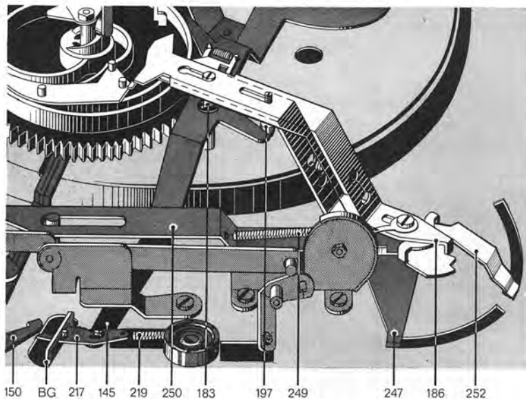
Fig. 13 Startstellung
