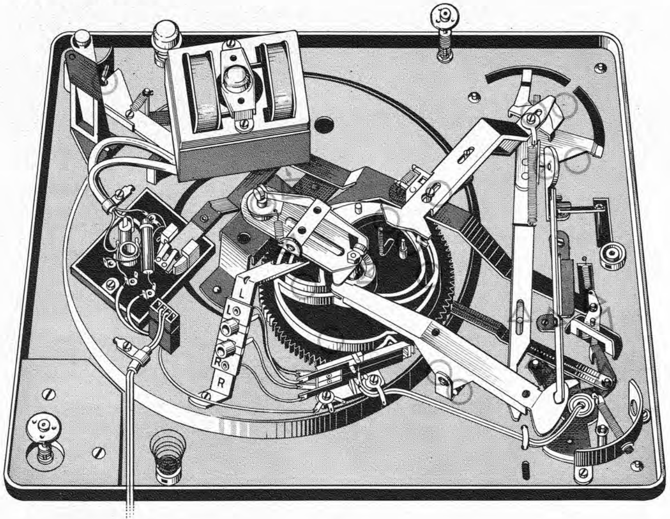
Fig. 22 Chassis, Unteransicht
