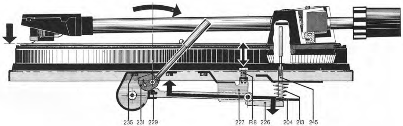
Fig. 11 Tonarmlift in Ruhestellung
