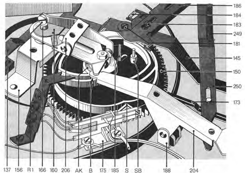
Fig. 15 Schallplattenabwurf
