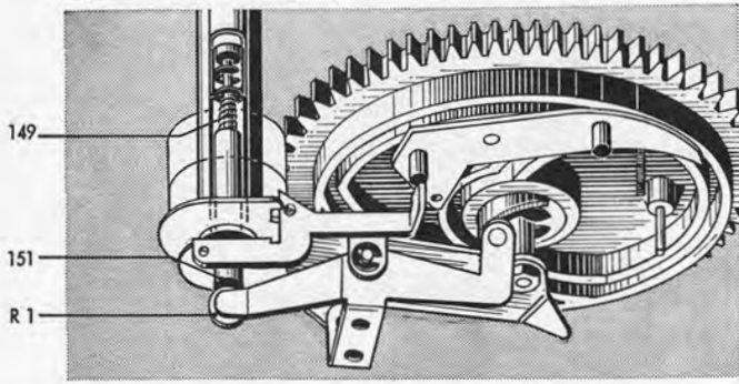
Fig. 16 Wechseltorgang
