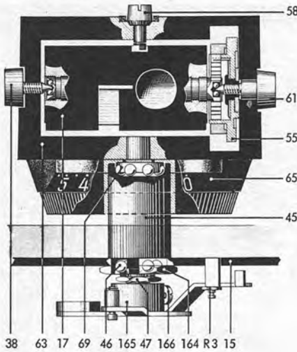
Fig. 5 Tonarmlagerung
