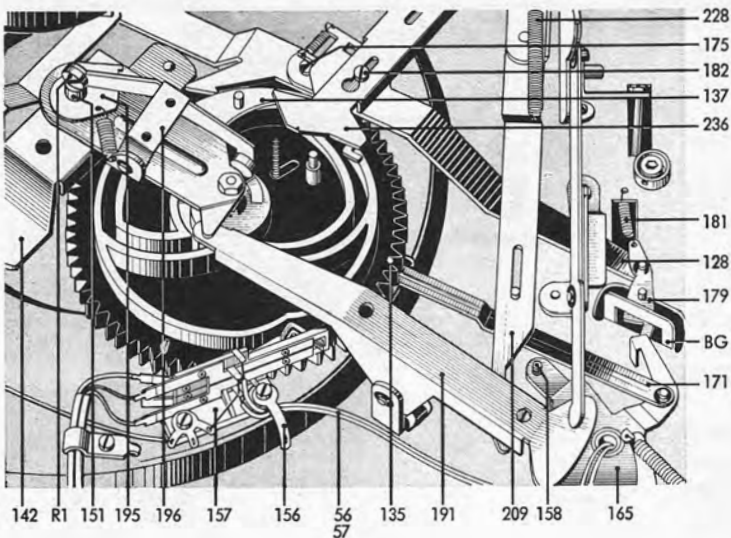
Fig. 9 Kinematik der Tonarmsteuerung
