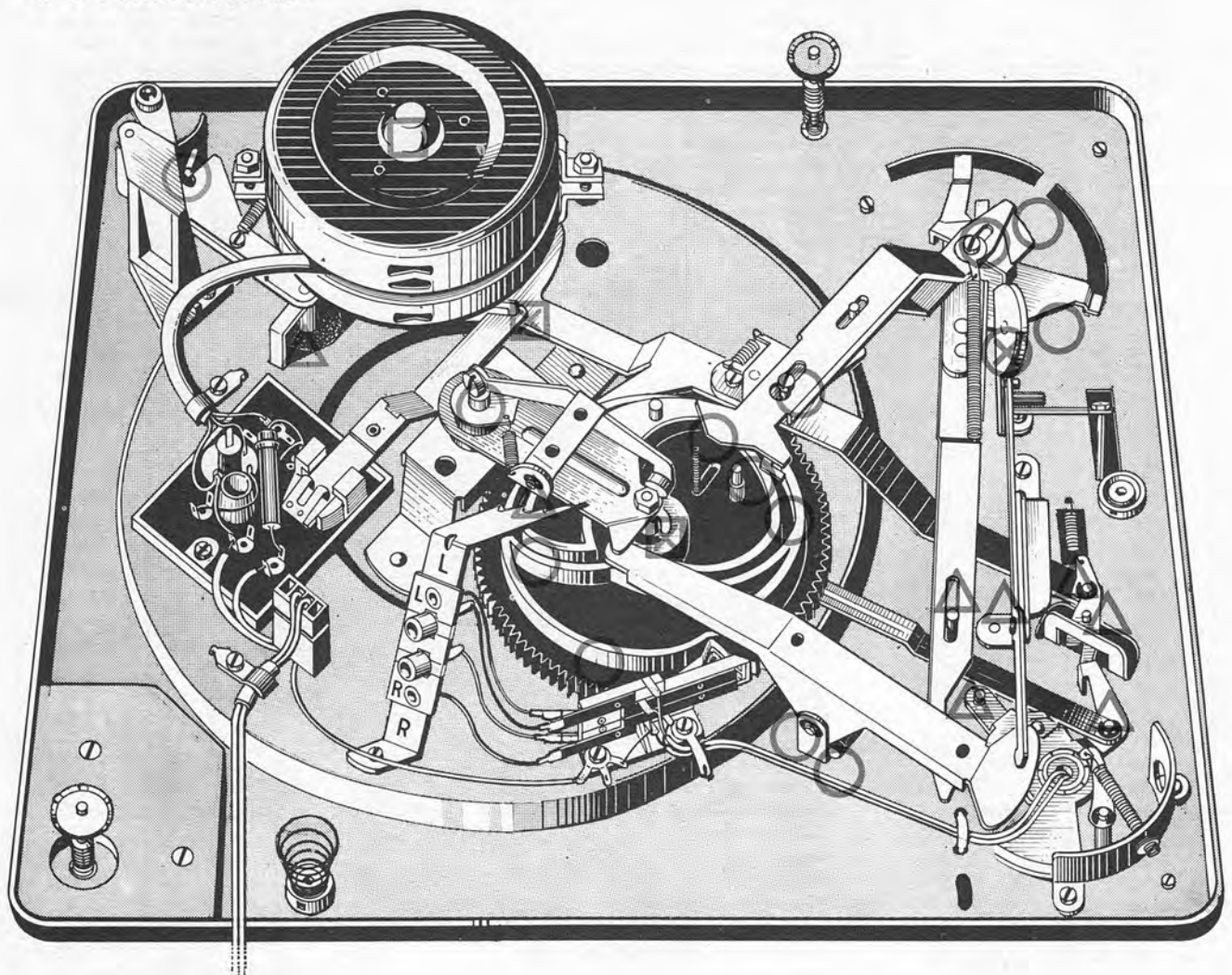
Fig. 20 Chassis, Unteransicht
