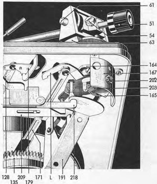
Fig. 7 Tonarmlagerung (Unteransicht)
