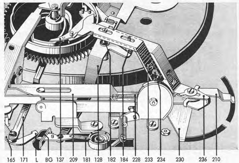
Fig. 14 Funktion „Stop“
