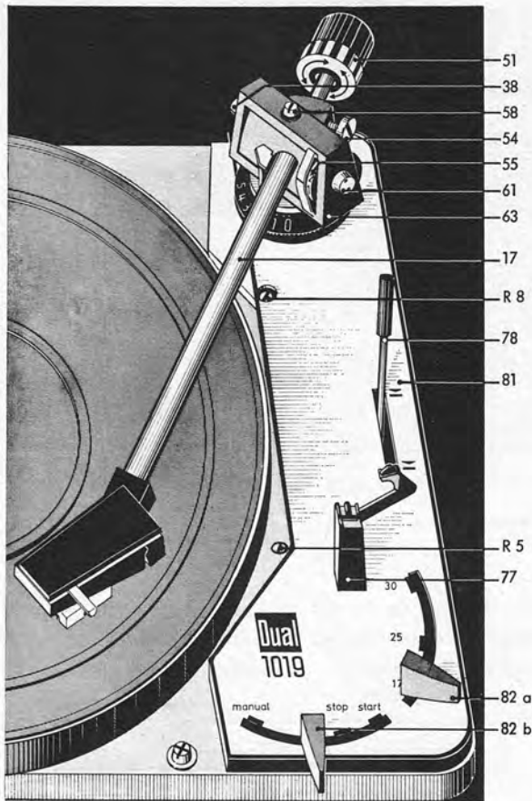
Fig. 12 Bedienungselemente
