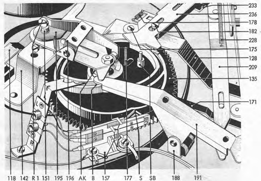
Fig. 15 Schallplattenabwurf
