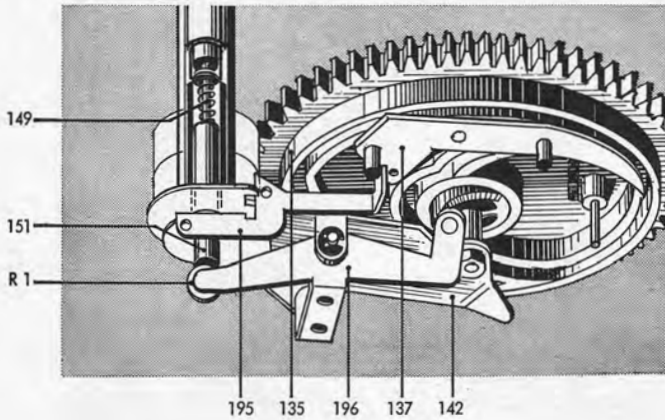
Fig. 18 Einleitung der Wechsel- bzw. Abstellfunktion
