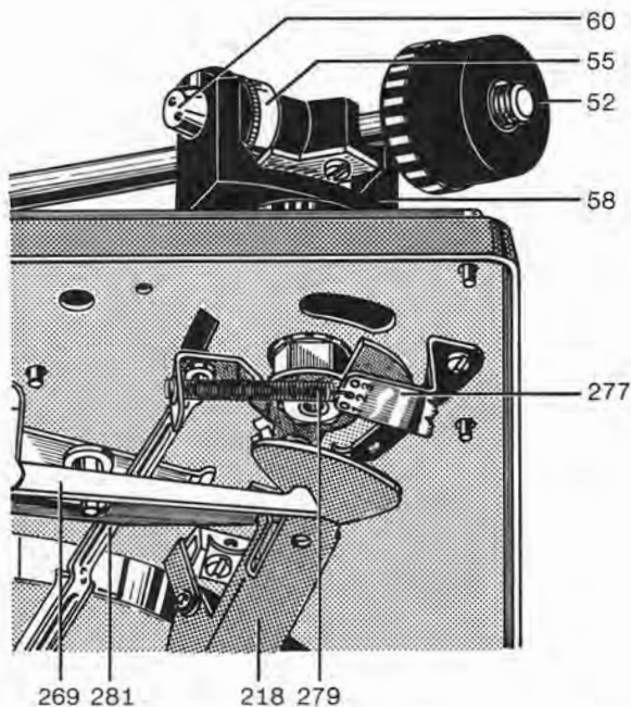
Fig. 8 Tonarmlagerung (Unteransicht)
