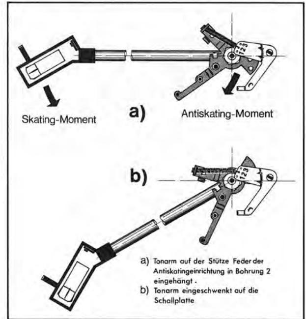
Fig. 9 Antiskatingkraft
