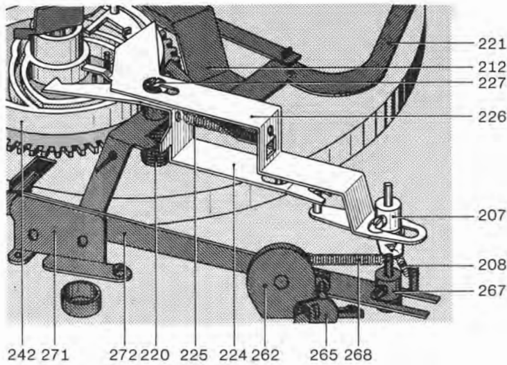
Fig. 13 Stoppstellung
