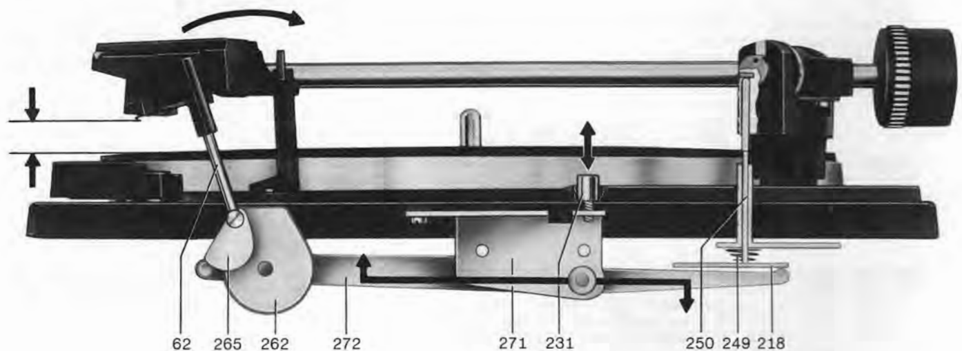
Fig. 11 Tonarmlift (Tonarm abgehoben)
