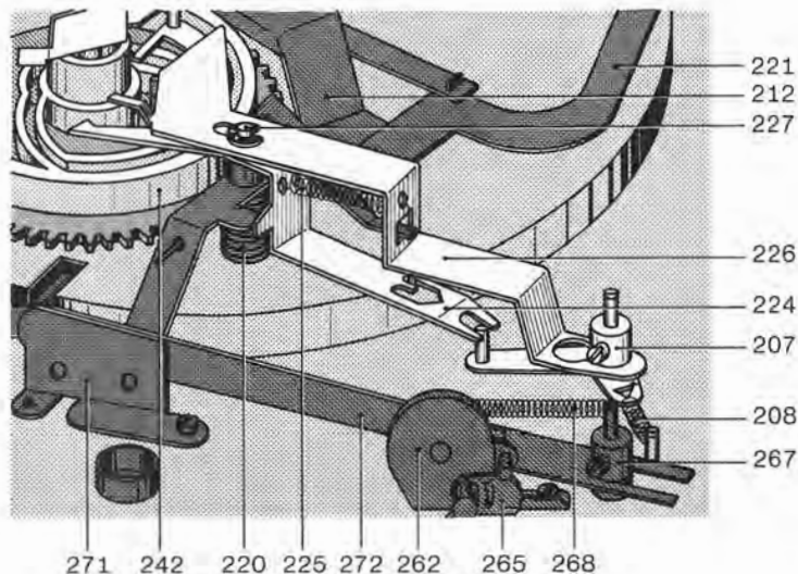
Fig. 12 Startstellung
