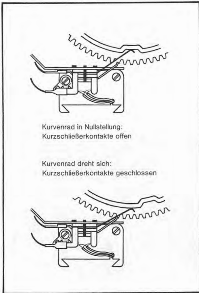
Fig. 14 Kurzschließer
