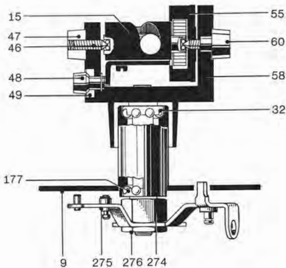
Fig. 7 Tonarmlagerung
