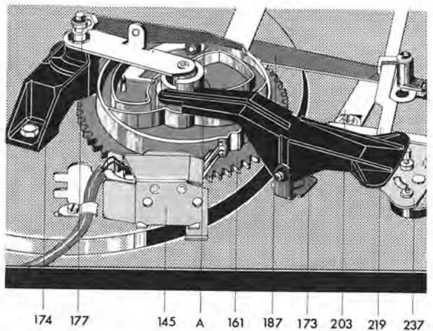
Fig. 15 Schallplattenabwurf
