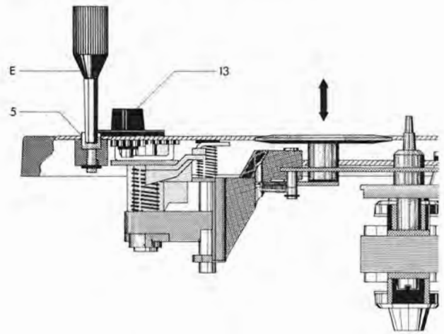
Fig. 5 Stellung des Treibrades
