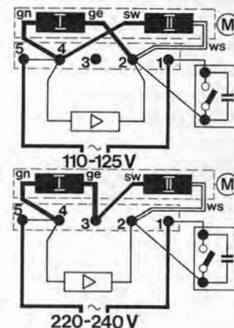
Fig. 4 Anschluß der Feldspulen (mit Anschlußplatte)
