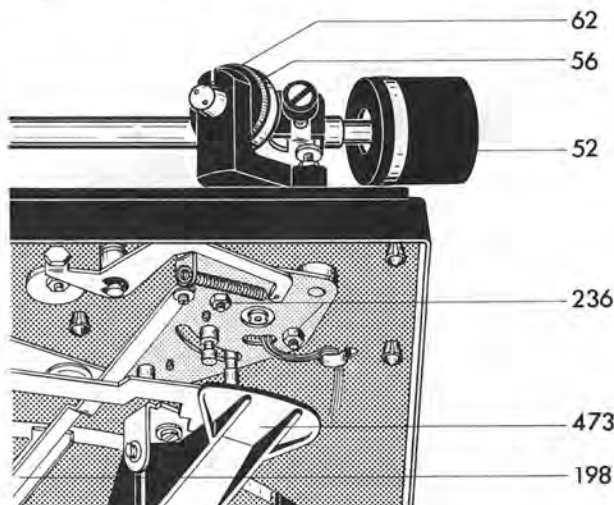
Fig. 8 Tonarmlagerung (Unteransicht)
