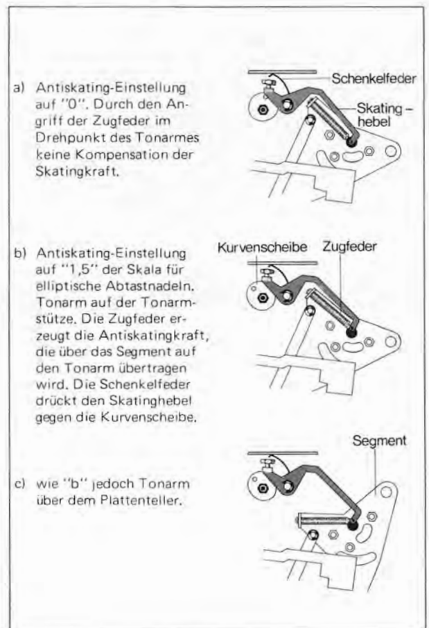
Fig. 9 Antiskatingkraft
