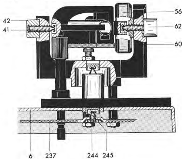
Fig. 7 Tonarmlagerung
