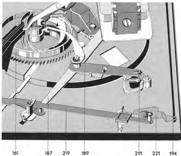
Fig. 13 Stoppstellung
