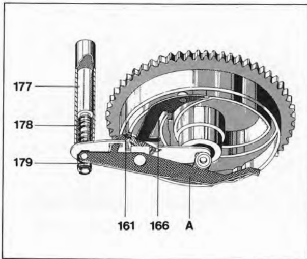
Fig. 17 Wechselvorgang
