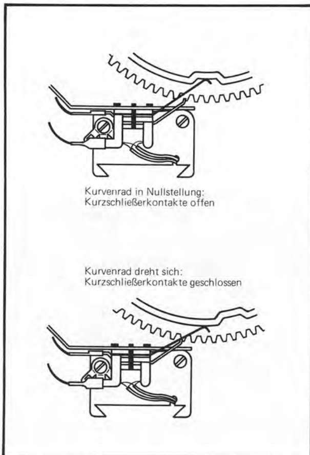
Fig. 14 Kurzschließer
