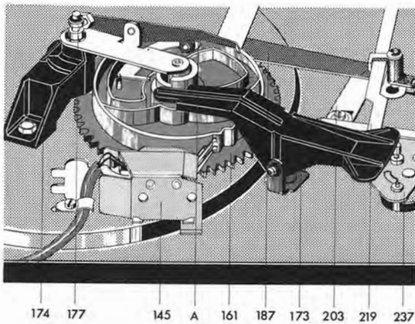
Fig. 10 Kinematik der Tonarmsteuerung
