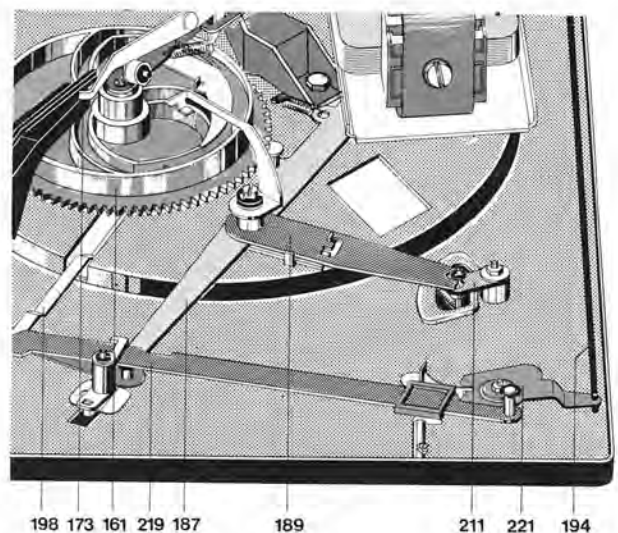
Fig. 12 Startstellung
