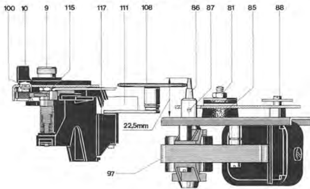
Fig. 2 Motoraufhängung und Antrieb 2-Pol-Motor
