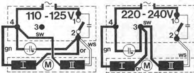
Fig. 4 Motoranschlußschema
