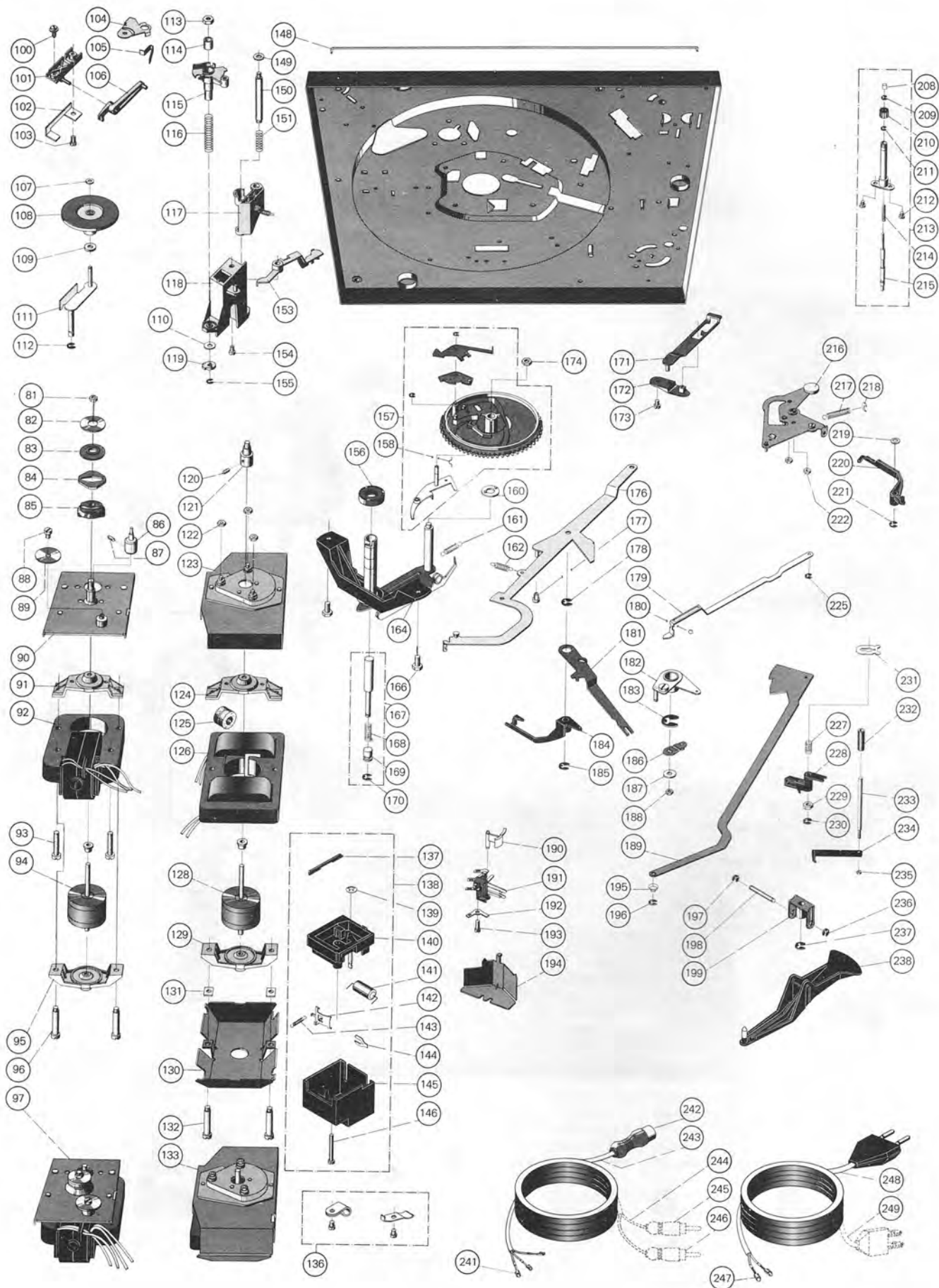
Fig. 18 Explosionszeichnung 2
