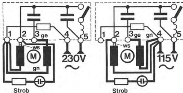
Schalterplatte / Switch plate / Plaque de manoeuvre
