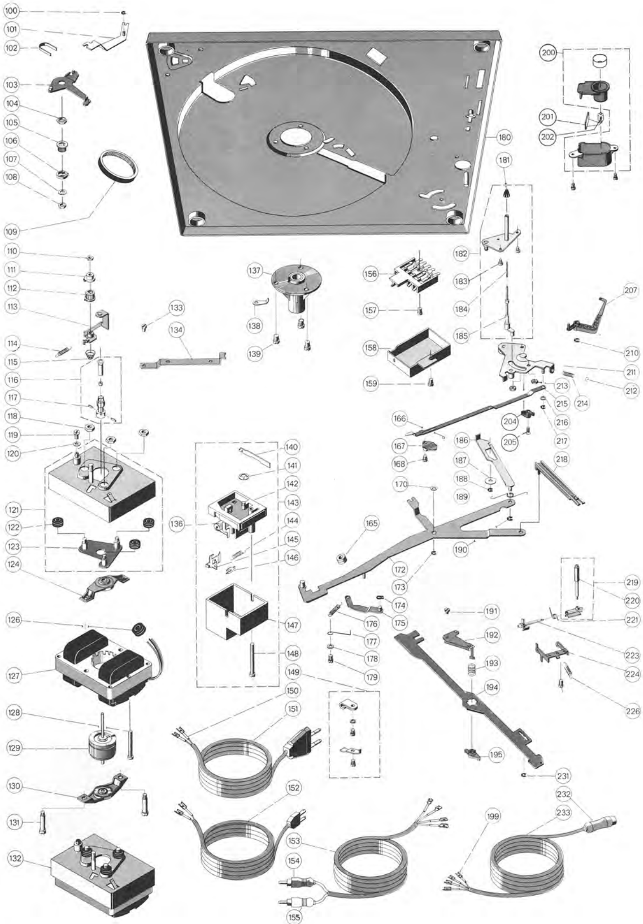
Fig. 13 Explosionszeichnung 2
