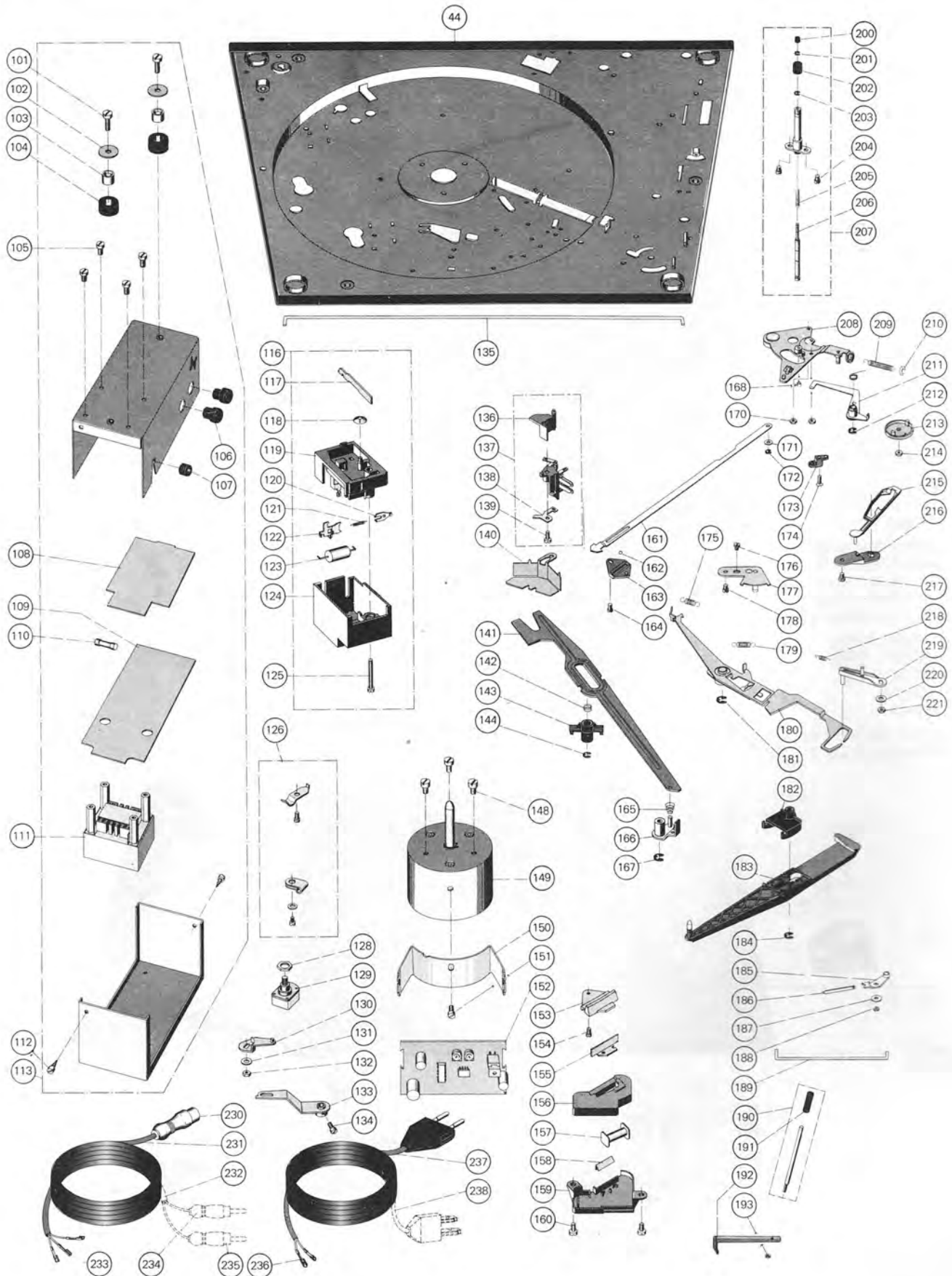
Fig. 23 Explosionsdarstellung 2
