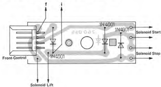
Fig. 5 Solenoid-Anschlußplatte (Bestückungsseite)
