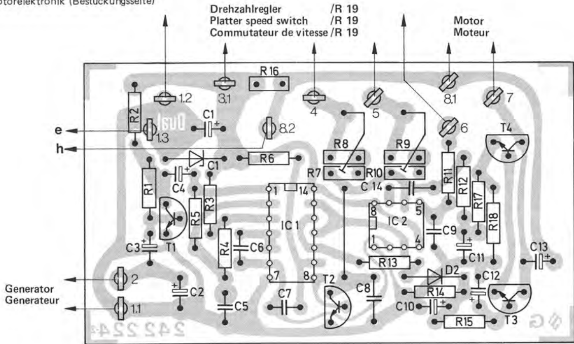
Fig. 3 Motorelektronik (Bestückungsseite)
