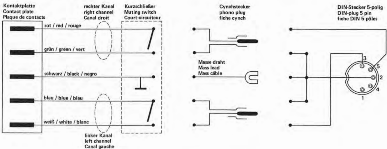
Fig. 1 TA-Anschlußschema
