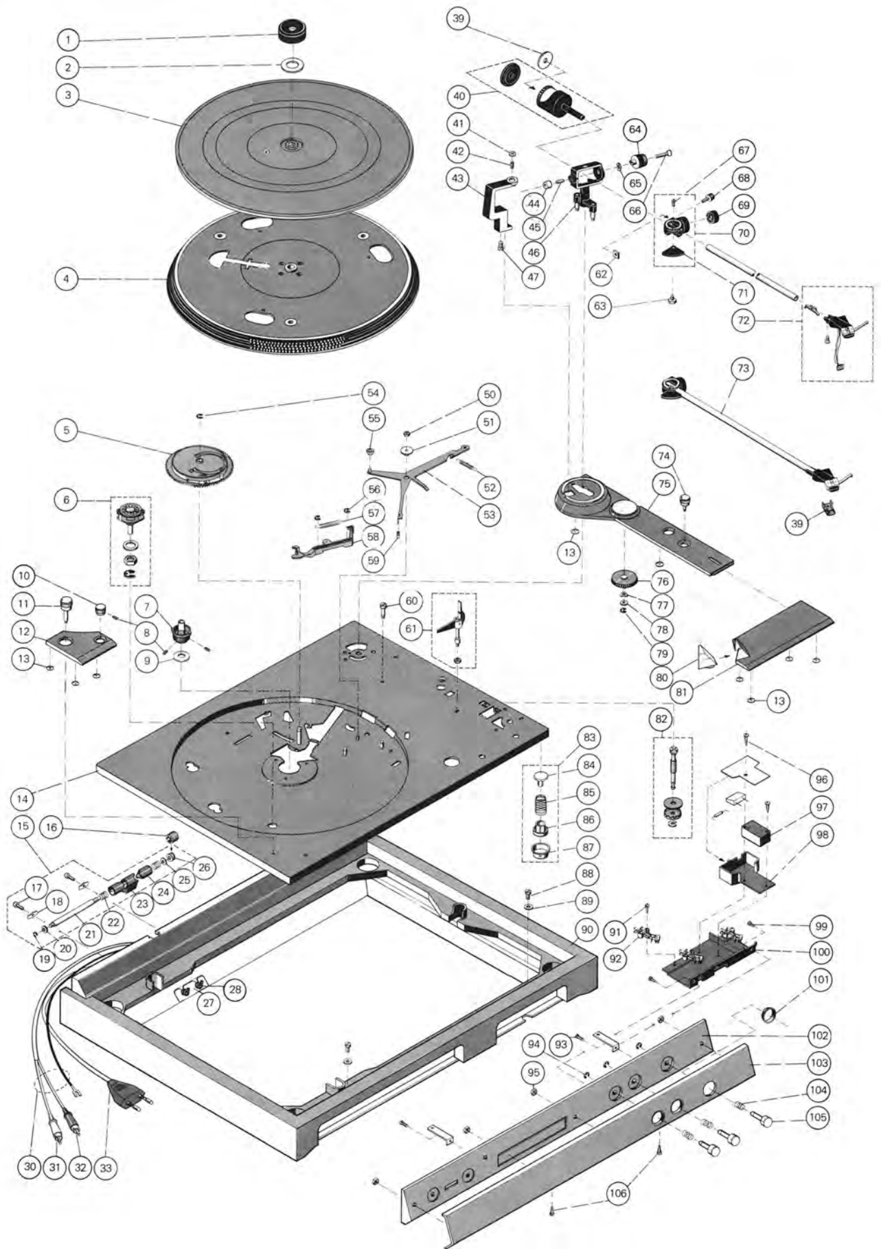
Fig. 24 Explosionsdarstellung 1
