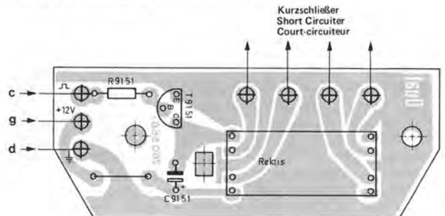
Fig. 6 Stummschaltung (Bestückungsseite)
