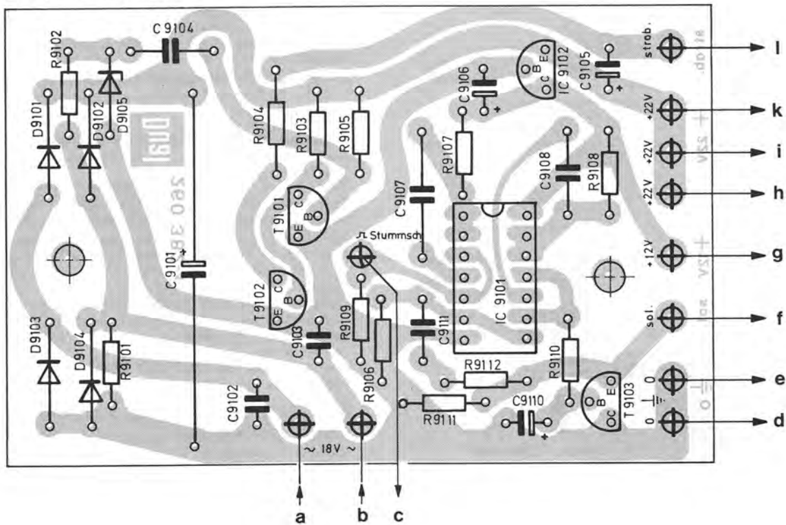
Fig. 5 Solenoid-Anschlußplatte (Bestückungsseite)
