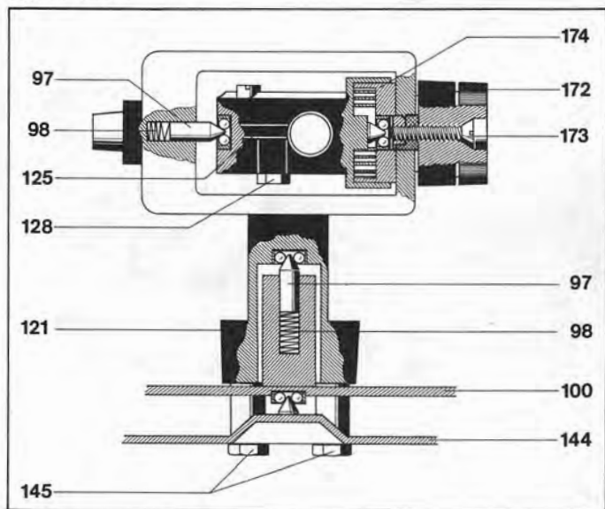
Federhaus-Tonarm / Spring housing tonearm / Bras de lecture avec cage de ressort
