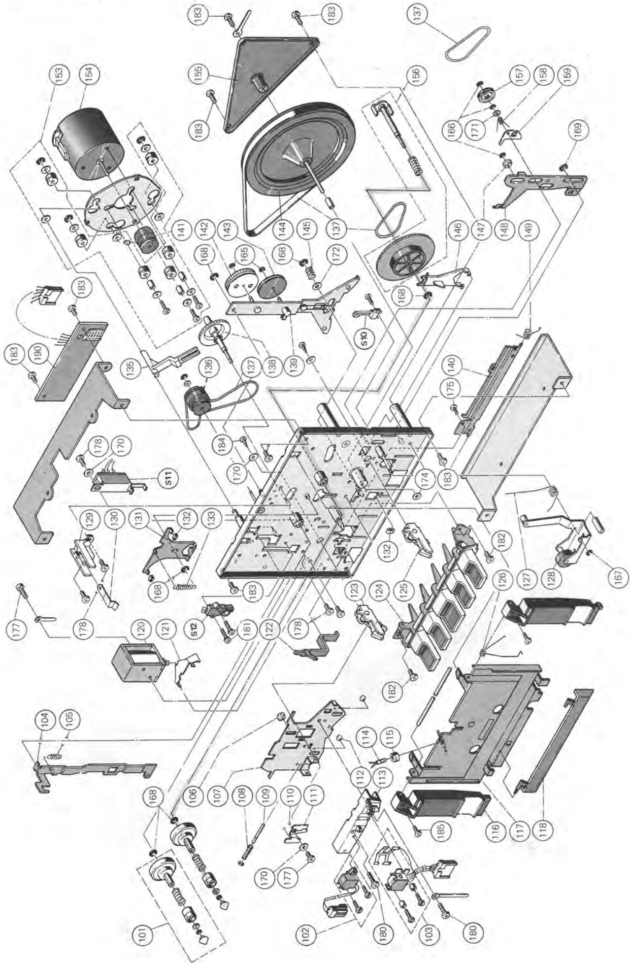
Fig. 14 Explosionszeichnung 2
