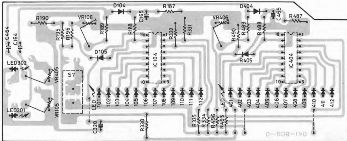
Fig. 2 LED-Anzeigeplatte
