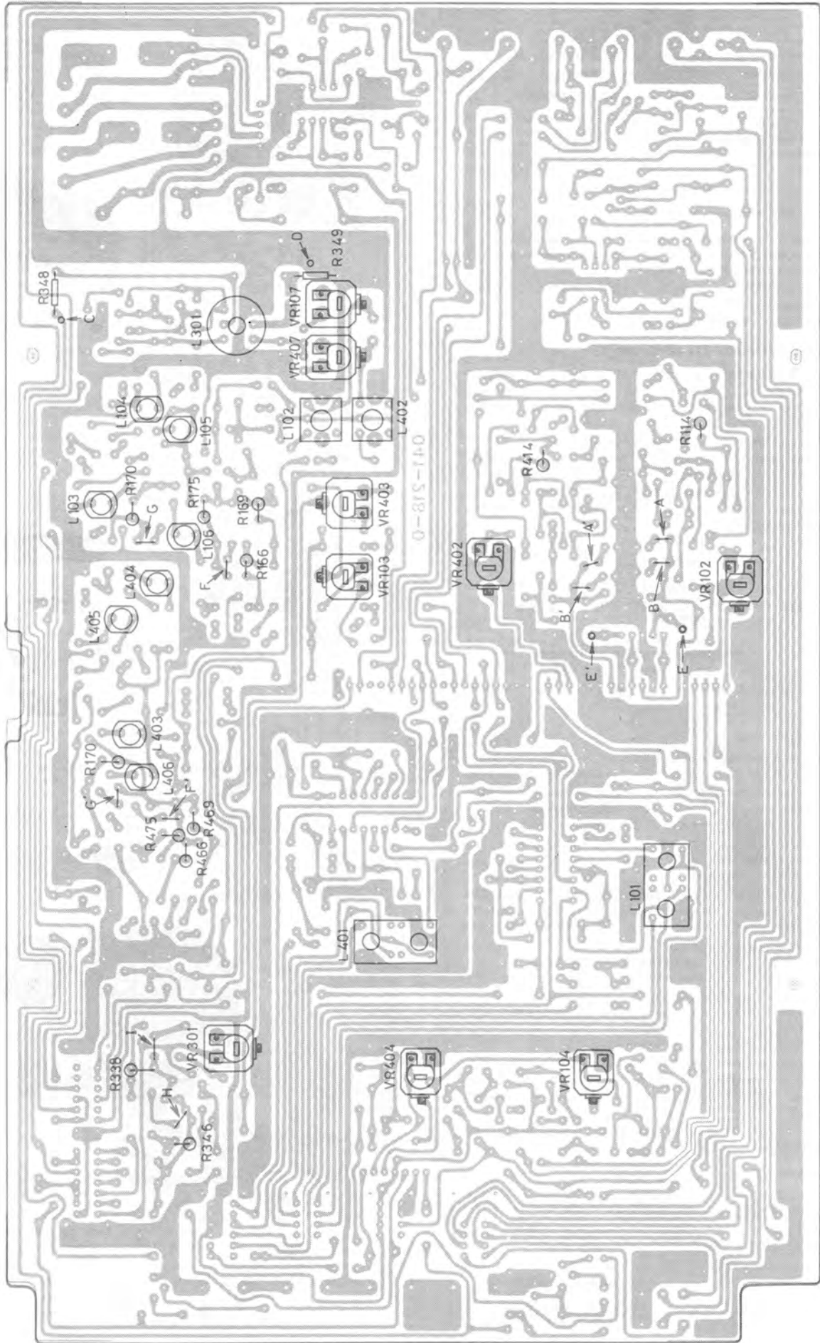
Fig. 1 Abgleichpositionen
