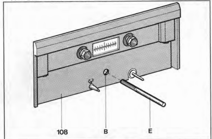
Aufnahme/Wiedergabekopf / Record/Playback head / Tête d'enregistrement
