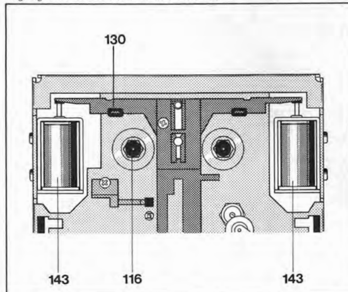
Zugmagnete / Solenoid / Aimants d'attraction
