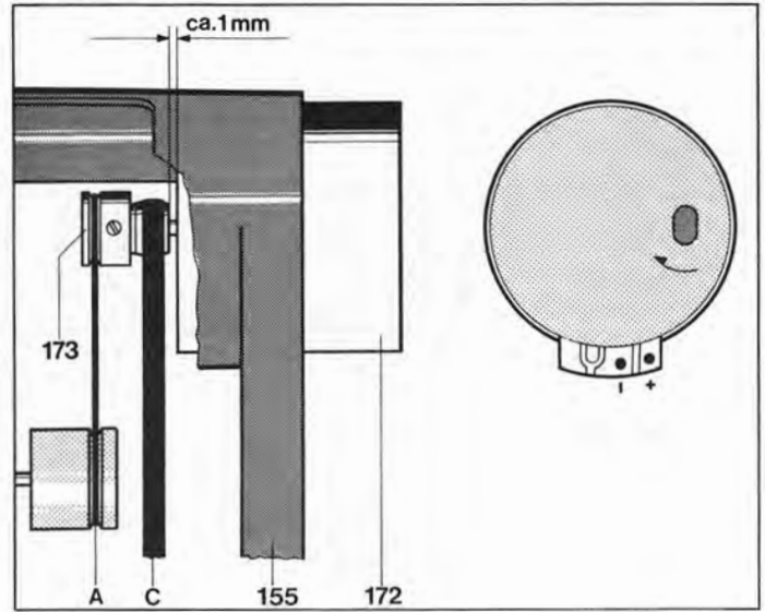
Riemenlaufplan / Belt diagram / Schéma de disposition de la courroie
