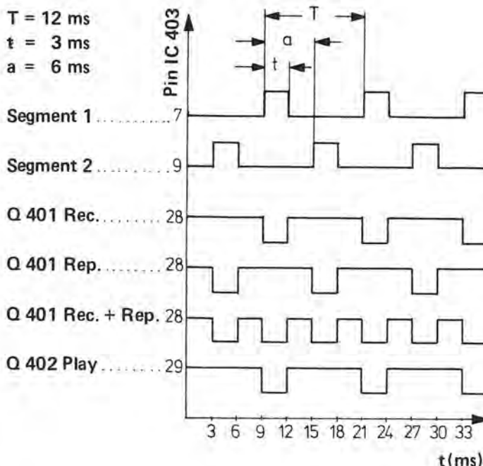
Pulse-Diagramm IC 403
