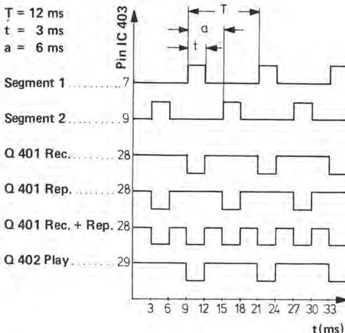
Pulse-Diagramm IC 403
