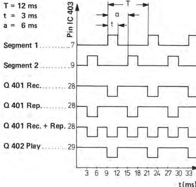
Pulse-Diagramm IC 403
