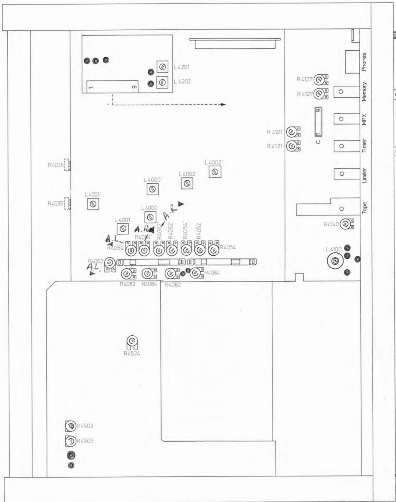
Fig. 1 Abgleichpositionen
