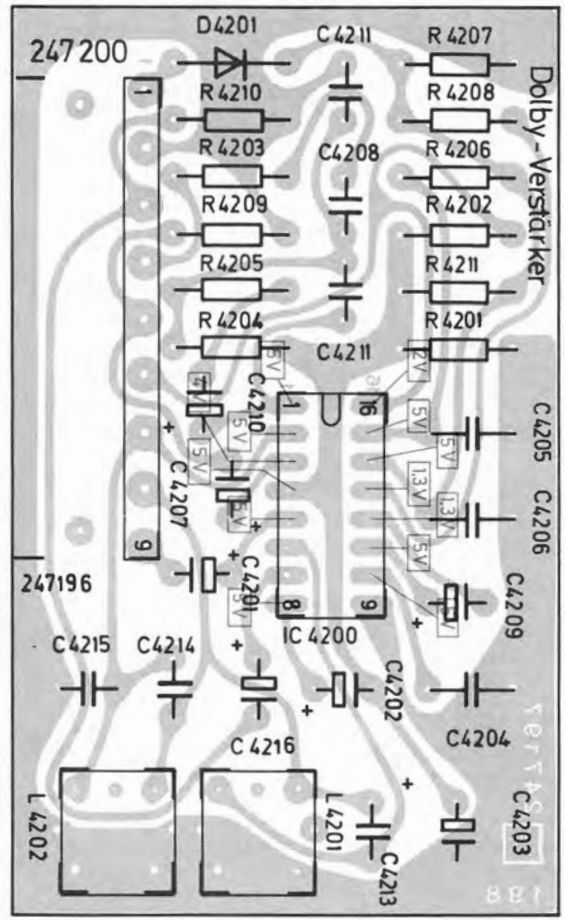
Fig. 11 Dolby-Verstärker 262 448 Bestückungsseite
