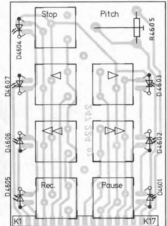
Fig. 12 Tipptastenplatte 262 469 Bestückungsseite
