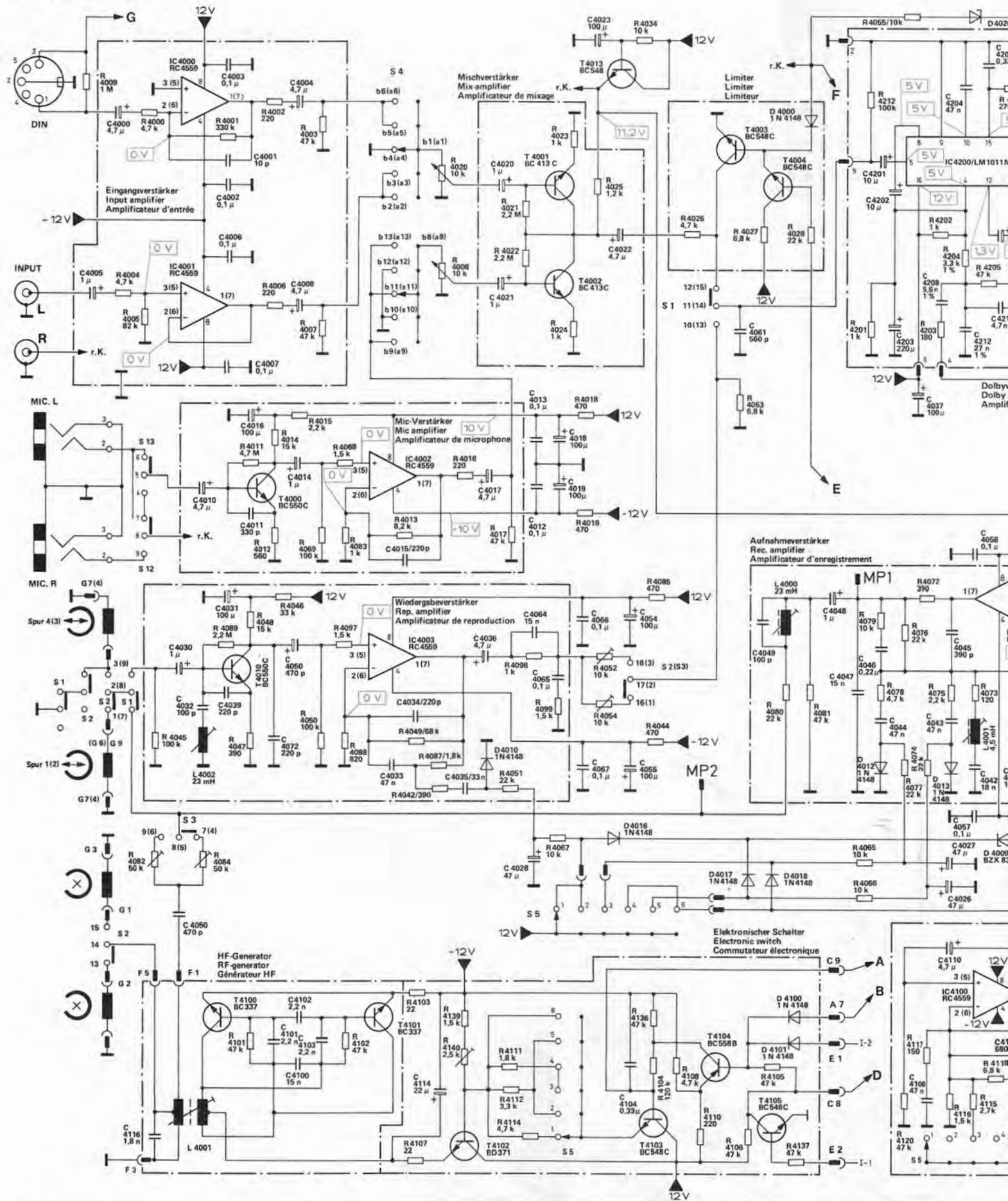
Fig. 5 Schaltbild Analogteil
