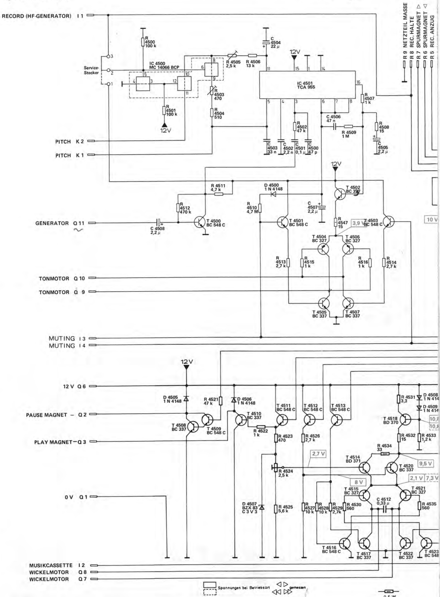
Fig. 4 Motorelektronik
