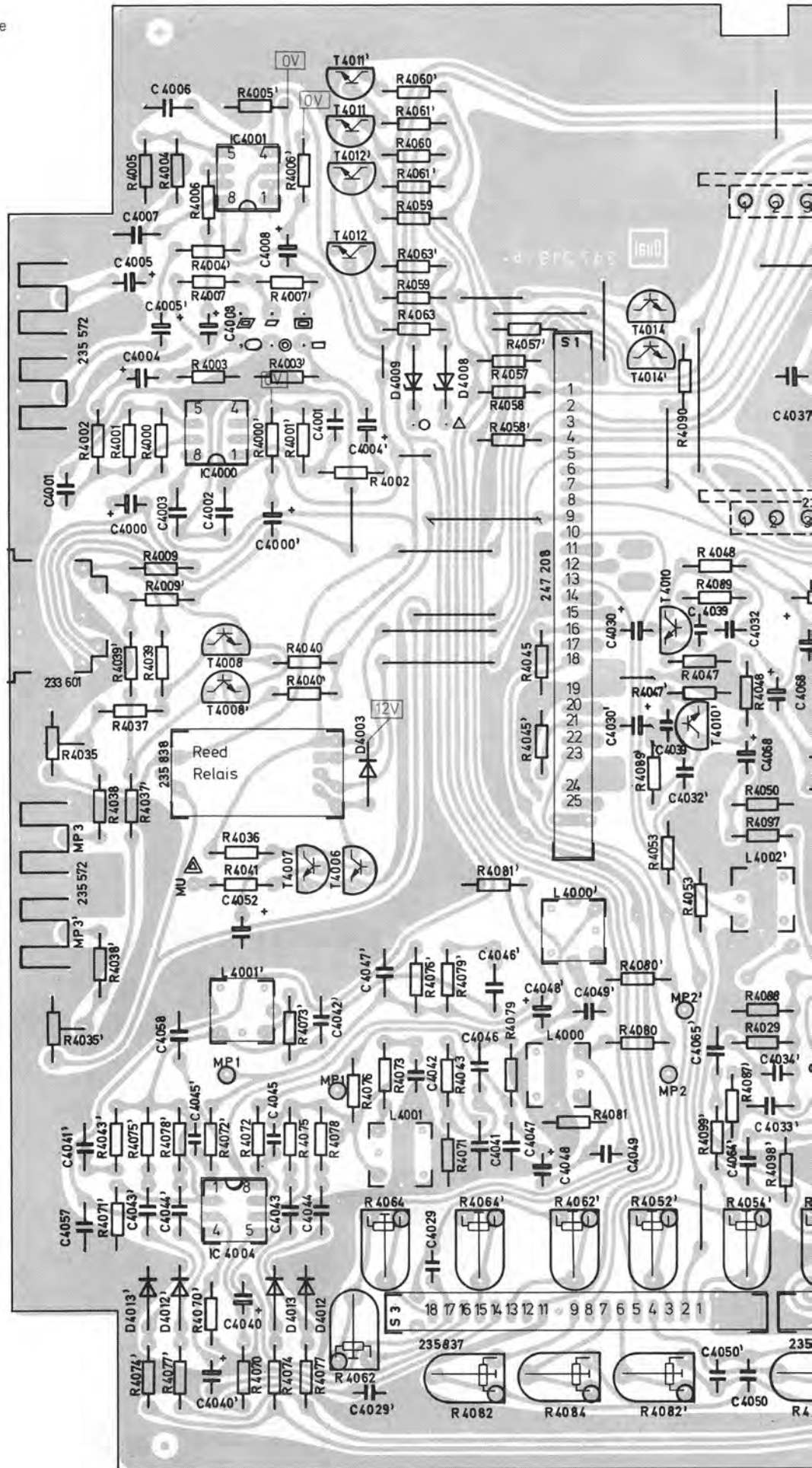
Fig. 6 Grundplatte 262 451 Bestückungsseite
