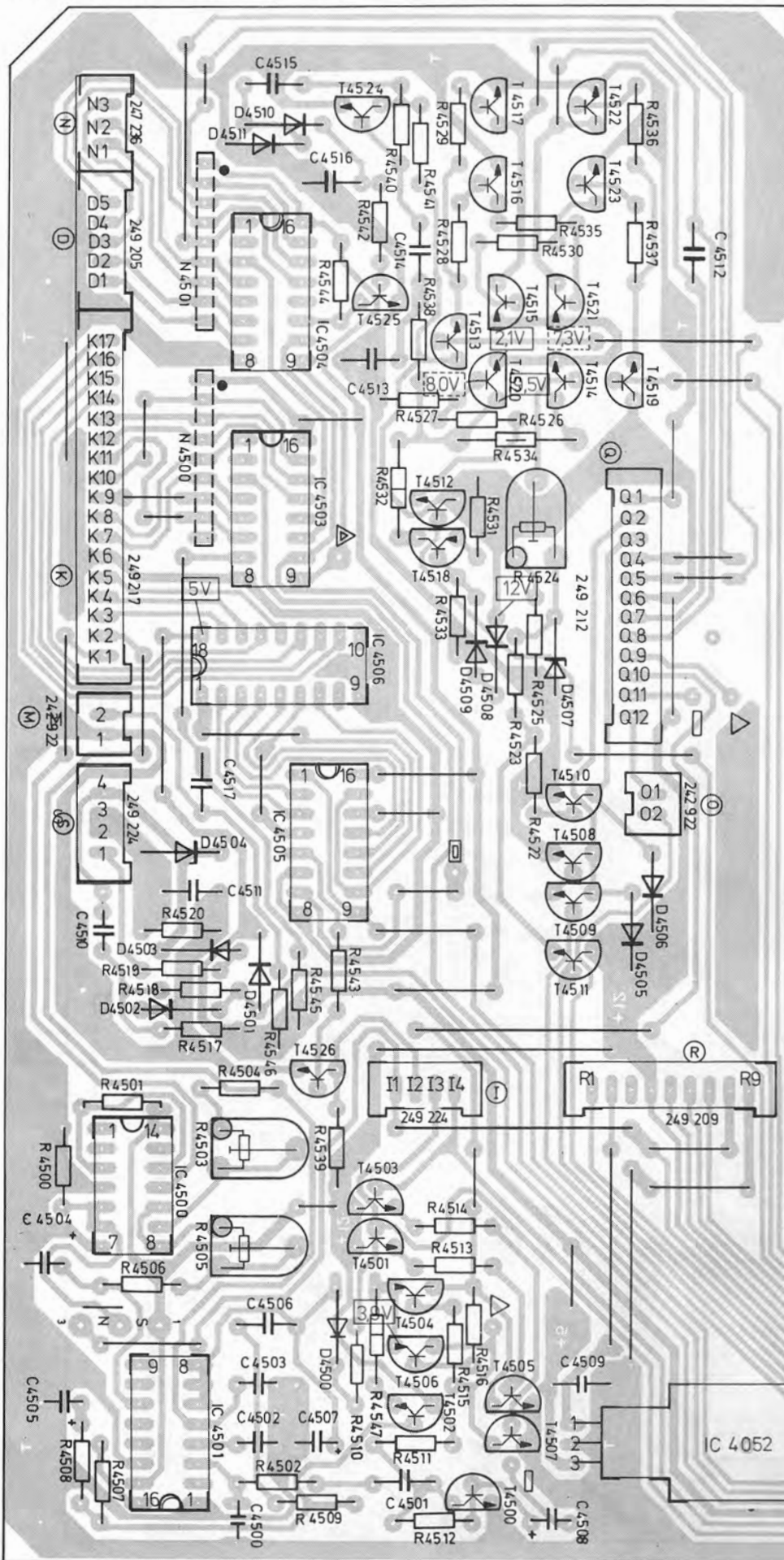
Fig. 7 Motorelektronik 262 460 Bestückungsseite
