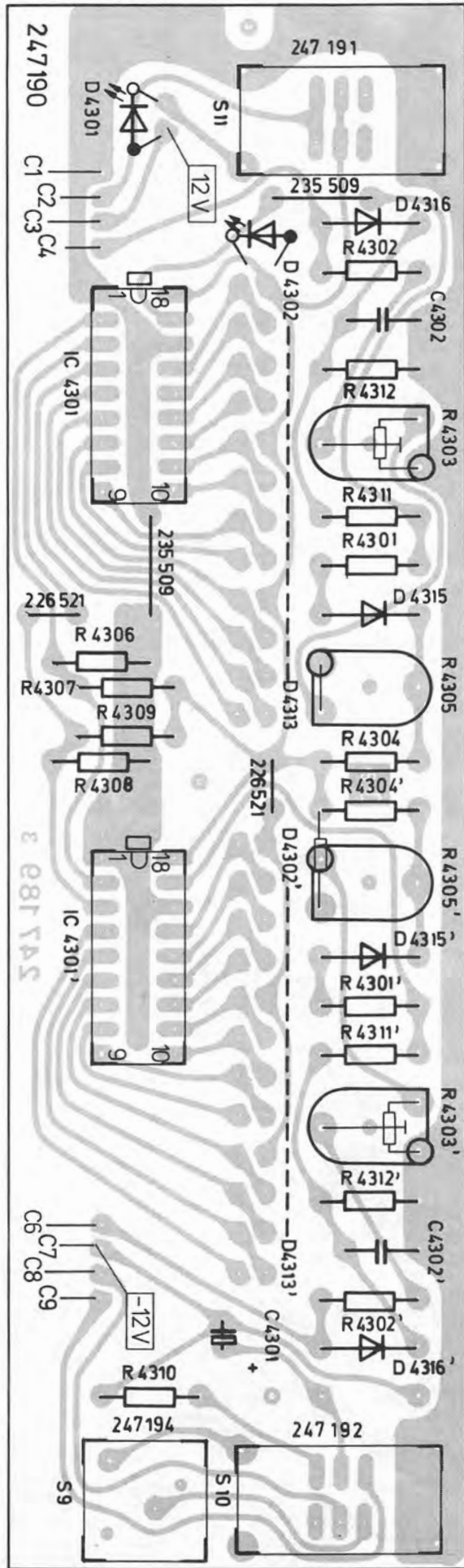
Fig. 10 LED-Anzeige 262 458 Bestückungsseite
