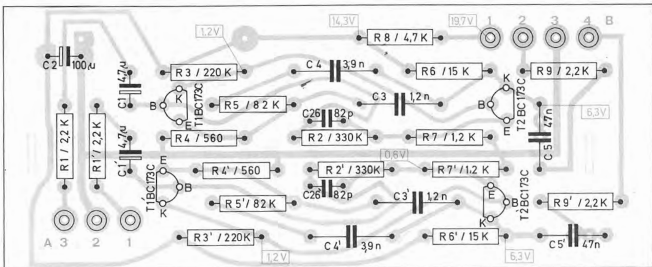
Fig. 5 Vorverstärker 227 746 (Leiterseite)
