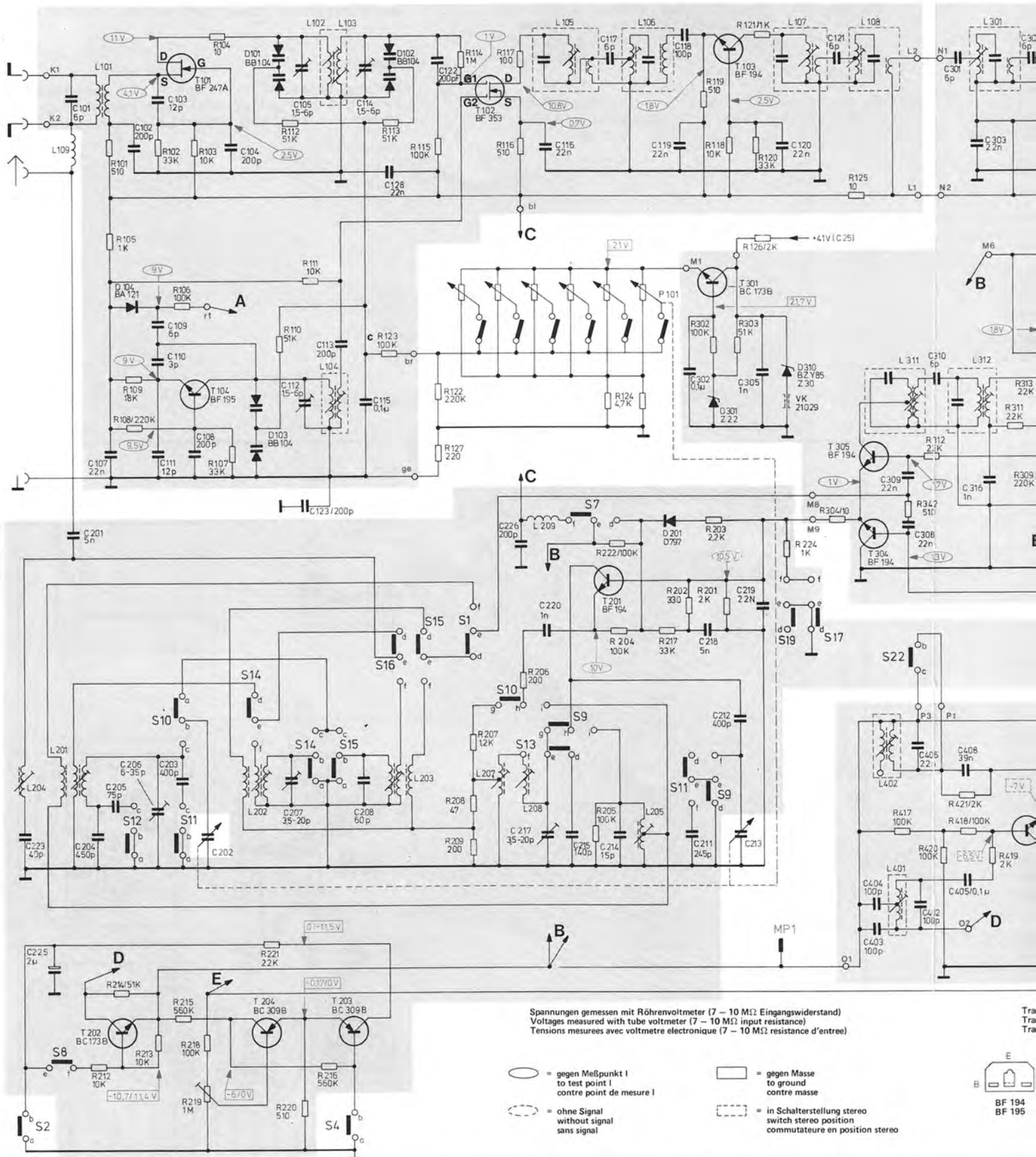
Fig. 2 Schaltbild HF
