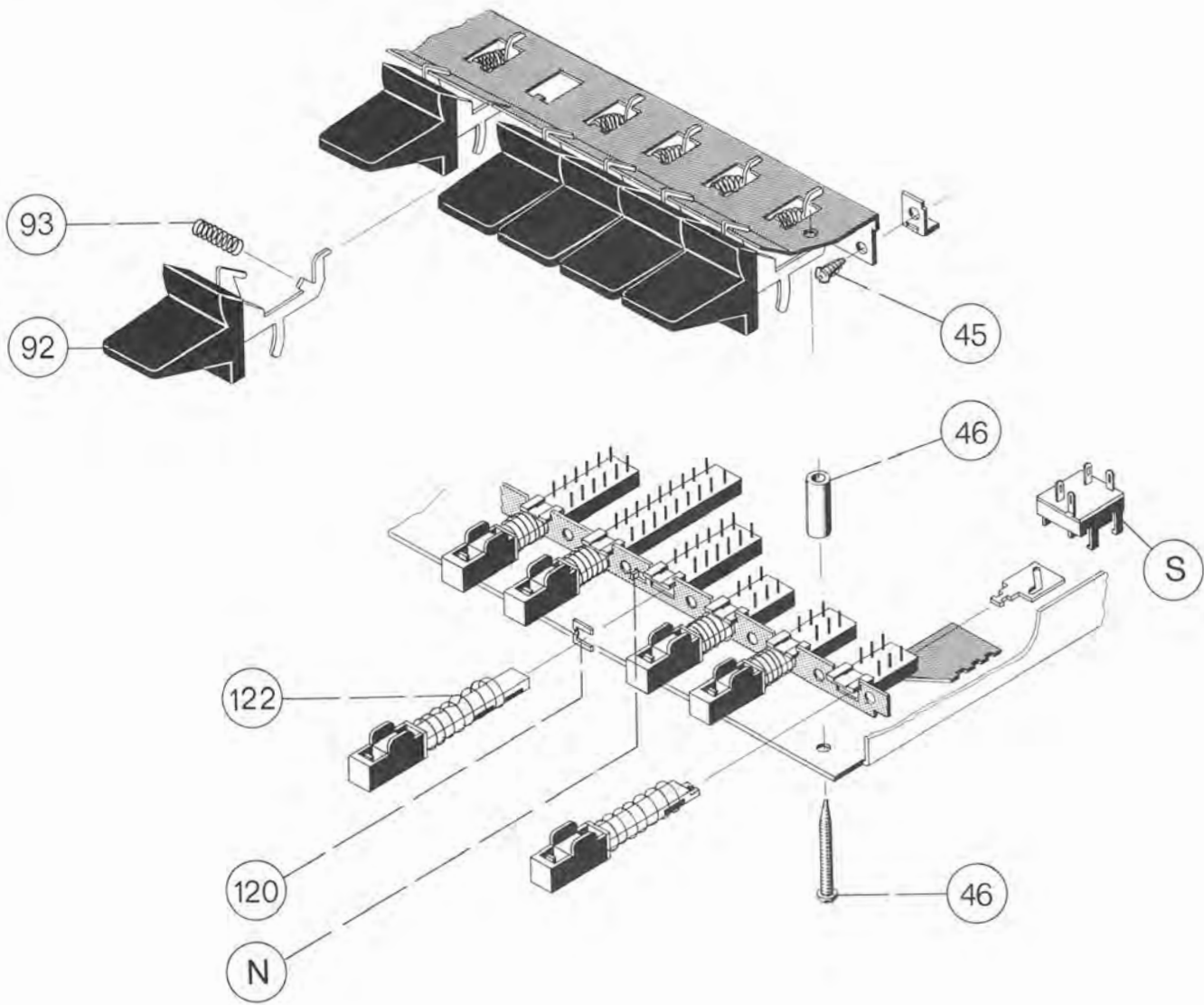
Fig. 15 Auswechseln der Tastenschieber
