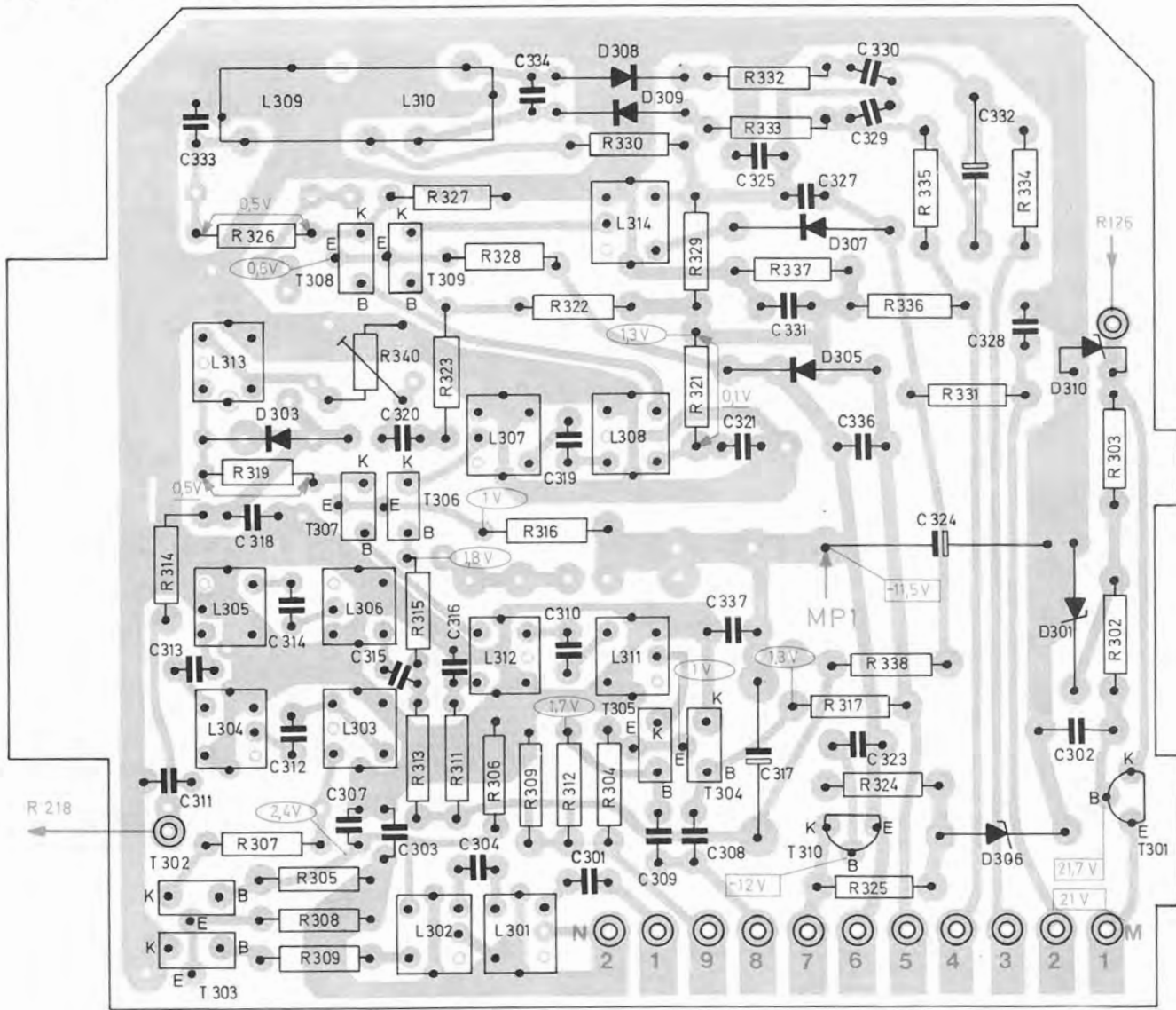
Fig. 4 ZF-Platte 231 220 (Leiterseite)
