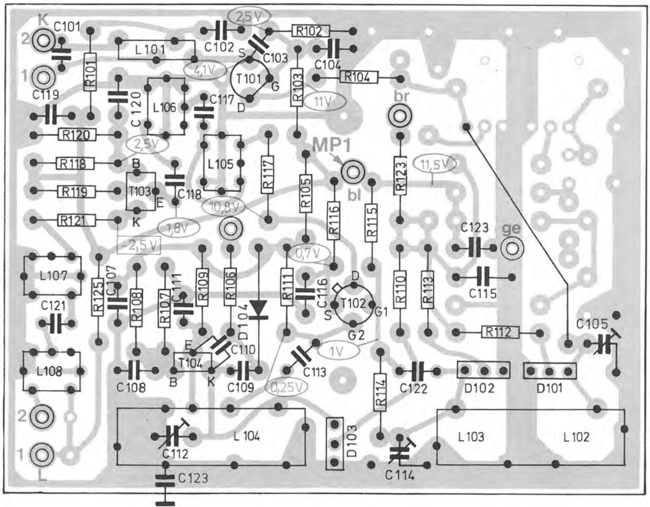
Fig. 11 UKW-Teil 231 211 (Leiterseite)
