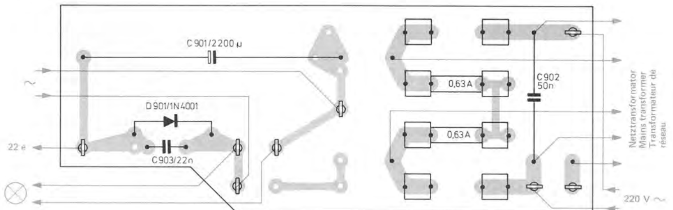
Fig. 12 Netzanschlußplatte 231 216 (Bestückungsseite)
