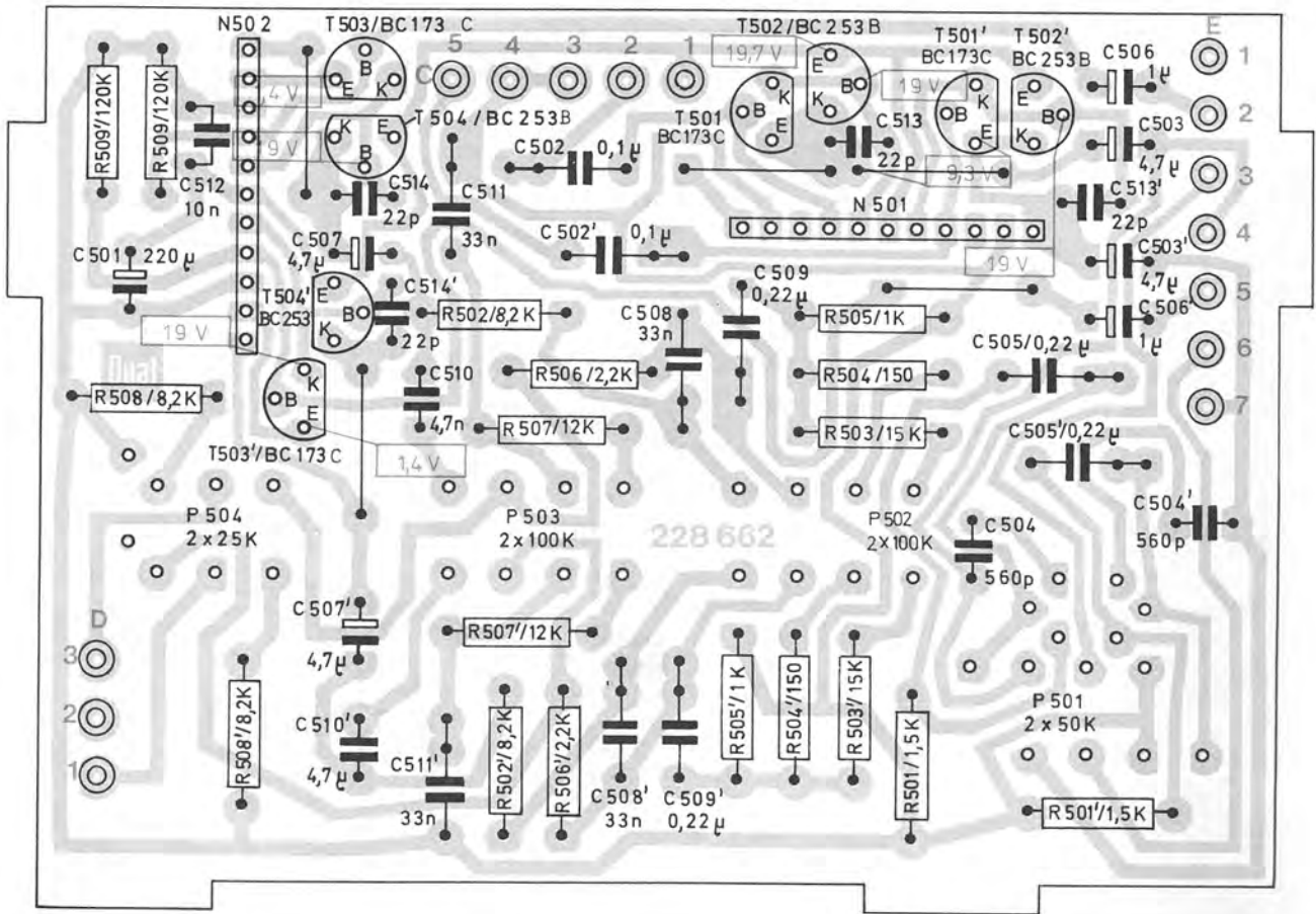
Fig. 9 Regelverstärker 230 606 (Leiterseite)
