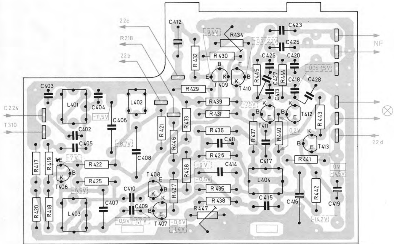
Fig. 6 Decoder 221 209 (Leiterseite)
