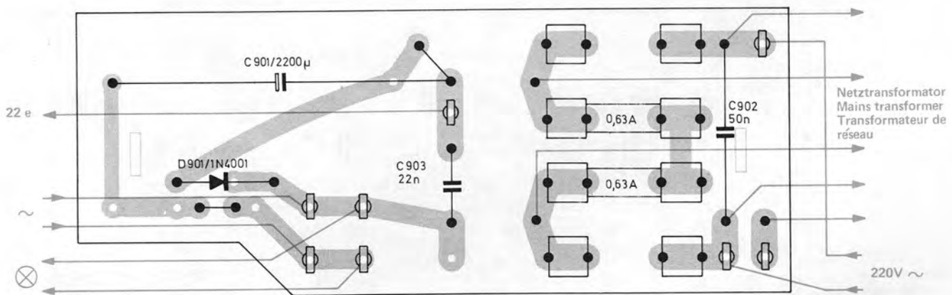
Fig. 11 Netzanschluß-Platte 231 216 (Bestückungsseite)
