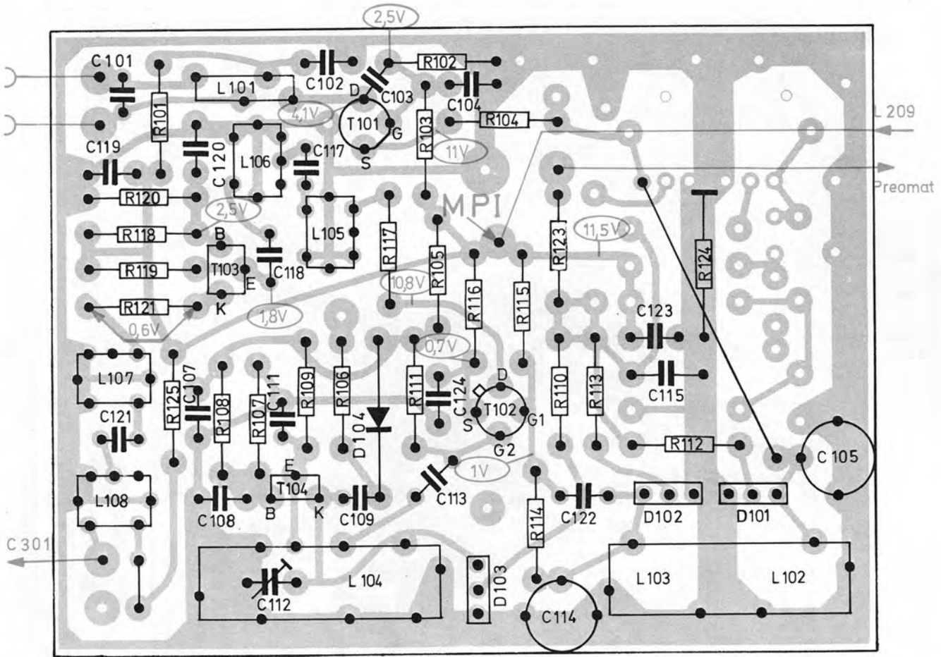
Fig. 10 UKW-Teil 231 211 (Leiterseite)
