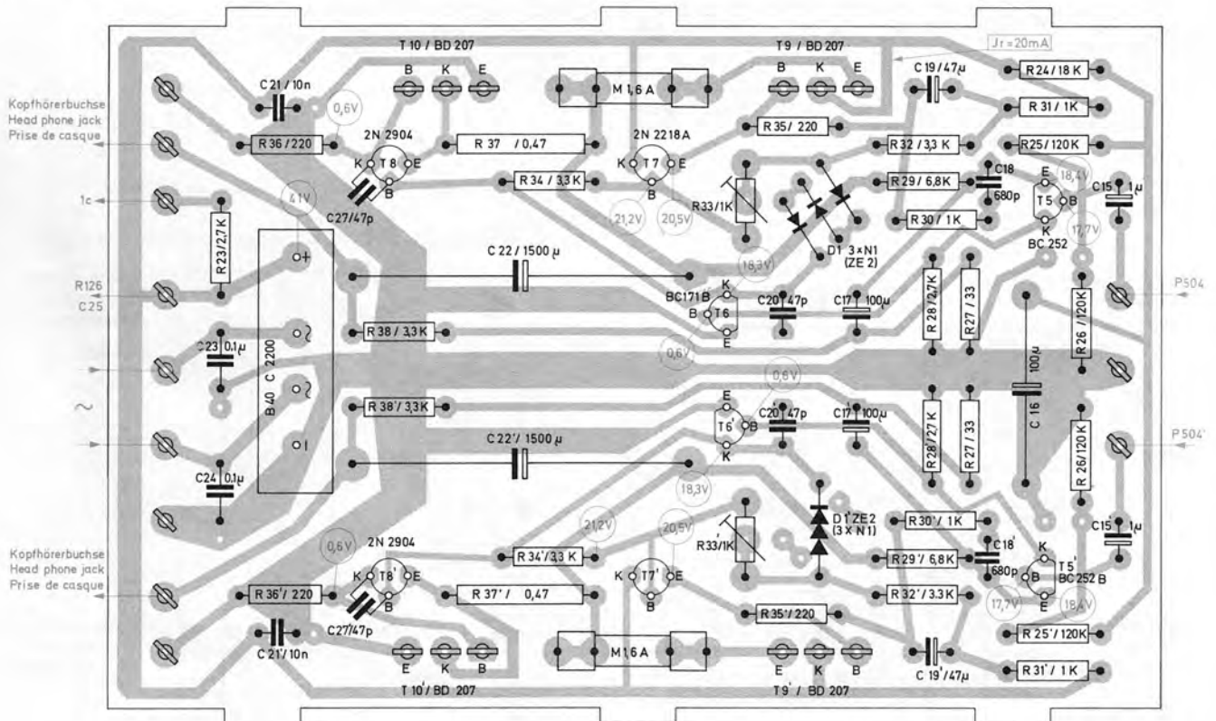
Fig. 9 Endverstärker 230 607 (Leiterseite)
