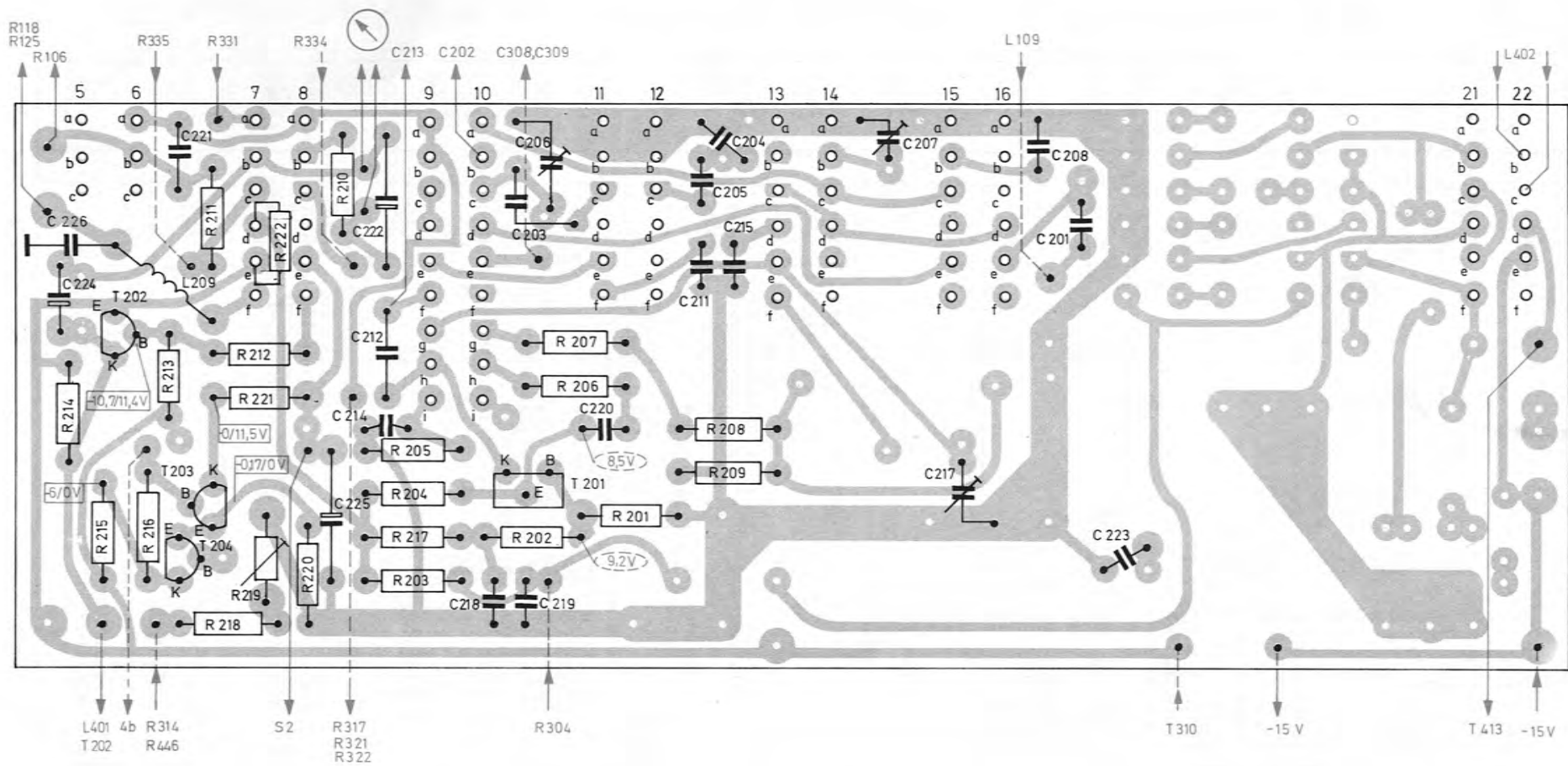
Fig. 12 AM-HF-Plate 231 206 (Leitersseite)
