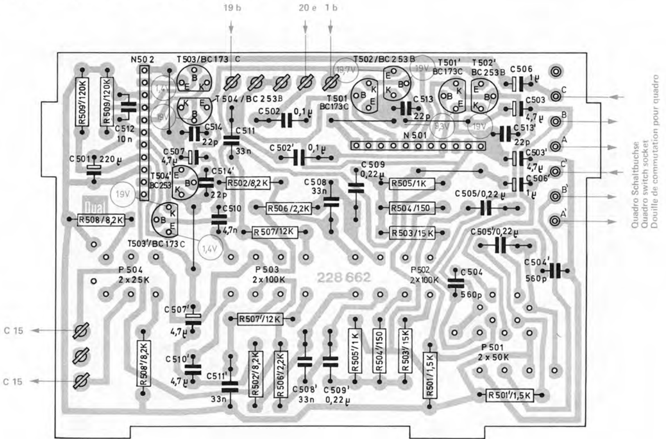
Fig. 8 Regelverstärker 230 606 (Leiterseite)
