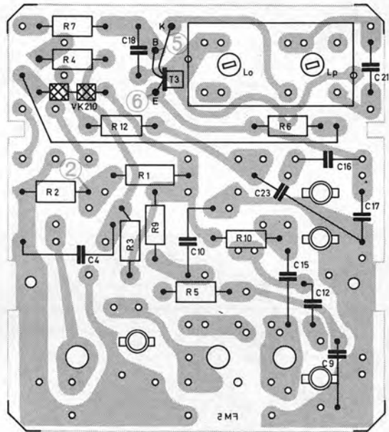
Fig. 9 UKW-Platte (Bestückungsseite)
