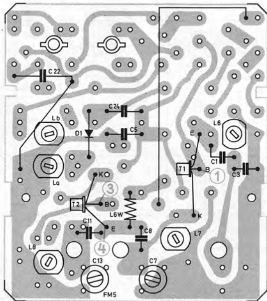
Fig. 8 UKW-Platte (Spulenseite)
