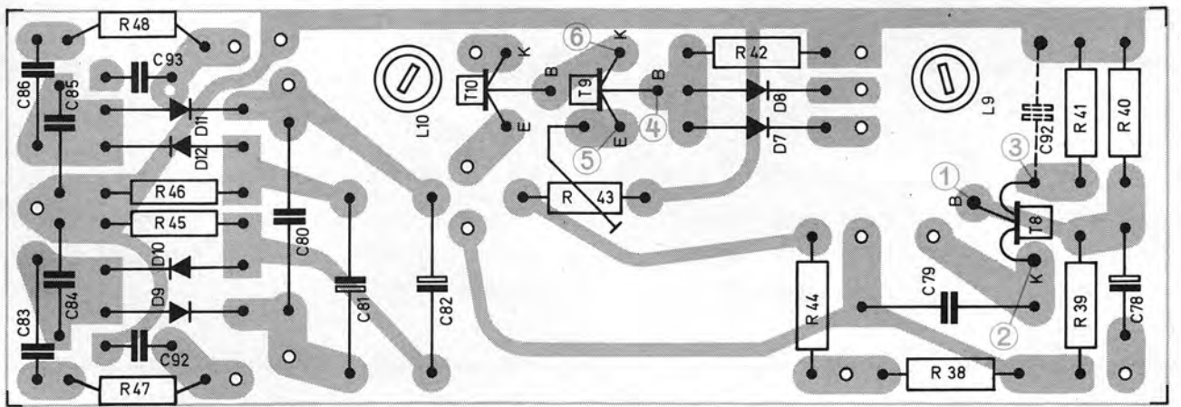
Fig. 6 Stereo-Decoder-Platte
