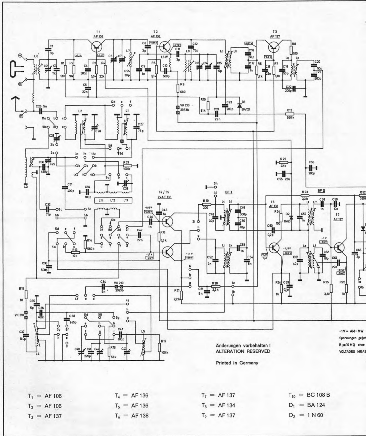
Fig. 4 Schaltplan Dual CT 12
