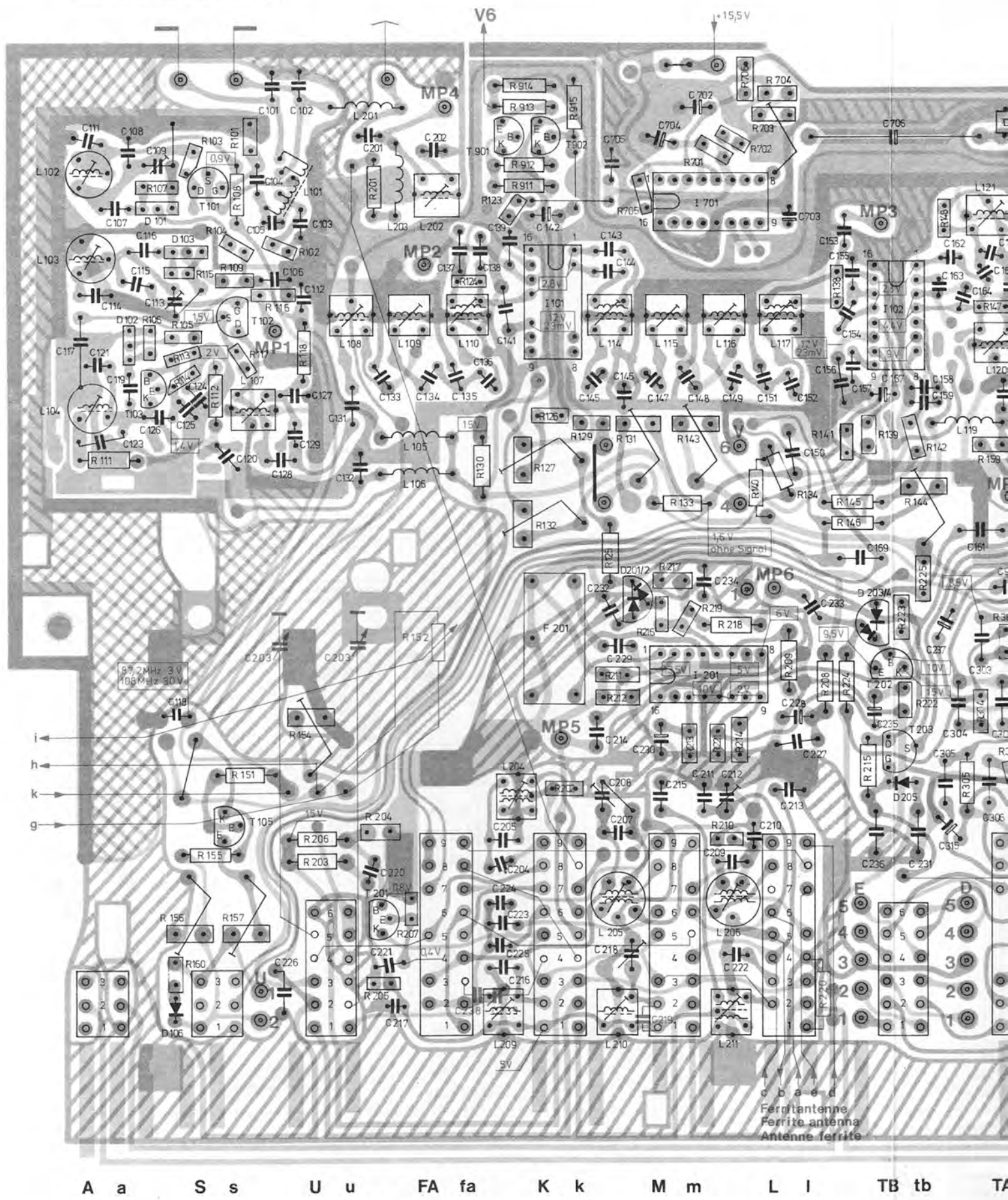
Fig. 3 HF-Teil 242 931 Leiterseite (Leiterbahnen Bestückungsseite grün)
