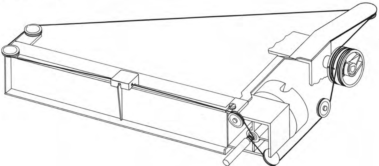
Fig. 5 Seillaufschaema
