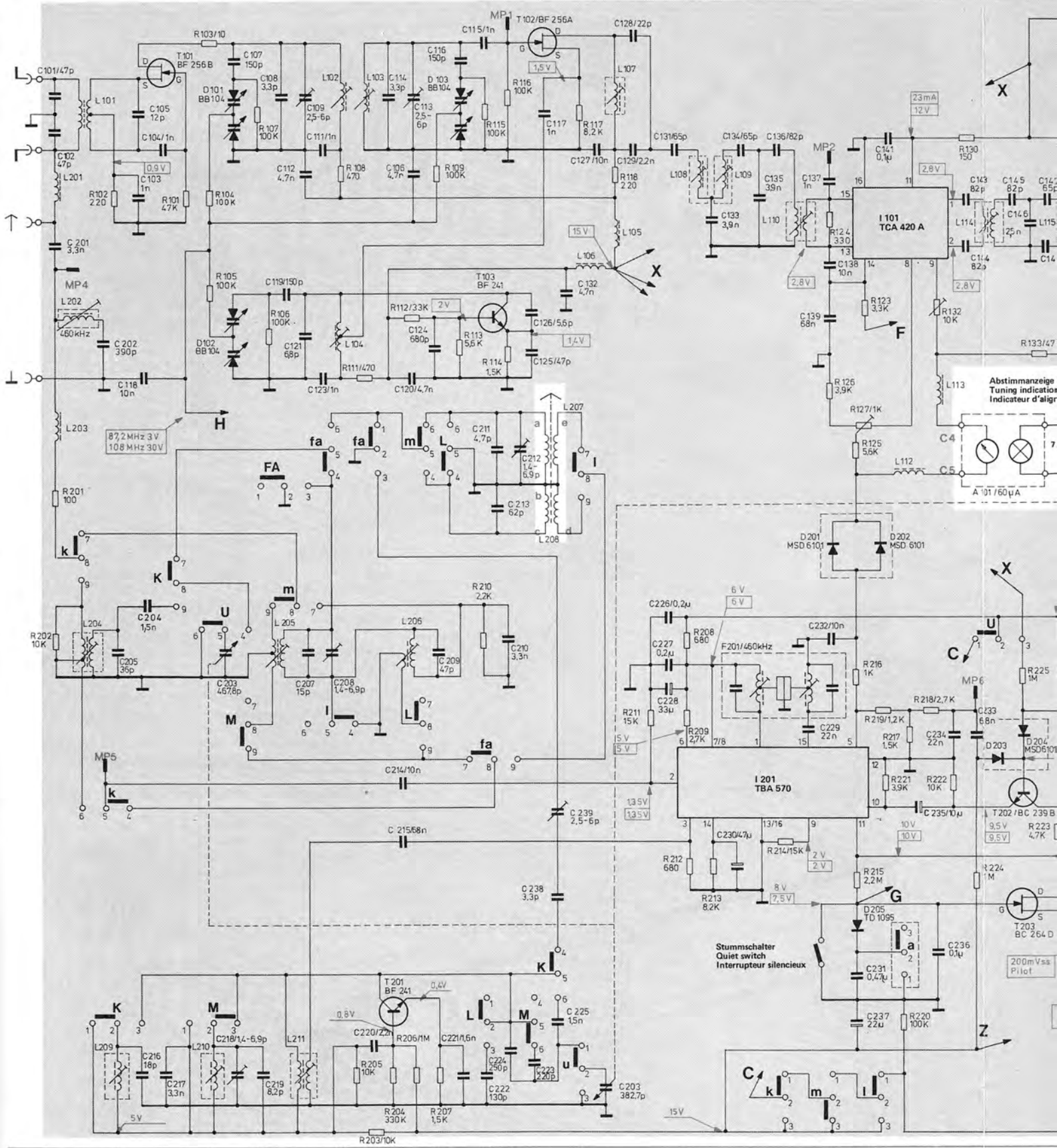
Fig. 2 Schaltbild
