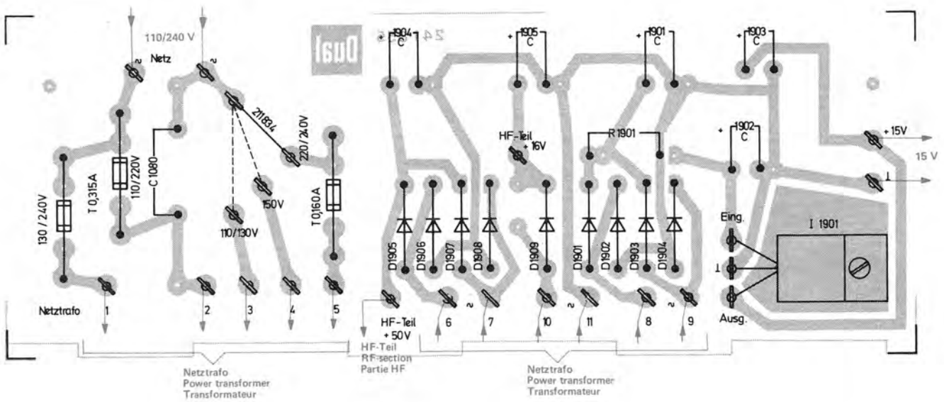
Fig. 4 Stromversorgung Bestückungsseite
