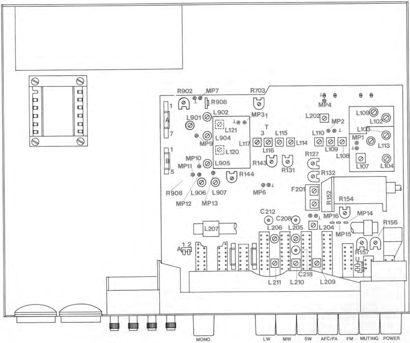
Fig. 1 Abgleichpositionen
