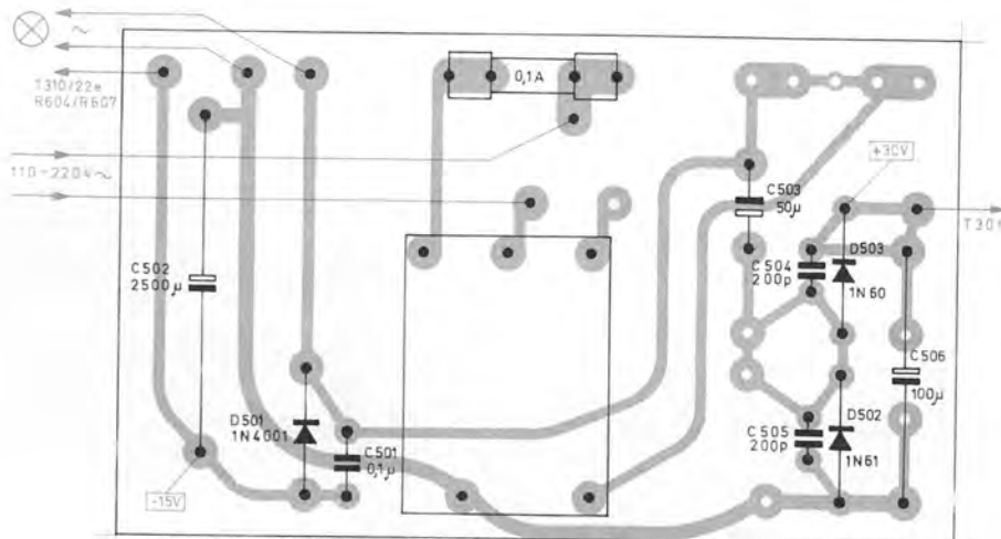
Fig. 8 Netzteil 231 203 (Bestückungsseite)
