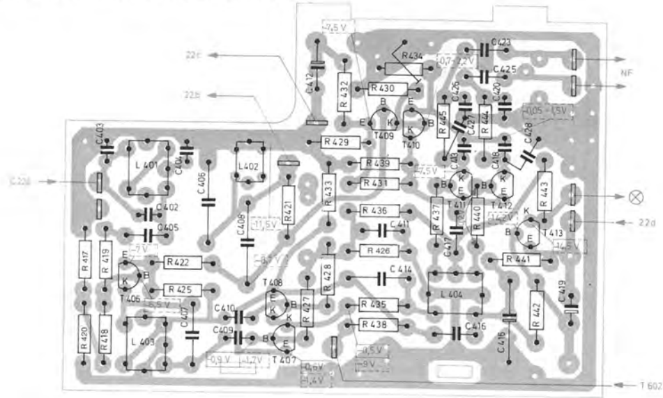
Fig. 7 Stereo-Decoder 231 210 (Leiterseite)
