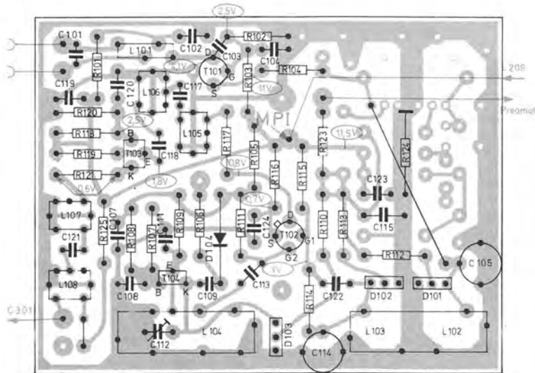
Fig. 3 UKW-Teil 231 211 (Leiterseite)
