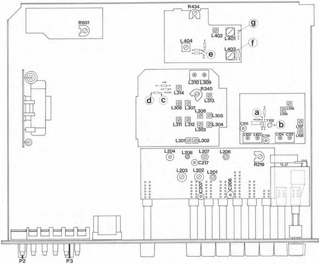
Fig. 1 Abgleichpositionen
