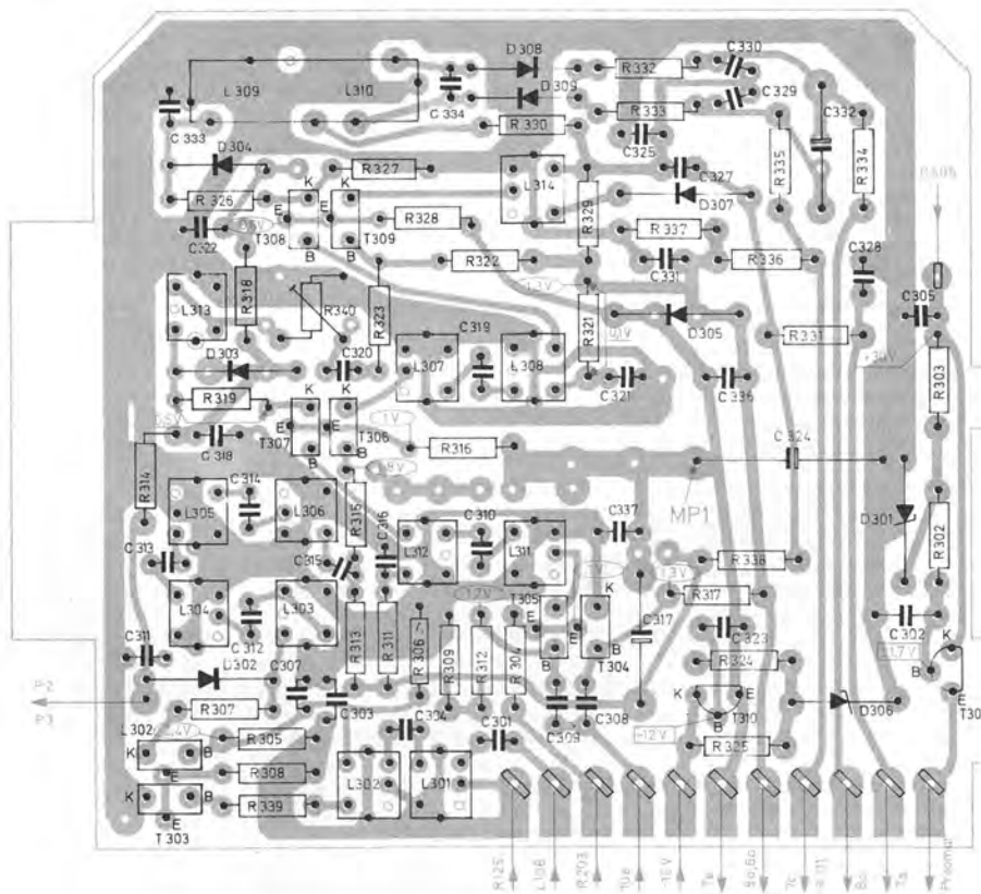
Fig. 5 Flip-Flop 231 213 (Bestückungsseite)
