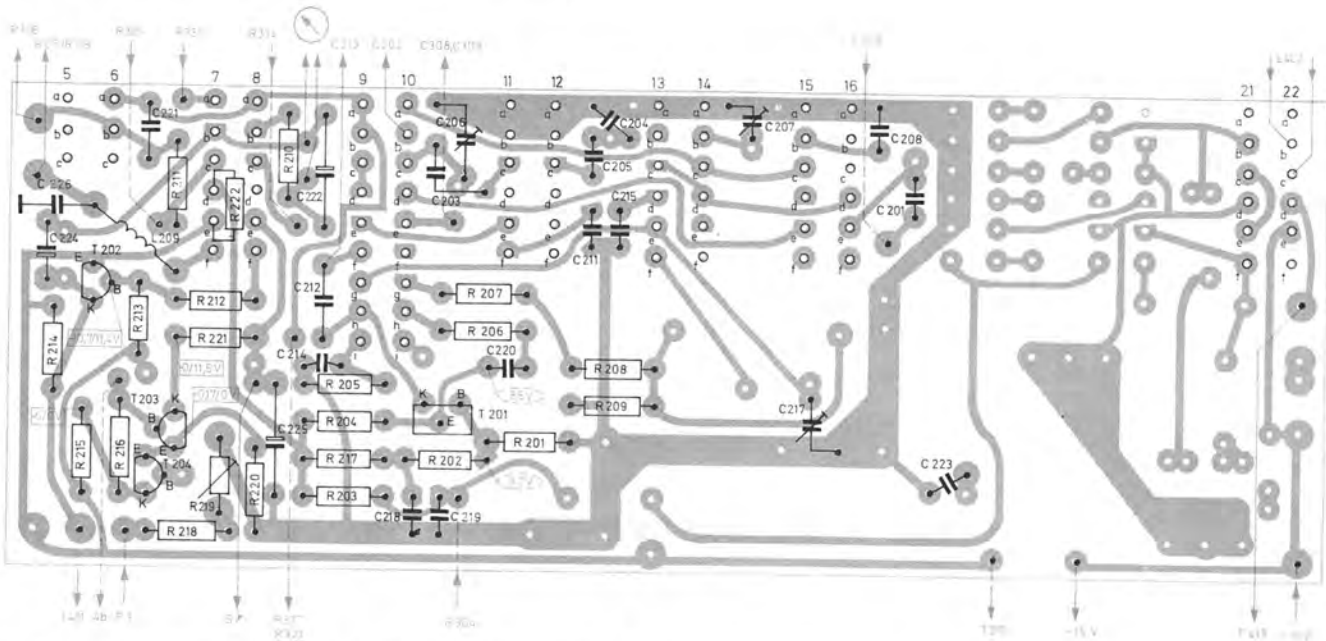
Fig. 7 Stereo-Decoder 231 210 (Leiterseite)
