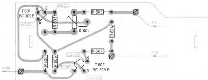
Fig. 5 Flip-Flop 231 213 (Bestückungsseite)
