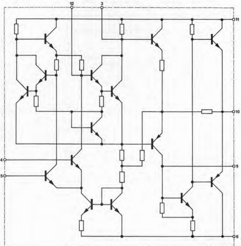
Fig. 4 Prinzipschaltbild, Operationsverstärker
