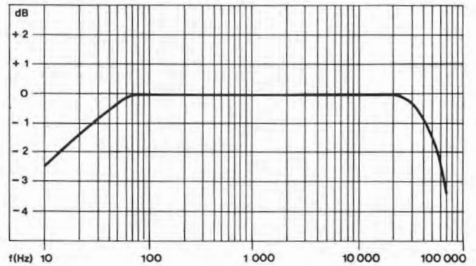
Fig. 6 Leistungsbandbreite nach DIN 45 500 8 Hz bis 55 000 Hz
