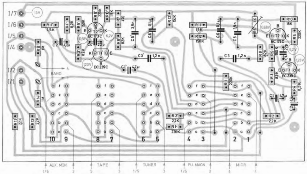
Fig. 12 Anschlußplatte 229 090 (Bestückungsseite)
