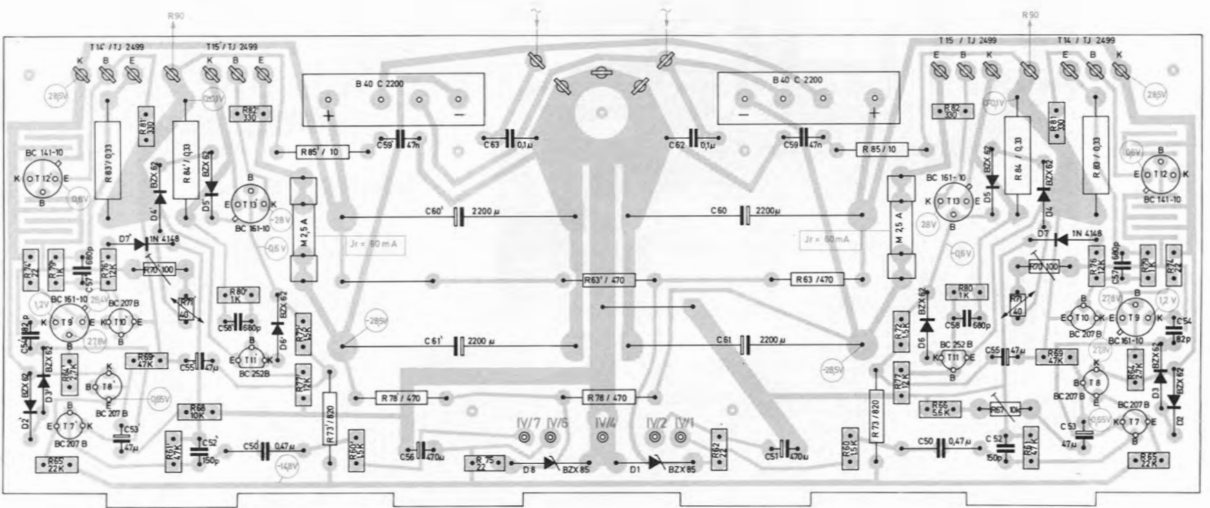
Fig. 17 Endverstärker 229 093 (Leitenseite)
