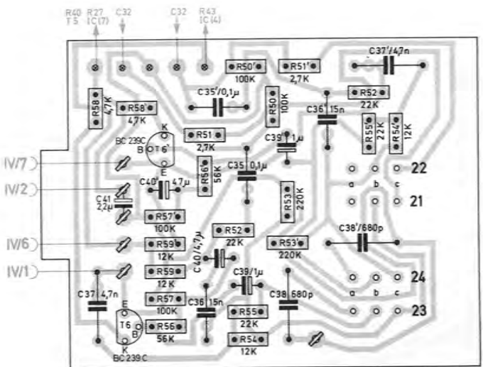
Fig. 16 Filterplatte 229 094 (Leiterseite)
