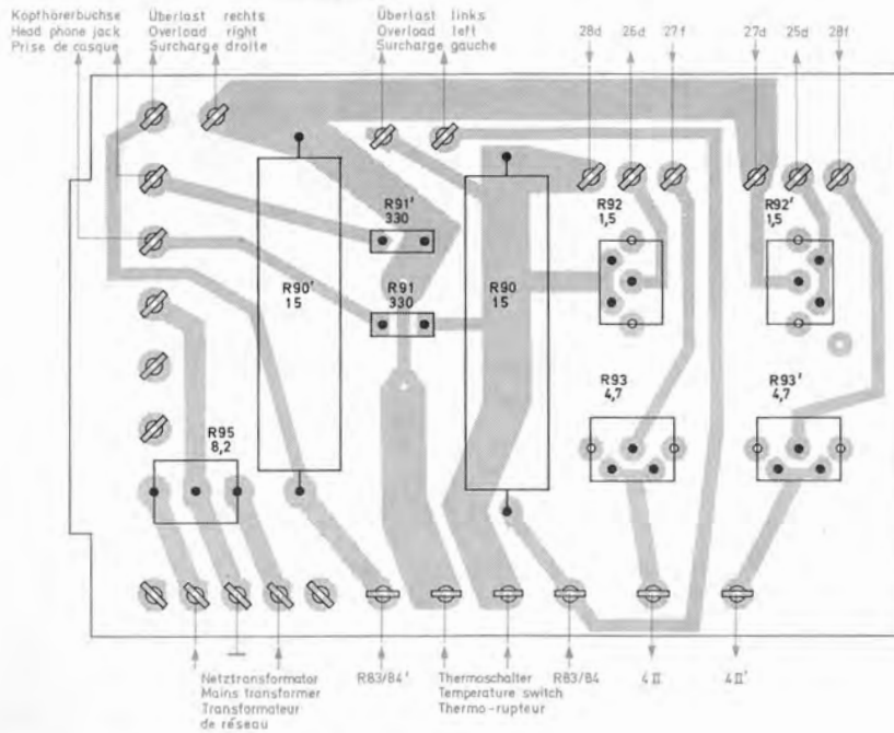
Fig. 13 Trafoanschlußplatte 223 814 (Bestückungsseite)
