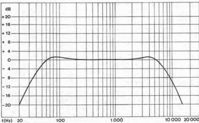
Fig. 9 Wirkungsweise der Rumpel- und Rauschfilter
