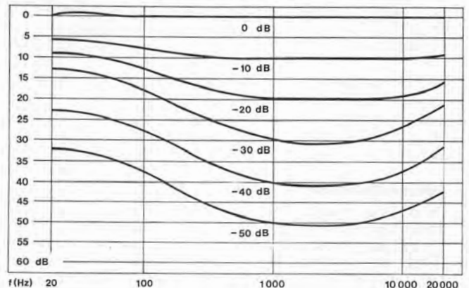
Fig. 10 Wirkungsweise der physiologischen Lautstärkeregelung. 0 dB = Lautstärkereglter offen
