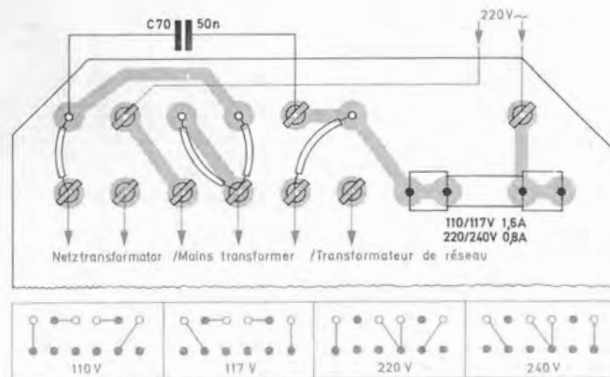
Fig. 13 Trafoanschlußplatte 223 814 (Bestückungsseite)
