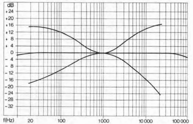
Fig. 10 Wirkungsweise der physiologischen Lautstärkeregelung. 0 dB = Lautstärkereglter offen
