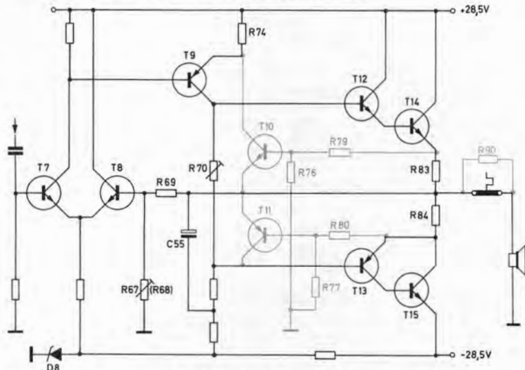
Fig. 4 Prinzipschaltbild, Operationsverstärker
