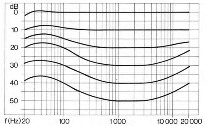
Fig. 9 Wirkungsweise der physiologischen Lautstärkeregelung. 0 dB = Lautstärkeregelung offen
