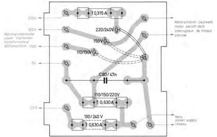
Fig. 3 Ätzsaltplatte der Stromversorgung 224 974 (Leiterseite)
