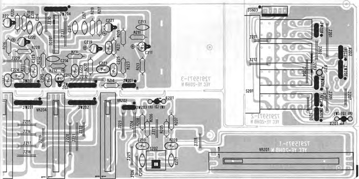
Platte / Control board / Plaque de Contrôle B
