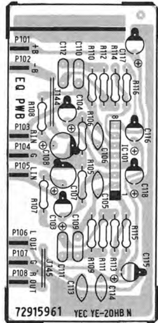
EQ-platte / EQ board / Plaque de EQ B
