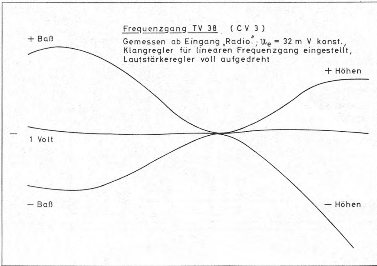
Fig. 13 Frequenzgänge
