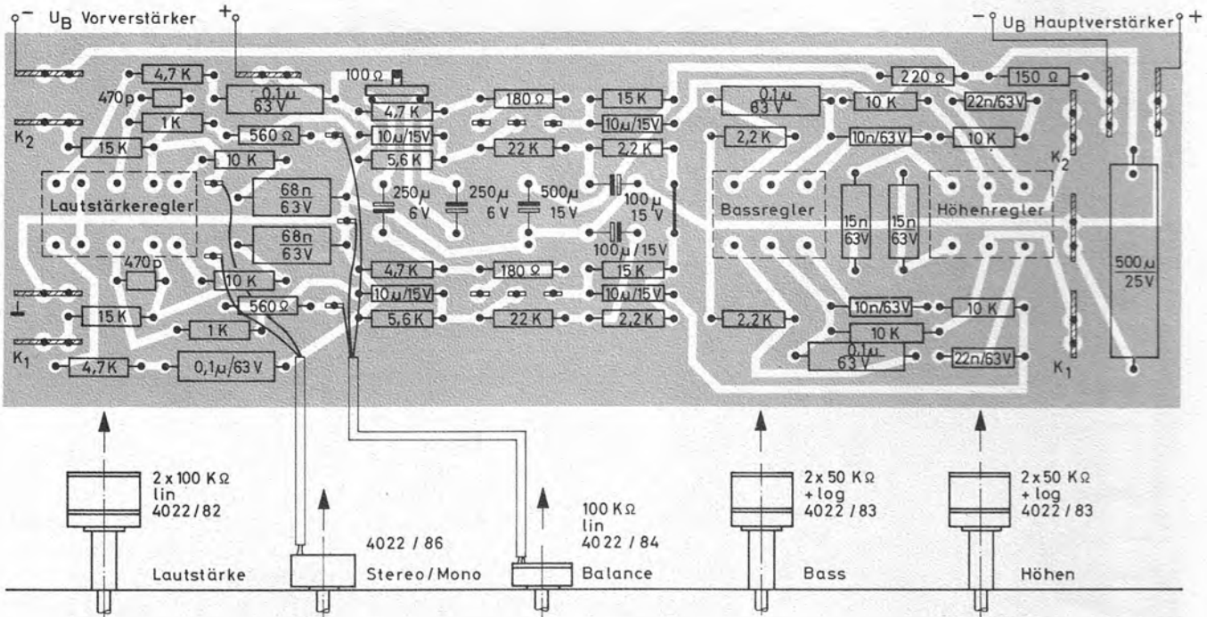
Fig. 10 Regelverstärker Ätzschriftplatte 36 J - U 63
