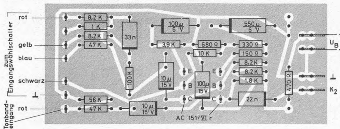
Fig. 8 Entzerrer-Vorverstärker Ät Schaltplatte unten 36 J - U 84 (linker Kanal)
