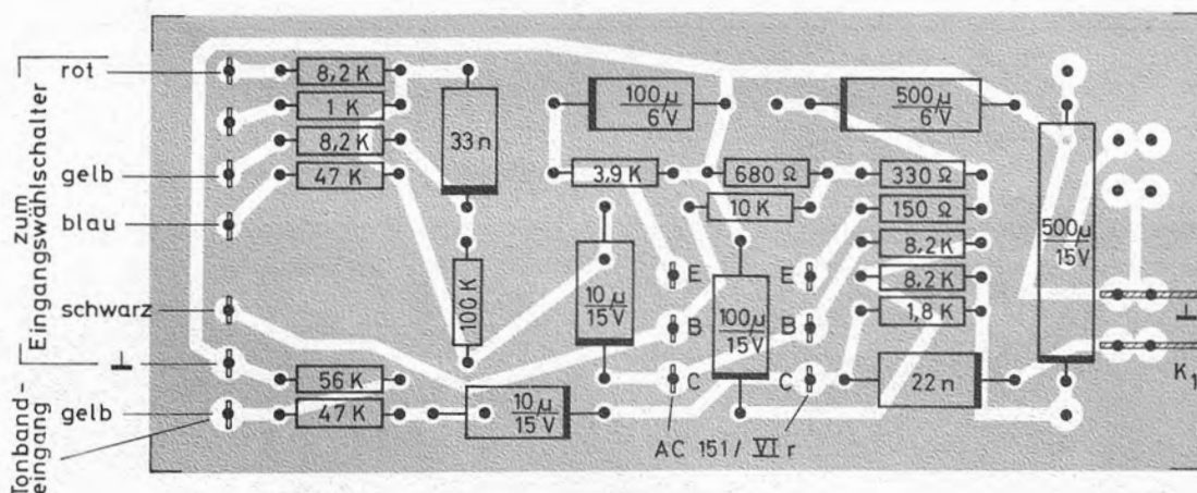
Fig. 7 Entzerrer-Vorverstärker Ät Schaltplatte oben 36 J - U 86 (rechter Kanal = K_1 )
