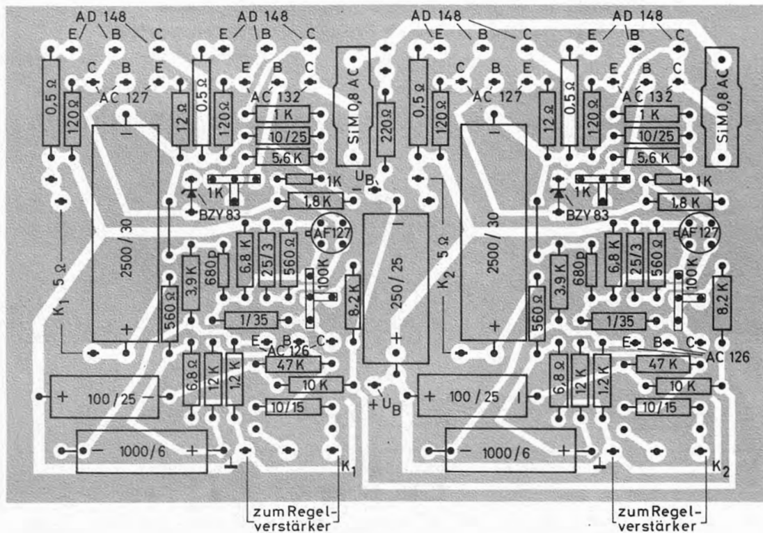
Fig. 12 Hauptverstärker (Endstufe) Ätzschatplatte 36 J - U 42
