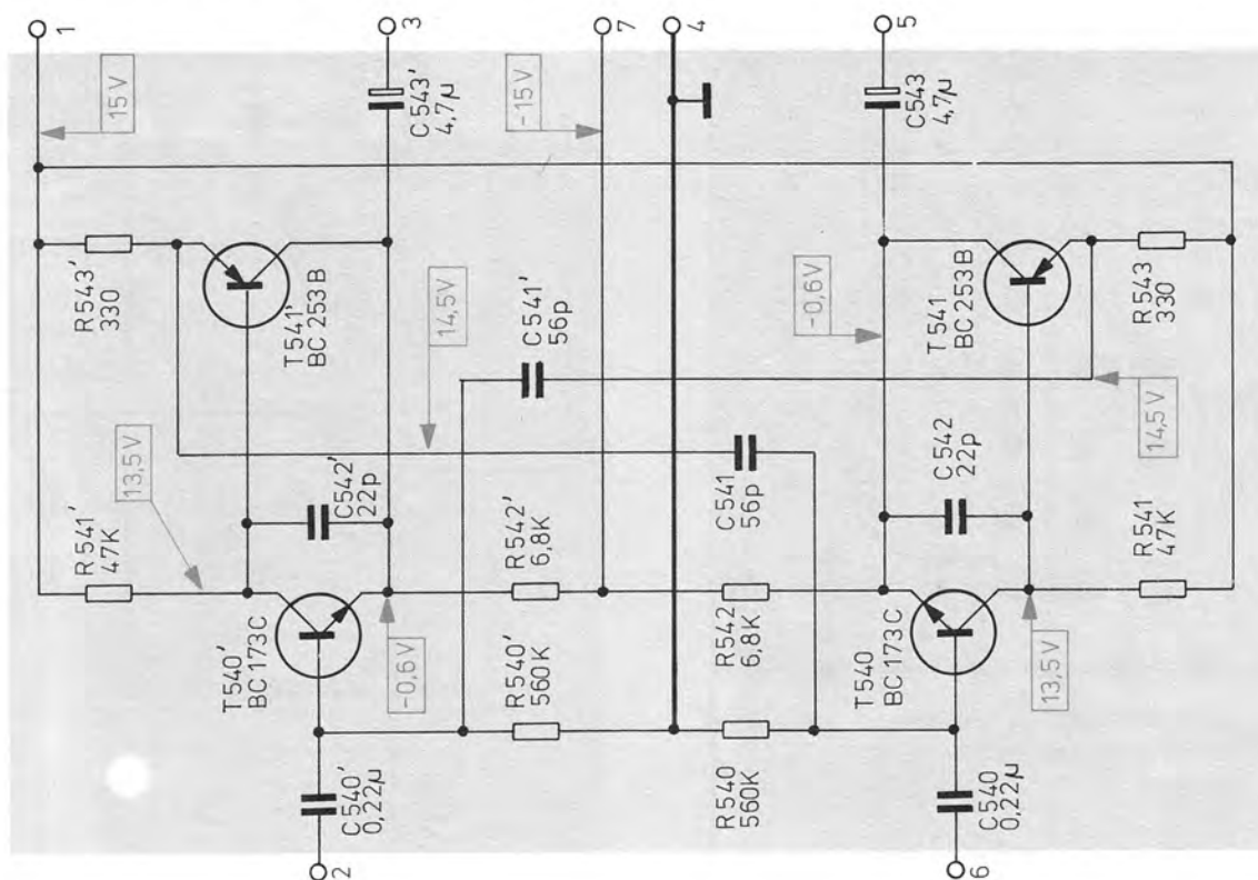
Fig. 16 Impedanzwandler III Schaltbild
