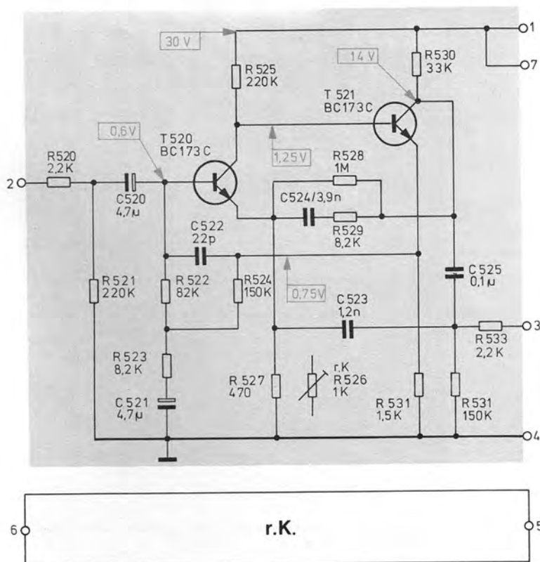
Fig. 17 Vorverstärker II Schaltbild
