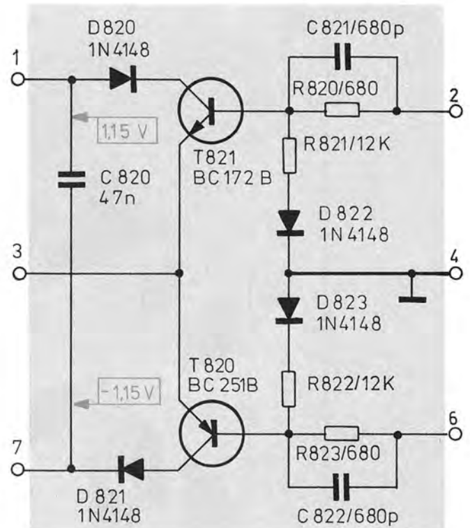
Fig. 24 Elektronische Sicherung VI Schaltbild
