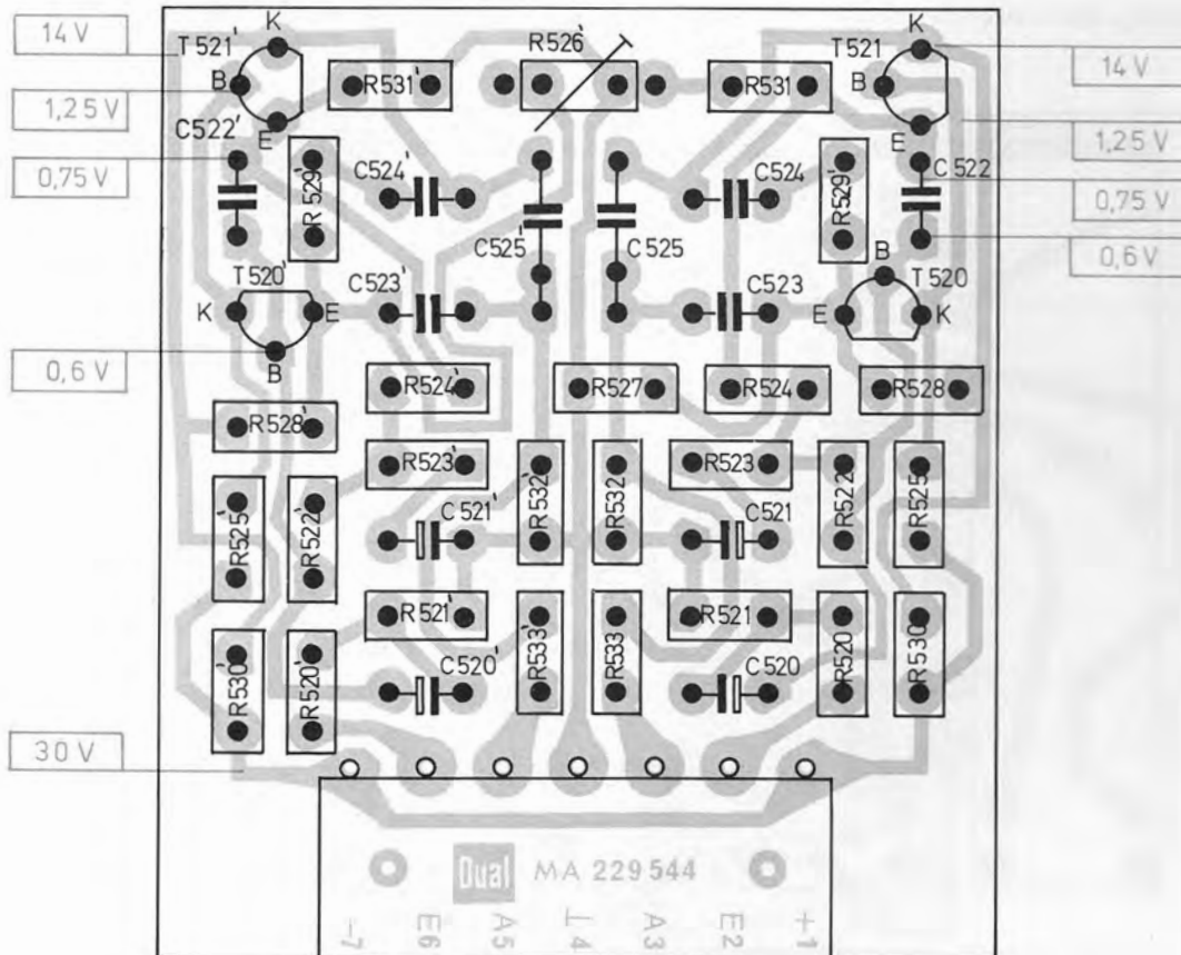
Fig. 15 Vorverstärker II 232 464 (Leiterseite)
