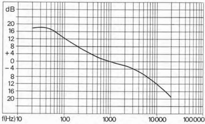
Fig. 1 Frequenzgang des Vorverstärkers Magneiteingang
