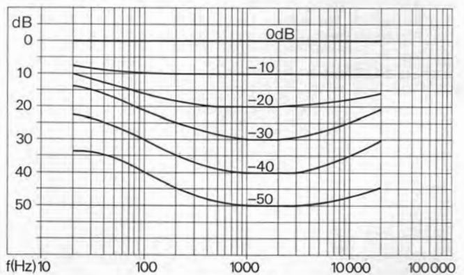
Fig. 6 Wirkungsweise der physiologischen Lautstärkeregelung 0 dB = Lautstärkereglern offen
