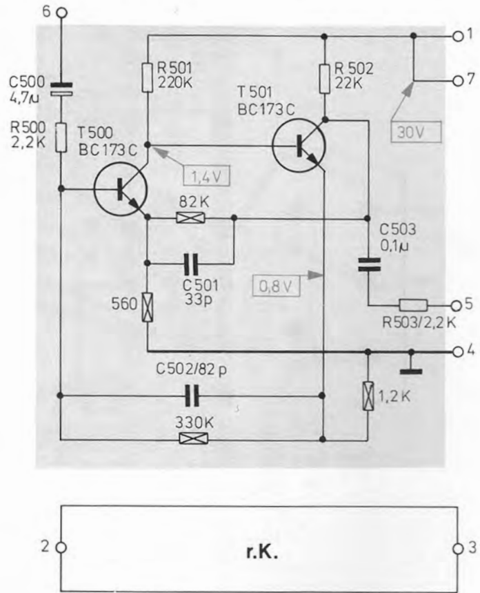
Fig. 14 Mikro-Vorverstärker I Schaltbild
