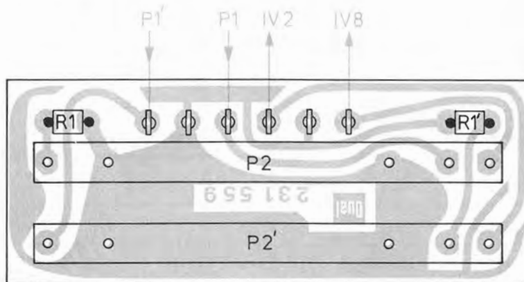
Fig. 9 Balancereglerplatte 233 989 (Leiterseite)
