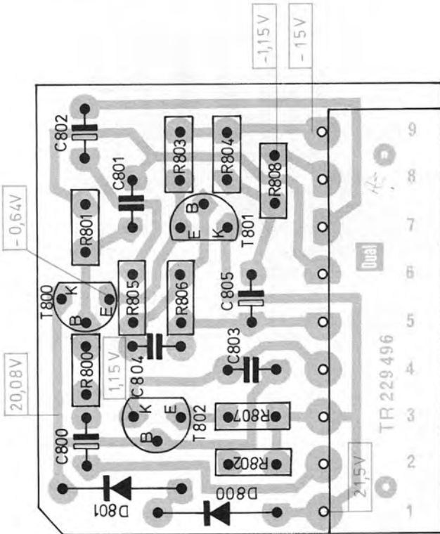
Fig. 21 Universaltreiber V 232 452 (Leiterseite)
