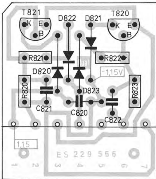
Fig. 23 Elektronische Sicherung VI 232 451 (Leiterseite)
