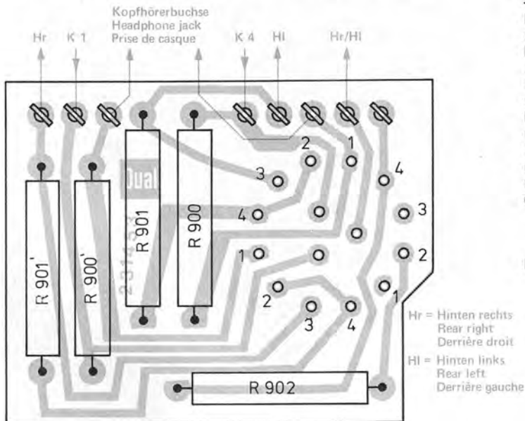
Fig. 25 Modeschalter 233 975 (Leiterseite)
