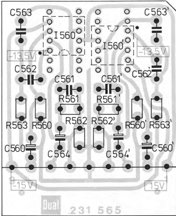
Fig. 19 Zwischenverstärker IV 233 991 (Leiterseite)
