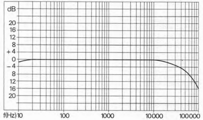
Fig. 2 Frequenzgang des Mikro-Vor- verstärkers
