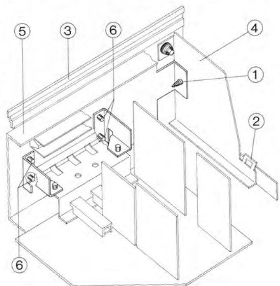
Fig. 26 Ausbau des Steuerverstärkers
