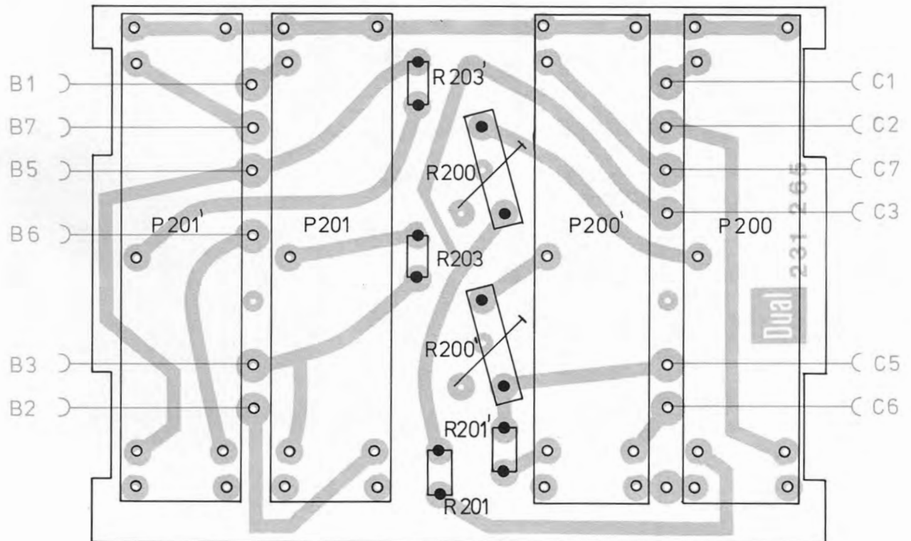
Fig. 12 Klangreglerplatte 233 987 (Leiterseite)
