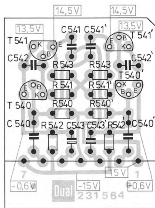
Fig. 18 Impedanzwandler III 233 985 (Leiterseite)
