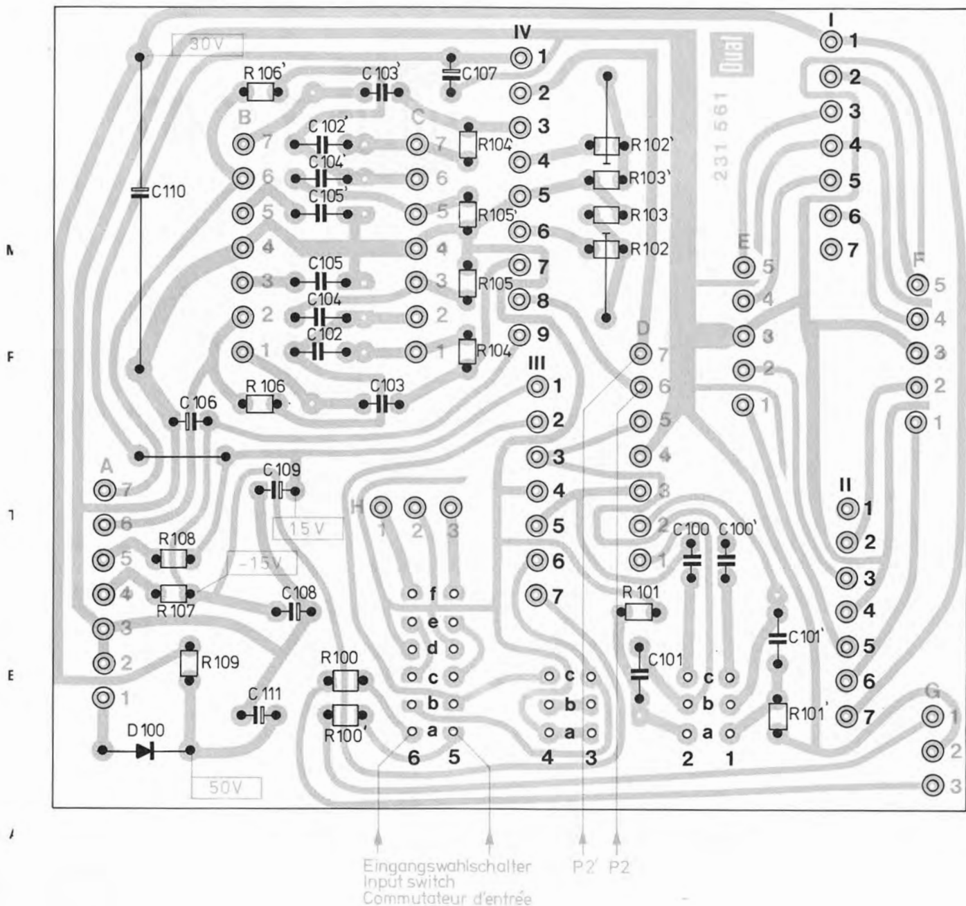
I Fig. 8 Steuerverstärker 233 988 (Leiterseite)
