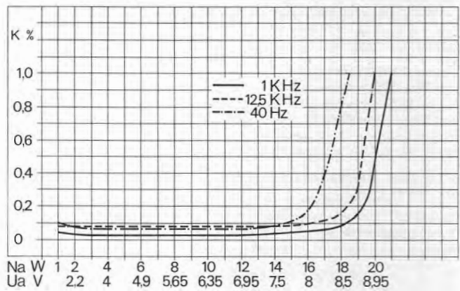
Fig. 4 Klirrrgrad bei 40 Hz, 1 kHz, 12,5 kHz in Abhängigkeit von der Ausgangslei- stung
