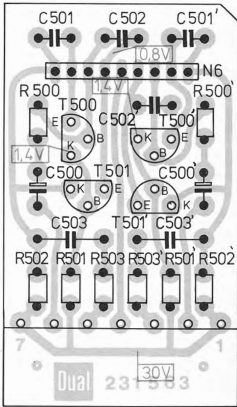
Fig. 13 Mikro-Vorverstärker I 233 992 (Leiterseite)
