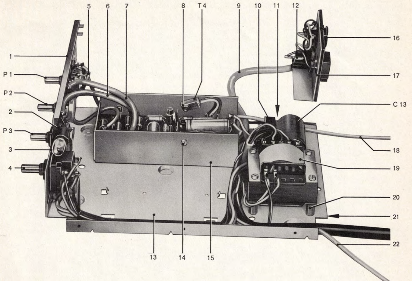
Fig. 2 Transistor-Verstärker TV 54 kpl.
