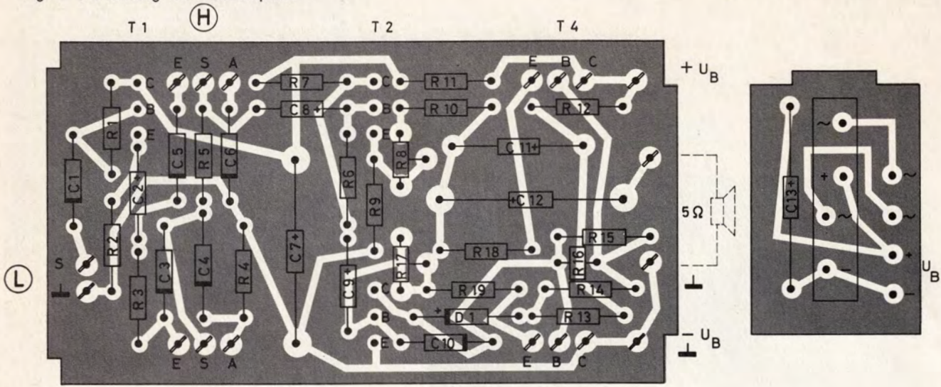
Fig. 3 Bestückung der Ätzschtaltplatte
